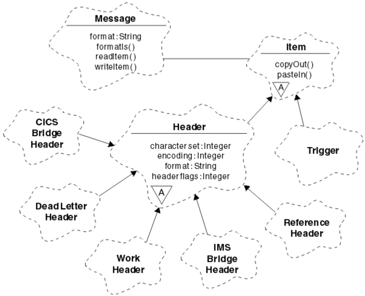
Şekil 58. IBM MQ C++ sınıfları (öğe işleme)
