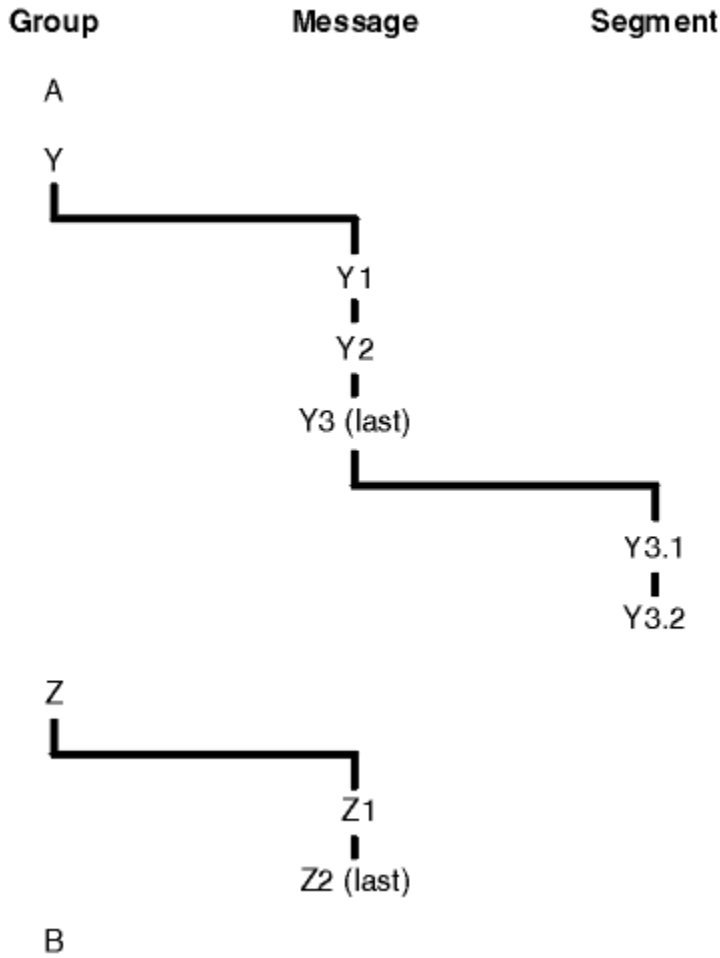
Şekil 66. Kuyruğun mantıksal sırası
