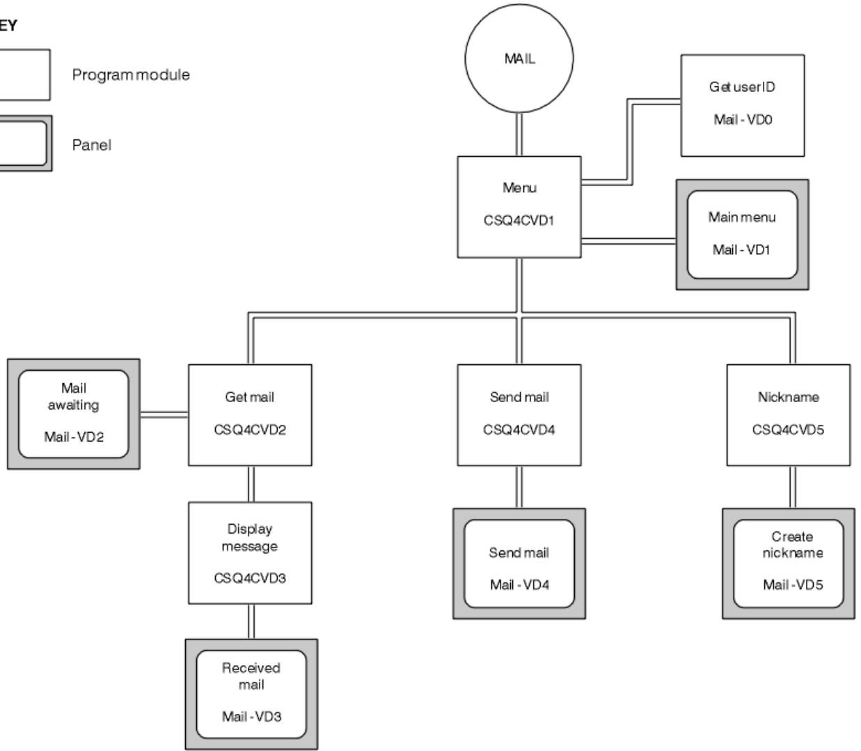
Şekil 148. Posta Yöneticisi 'nin CICS sürümüne ilişkin programlar ve panolar
