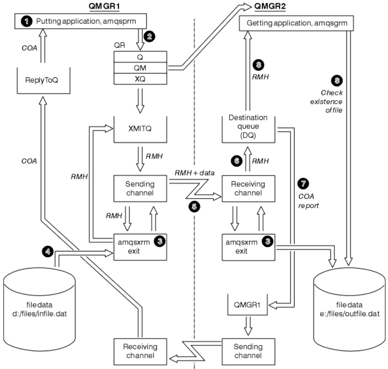
Şekil 138. Başvuru İletisi örneklerinin çalıştırılması
