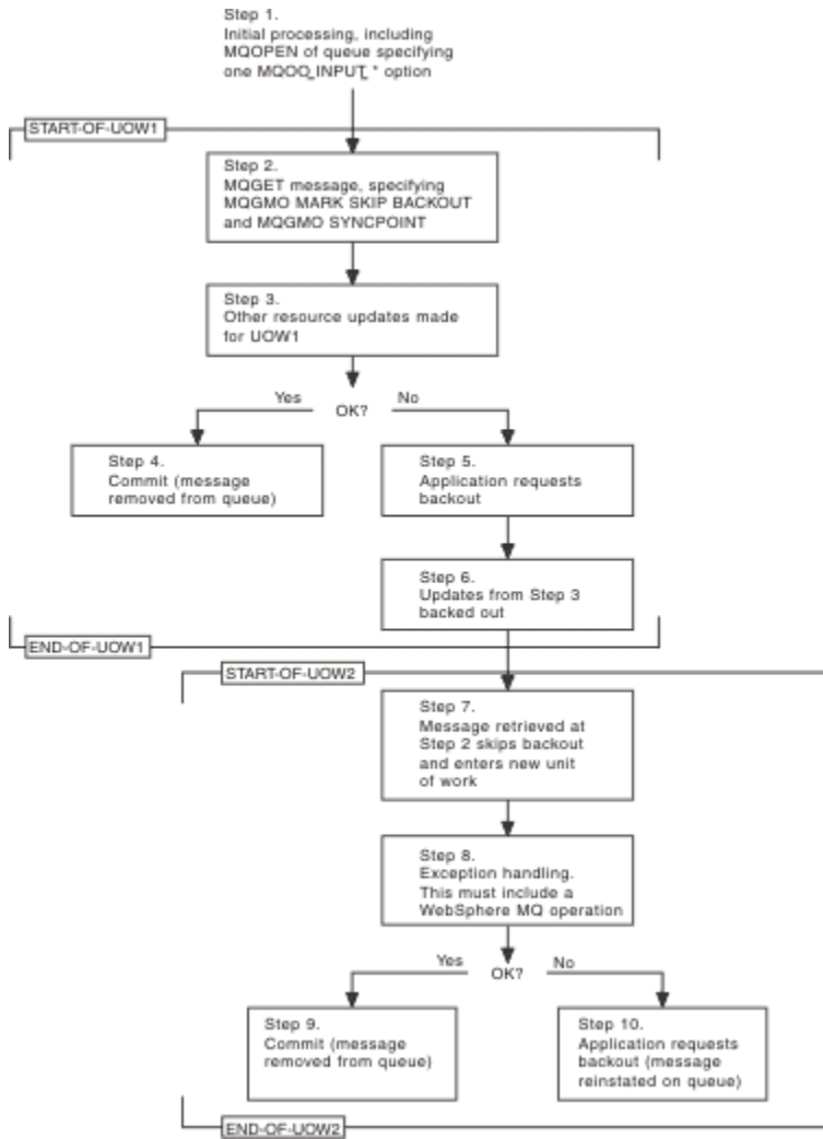
Şekil 68. MQGMO_MARK_SKIP_BACKOUT kullanılarak geriiletme atlanıyor
