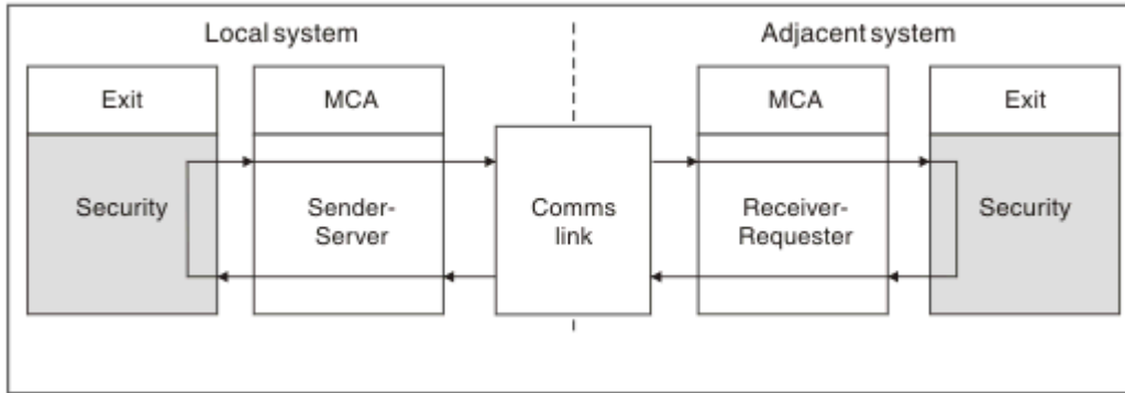
Şekil 110. Güvenlik çıkış döngüsü
