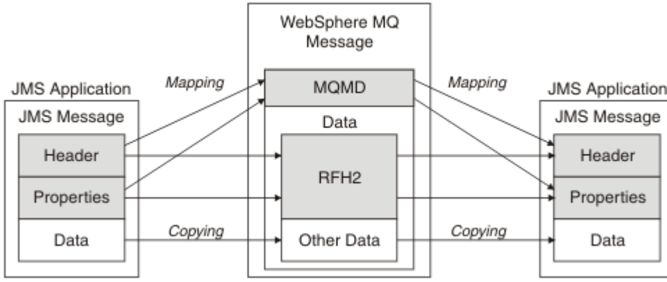
Şekil 12. İletilerin MQRFH2 üstbilgisi kullanılarak JMS ile IBM MQ arasında nasıl dönüştürülebileceğini
