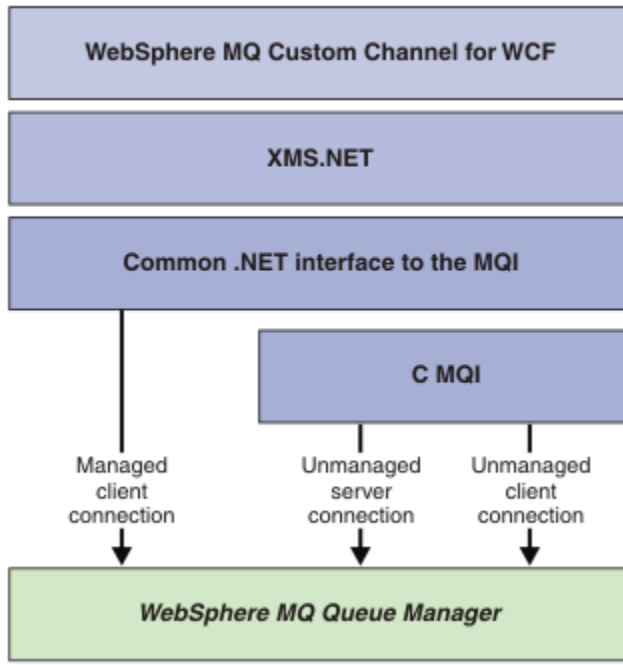
Şekil 156. SOAP/JMS arabirimi için WCF mimarisi
