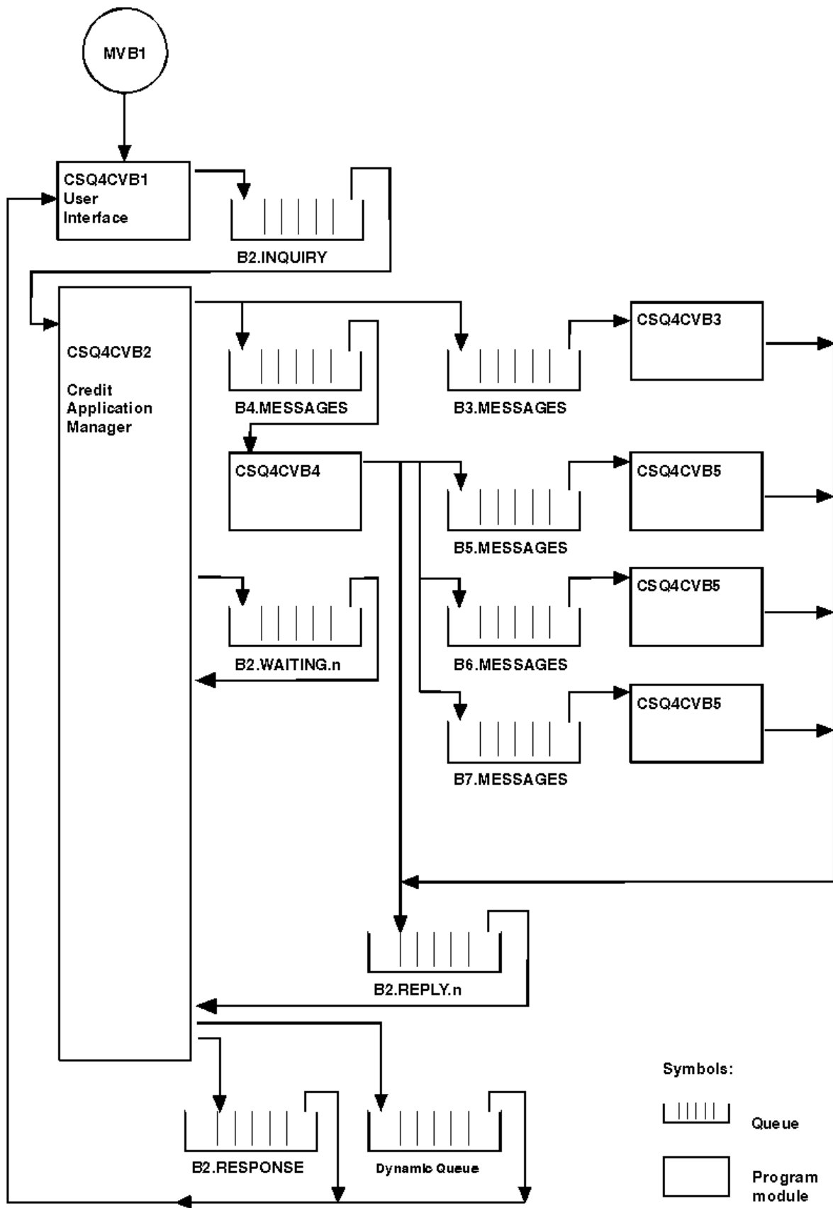
Şekil 152. Credit Check örnek uygulamasına ilişkin programlar ve kuyruklar (yalnızca COBOL programları)
