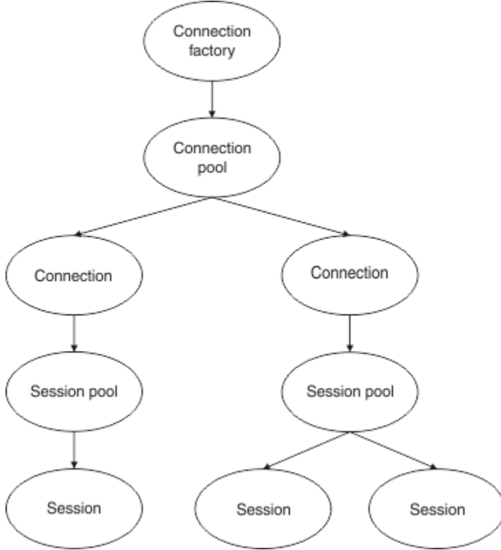
Şekil 10. Bağlantı havuzları ve oturum havuzları
