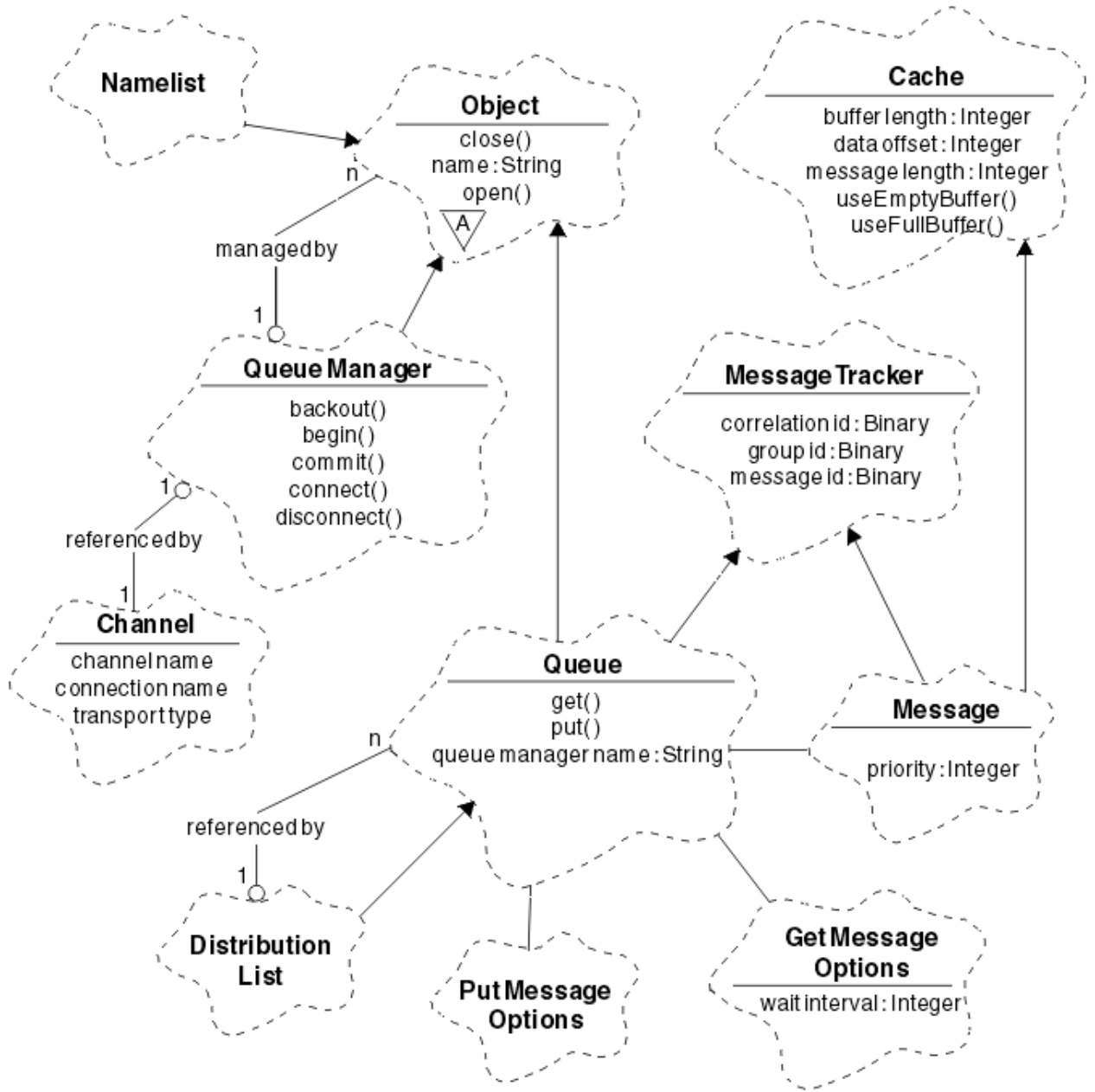
Şekil 59. IBM MQ C++ sınıfları (kuyruk yönetimi)
