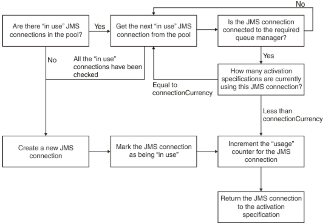
Şekil 51. WebSphere Application Server V7.5 ve V8.0 -bağlantı havuzunun nasıl çalıştığı
