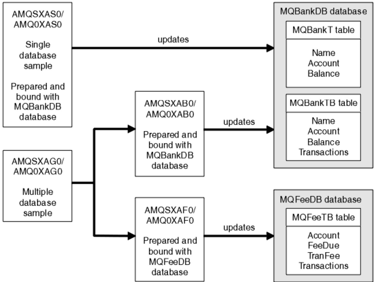
Şekil 135. Veritabanı koordinasyonu örnekleri
