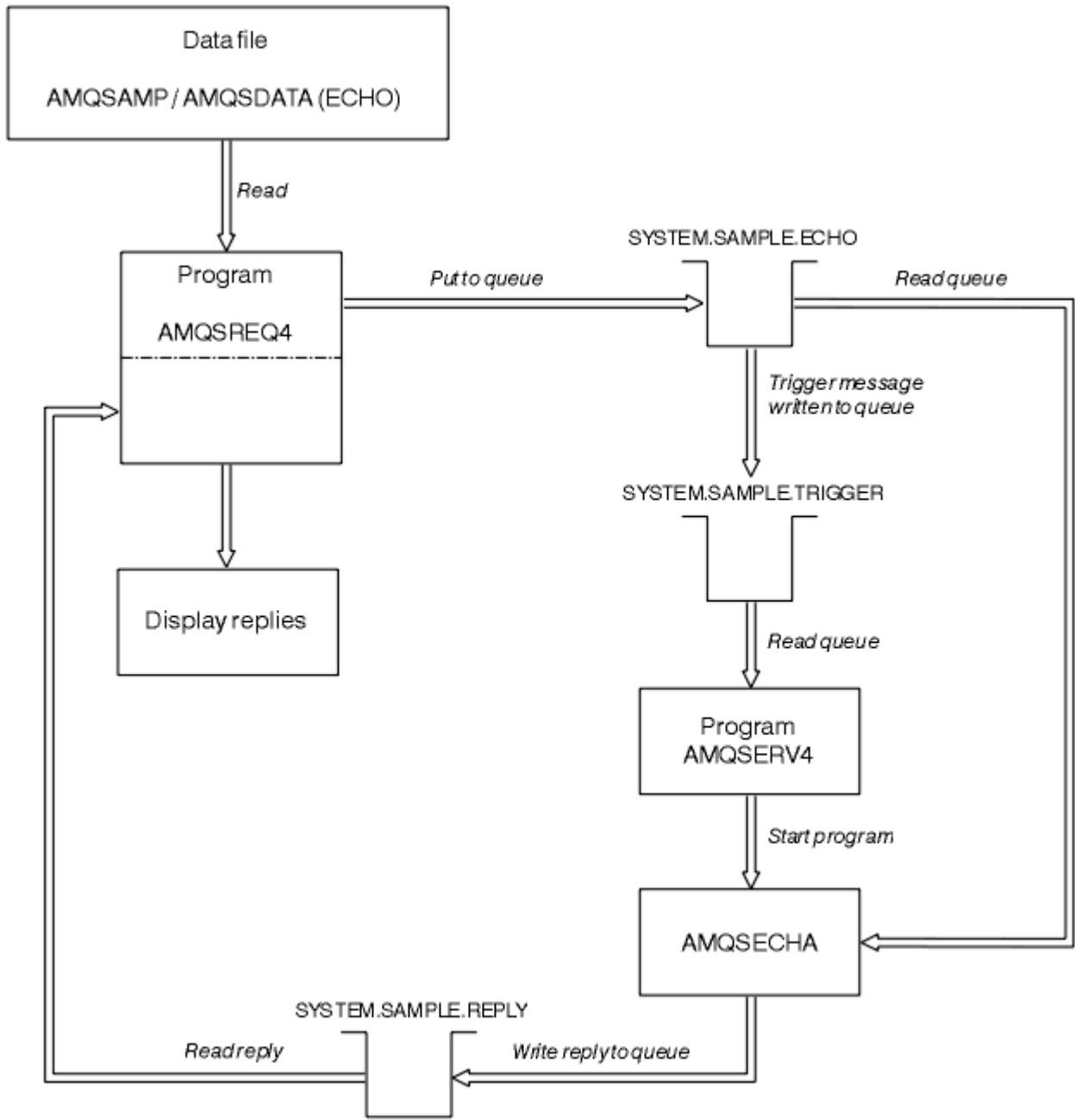
Şekil 140. Örnek IBM i Client/Server (Echo) programı akış şeması
