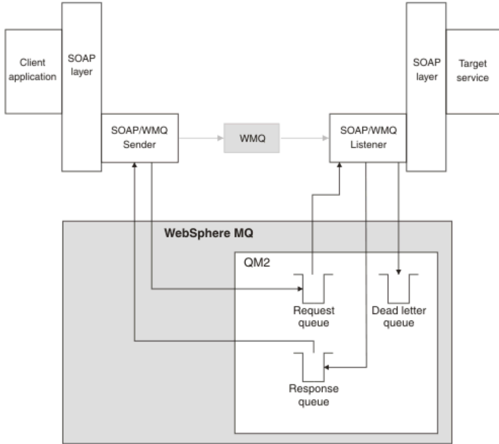
Şekil 160. SOAP/IBM MQ tarafından kullanılan kuyruklar (tek kuyruk yöneticisi)
