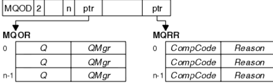
Şekil 62. C içinde bir dağıtım listesinin açılması
