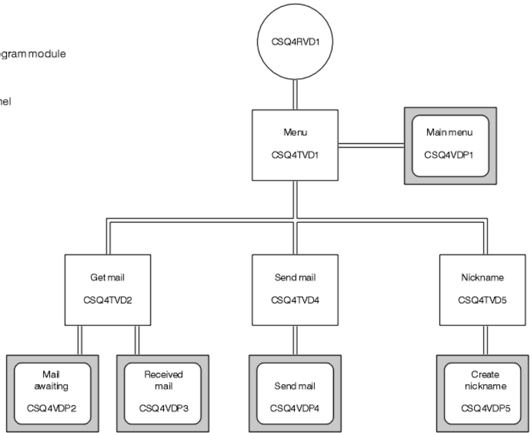
Şekil 147. Posta Yöneticisinin TSO sürümlerine ilişkin programlar ve panolar
