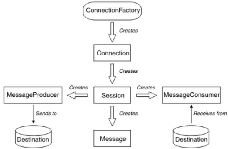
Şekil 11. JMS nesneleri ve ilişkileri
