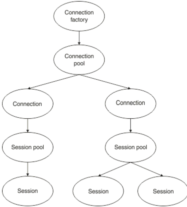
Şekil 50. Bağlantı havuzları ve oturum havuzları
