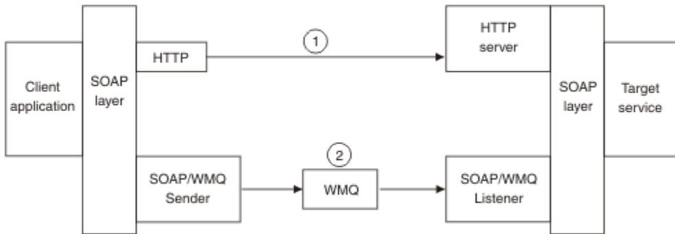
Şekil 159. SOAP için IBM MQ iletimi genel bakış
