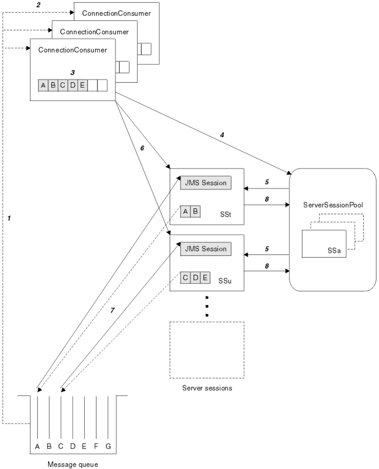
Şekil 53. ServerSessionhavuzu ve ServerSession işlevi
