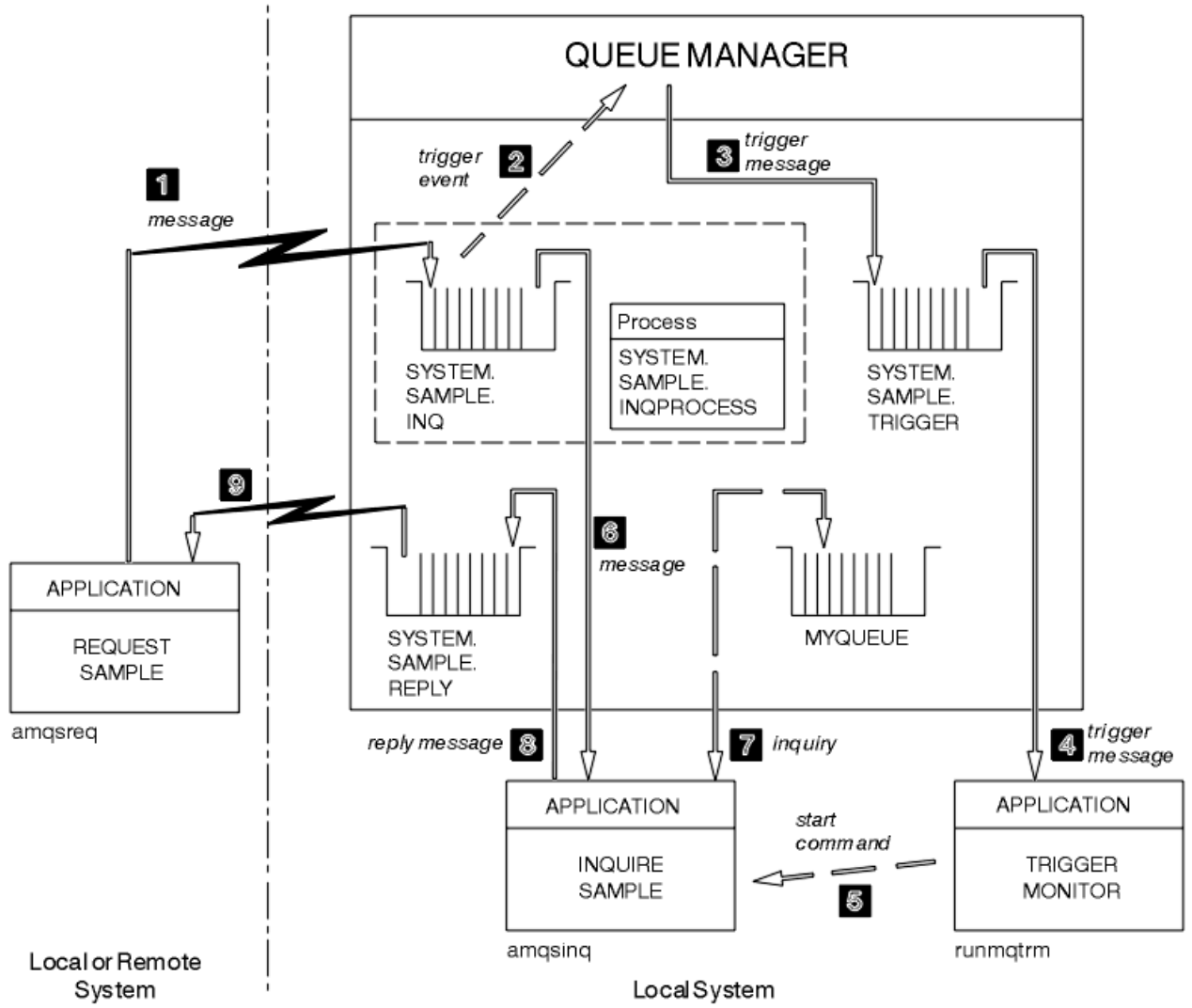
Şekil 139. Tetikleme kullanarak istek ve sorgulama örnekleri
