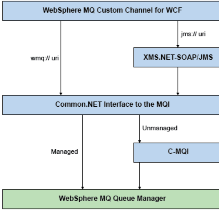
Şekil 157. SOAP/Non-JMS arabirimi için WCF mimarisi
