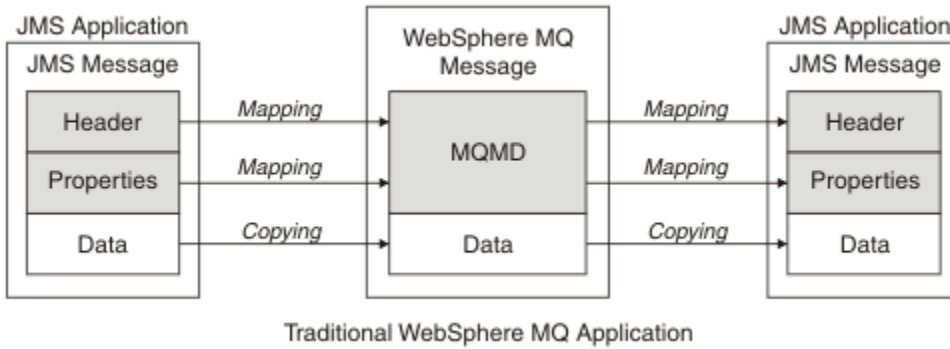
Şekil 13. JMS iletilerinin, MQRFH2 üstbilgisi içermeyen IBM MQ iletilerine nasıl dönüştürülebileceği
