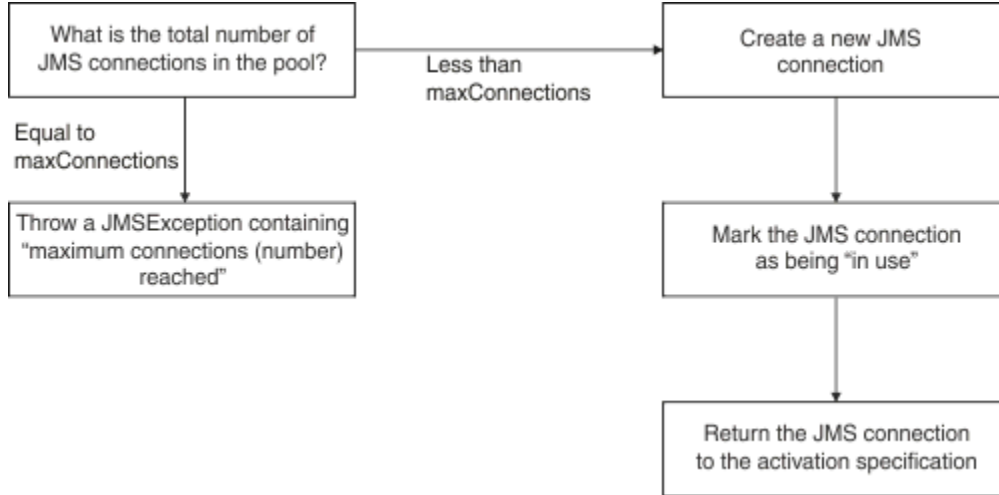
Şekil 52. WebSphere Application Server V8.5 -bağlantı havuzunun nasıl çalıştığı
