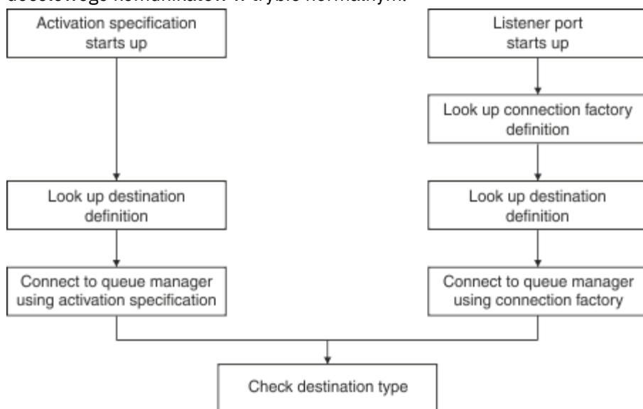
Rysunek 49. Tryb standardowy
