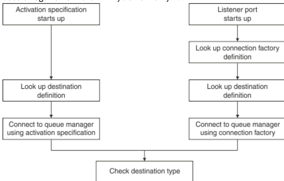
Rysunek 9. Tryb standardowy
