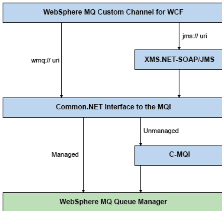
Rysunek 157. Architektura WCF dla interfejsu Non-SOAP/Non-JMS
