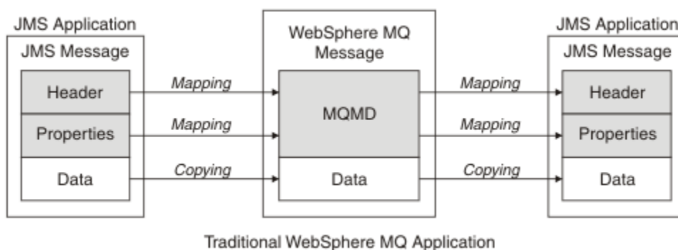
Rysunek 13. Sposób transformowania komunikatów produktu JMS na komunikaty produktu IBM MQ bez nagłówka MQRFH2 .
