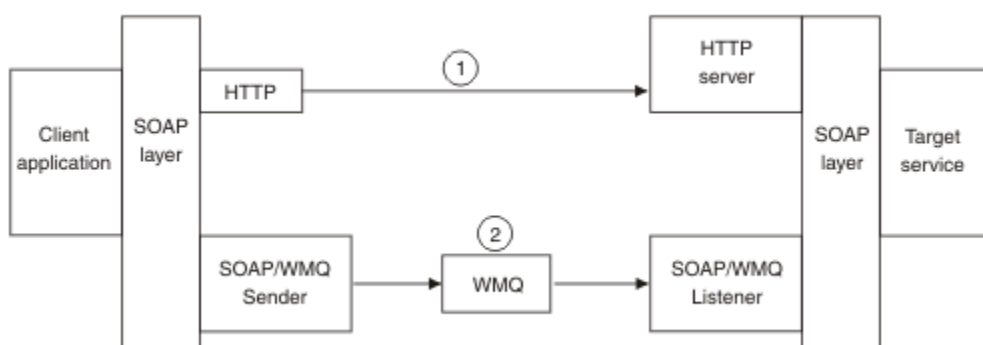
Rysunek 159. Przegląd transportu produktu IBM MQ dla protokołu SOAP
