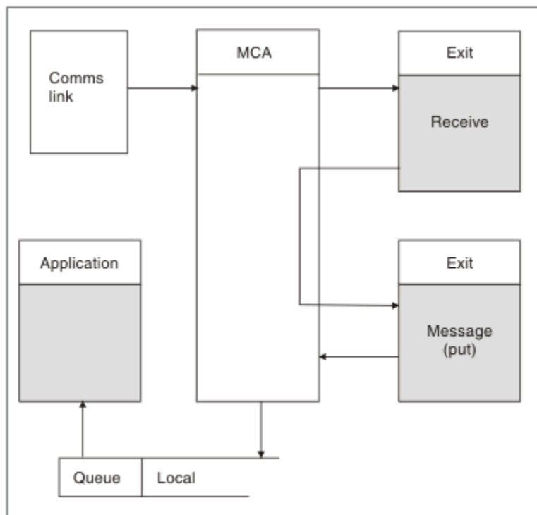
Rysunek 112. Przykład wyjścia odbierania na końcu kanału komunikatów kanału komunikatów
