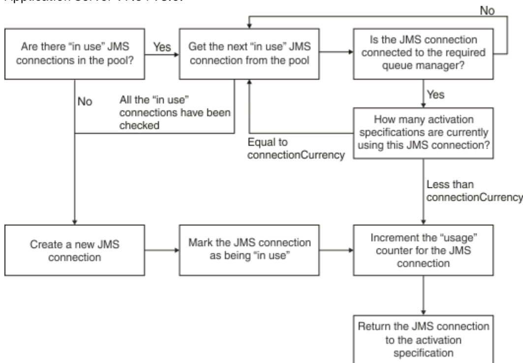
Rysunek 51. WebSphere Application Server V7.5 i V8.0 -sposób działania puli połączeń
