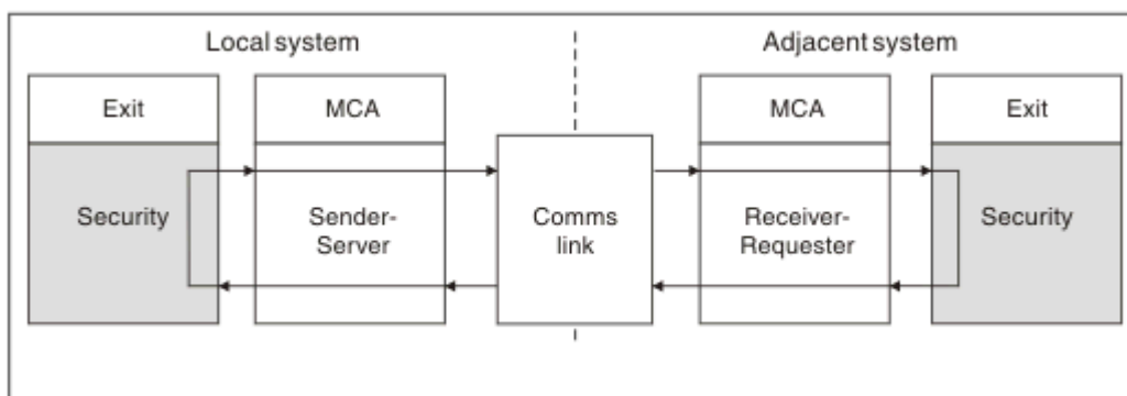
Rysunek 110. Pętla wyjścia zabezpieczeń
