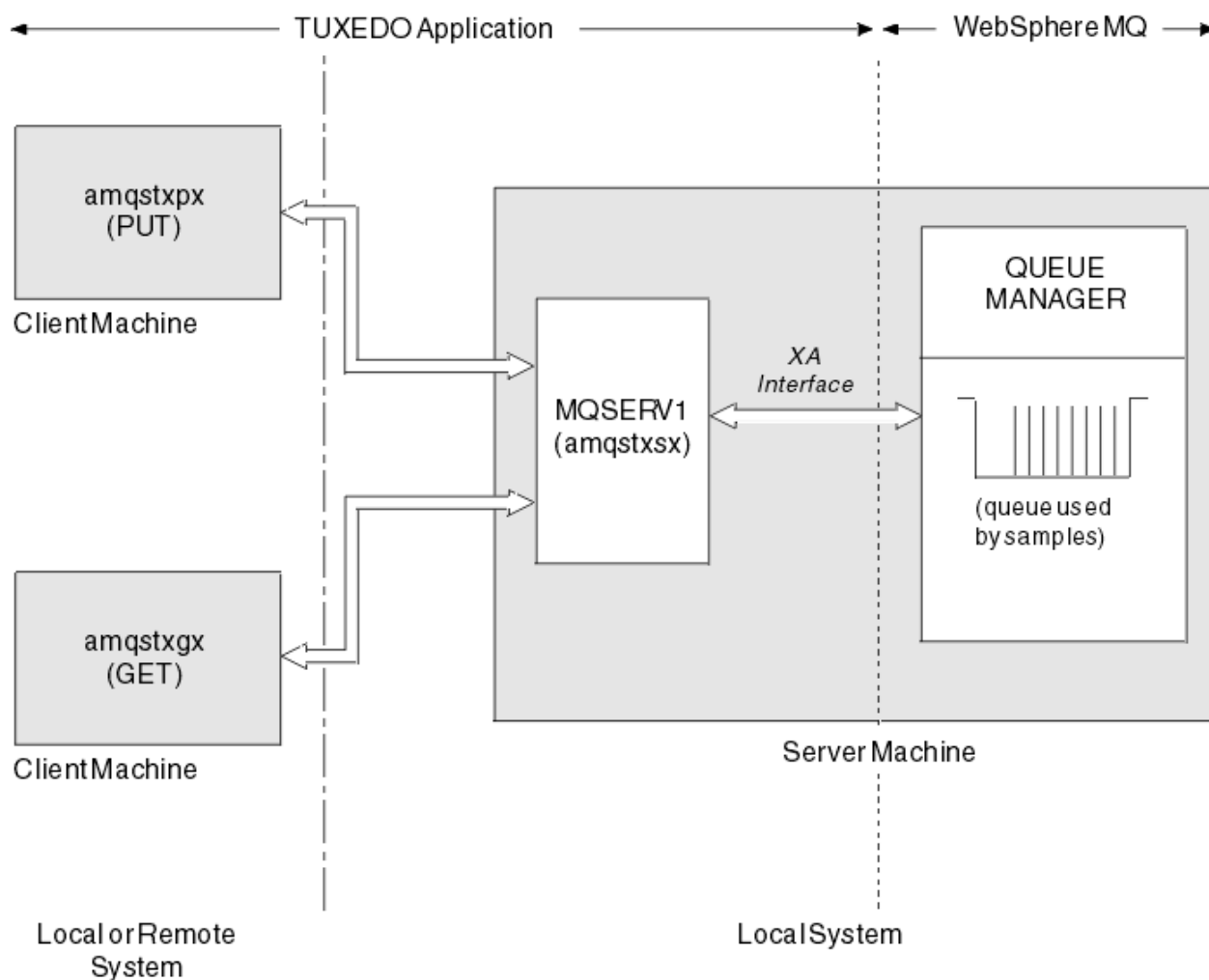
Rysunek 145. Jak próbki TUXEDO współpracują ze sobą
