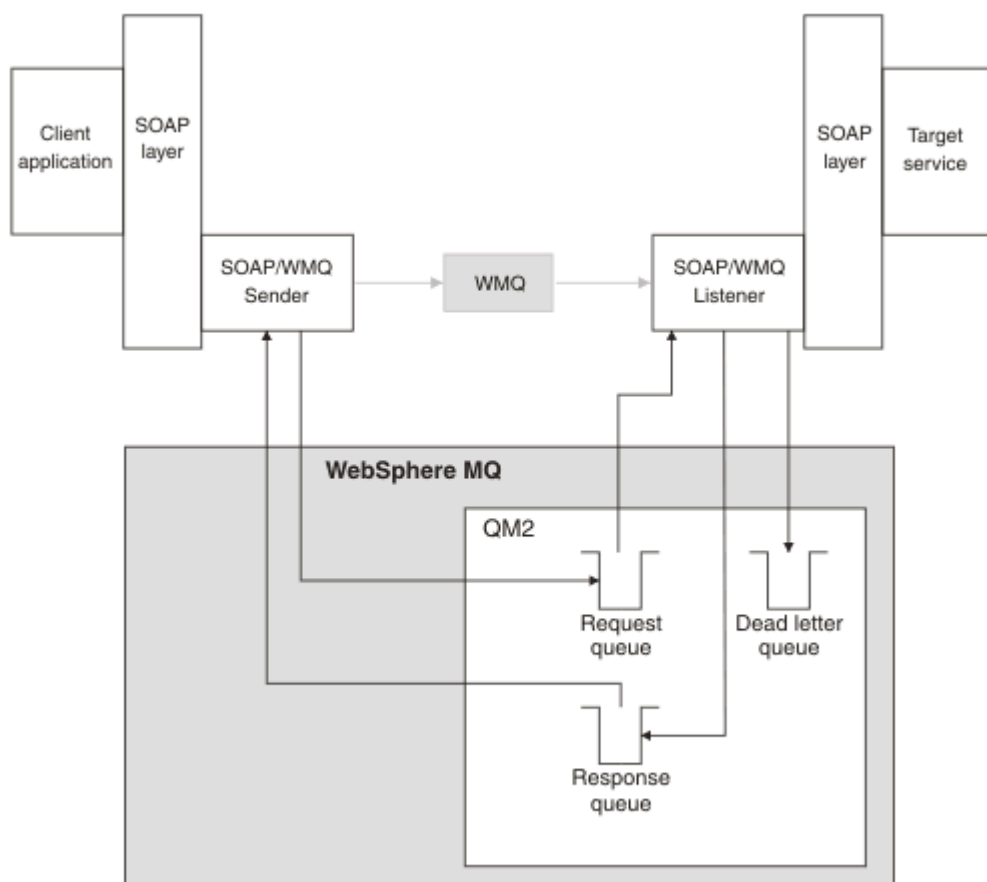
Rysunek 160. Kolejki używane przez SOAP/IBM MQ (pojedynczy menedżer kolejek)
