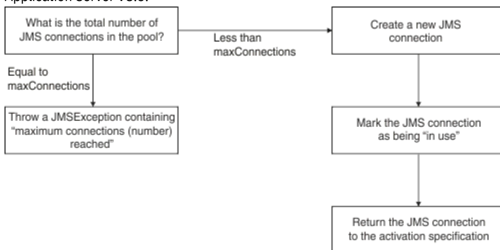
Rysunek 52. WebSphere Application Server V8.5 -sposób działania puli połączeń
