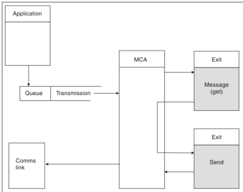
Rysunek 111. Przykład wyjścia wysyłania na końcu kanału komunikatów nadawcy
