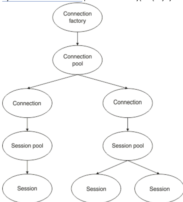
Rysunek 10. Pule połączeń i pule sesji
