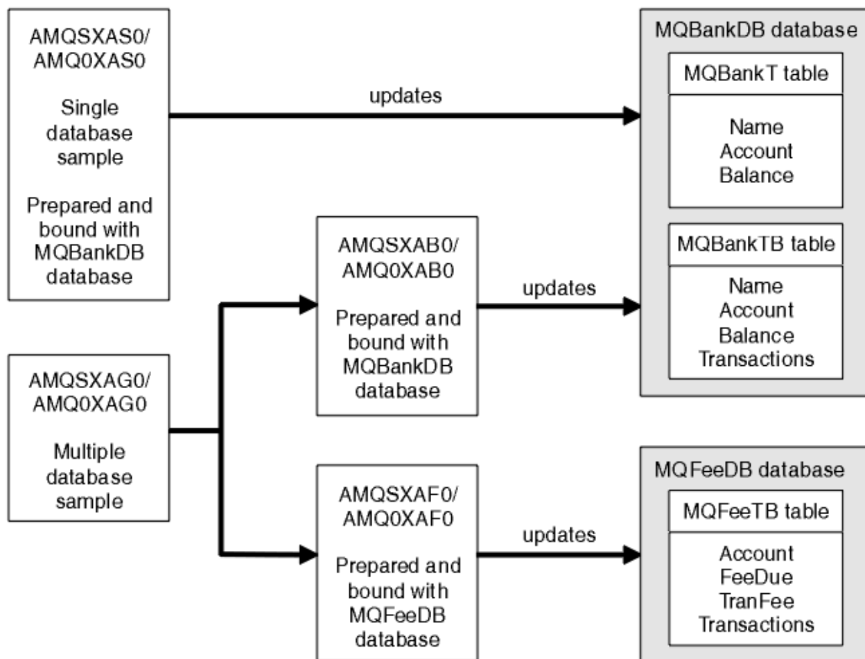
Rysunek 135. Przykłady koordynacji bazy danych
