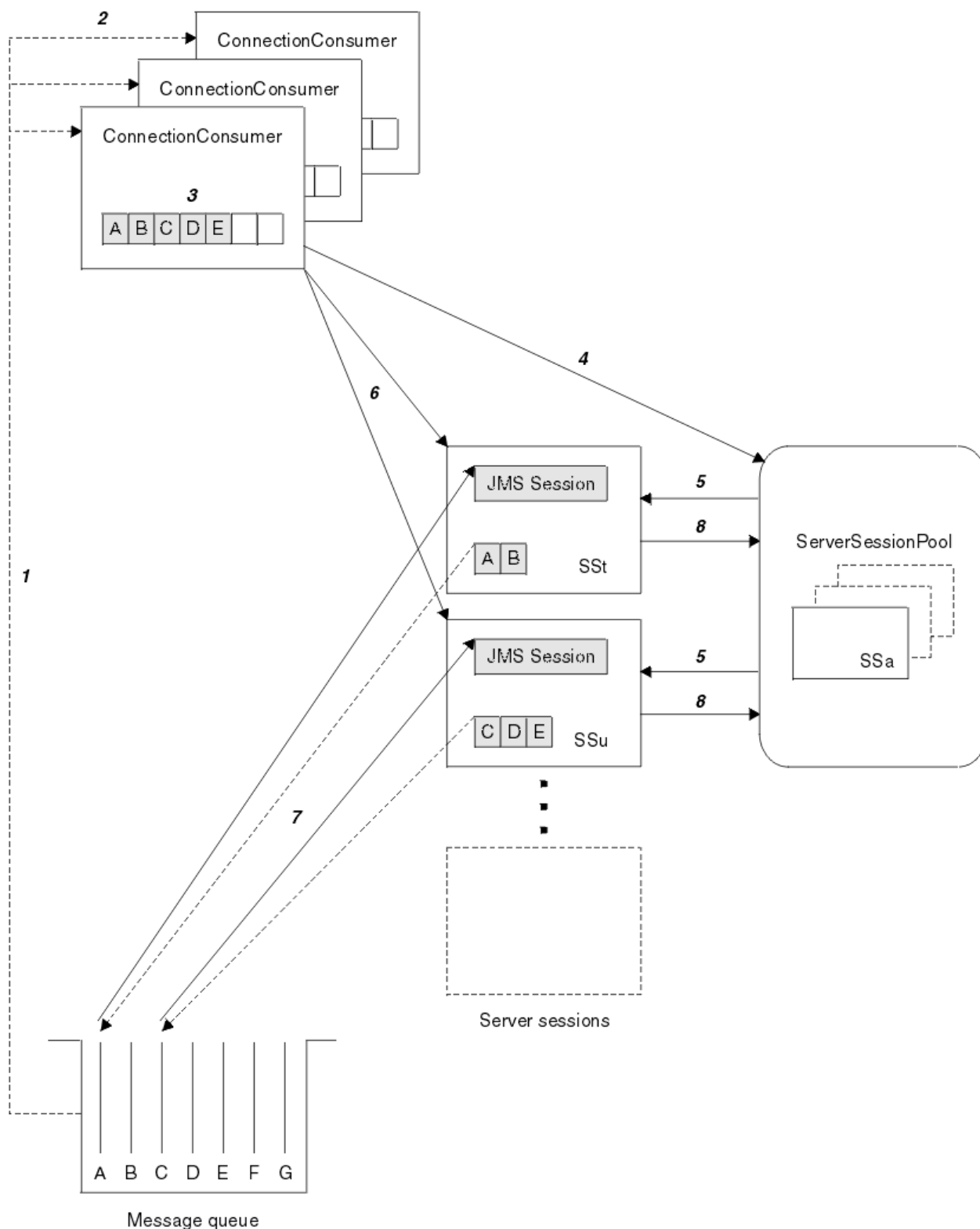
Rysunek 53. Funkcje ServerSessionPool i ServerSession
