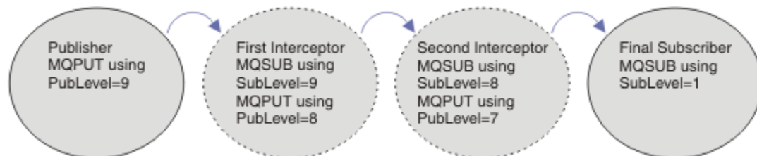
Rysunek 91. Sekwencja przechwytyjących subskrybentów
