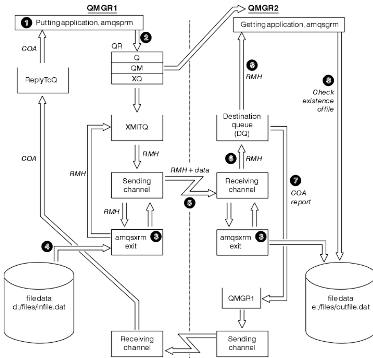
Rysunek 138. Uruchamianie przykładów komunikatów odniesienia
