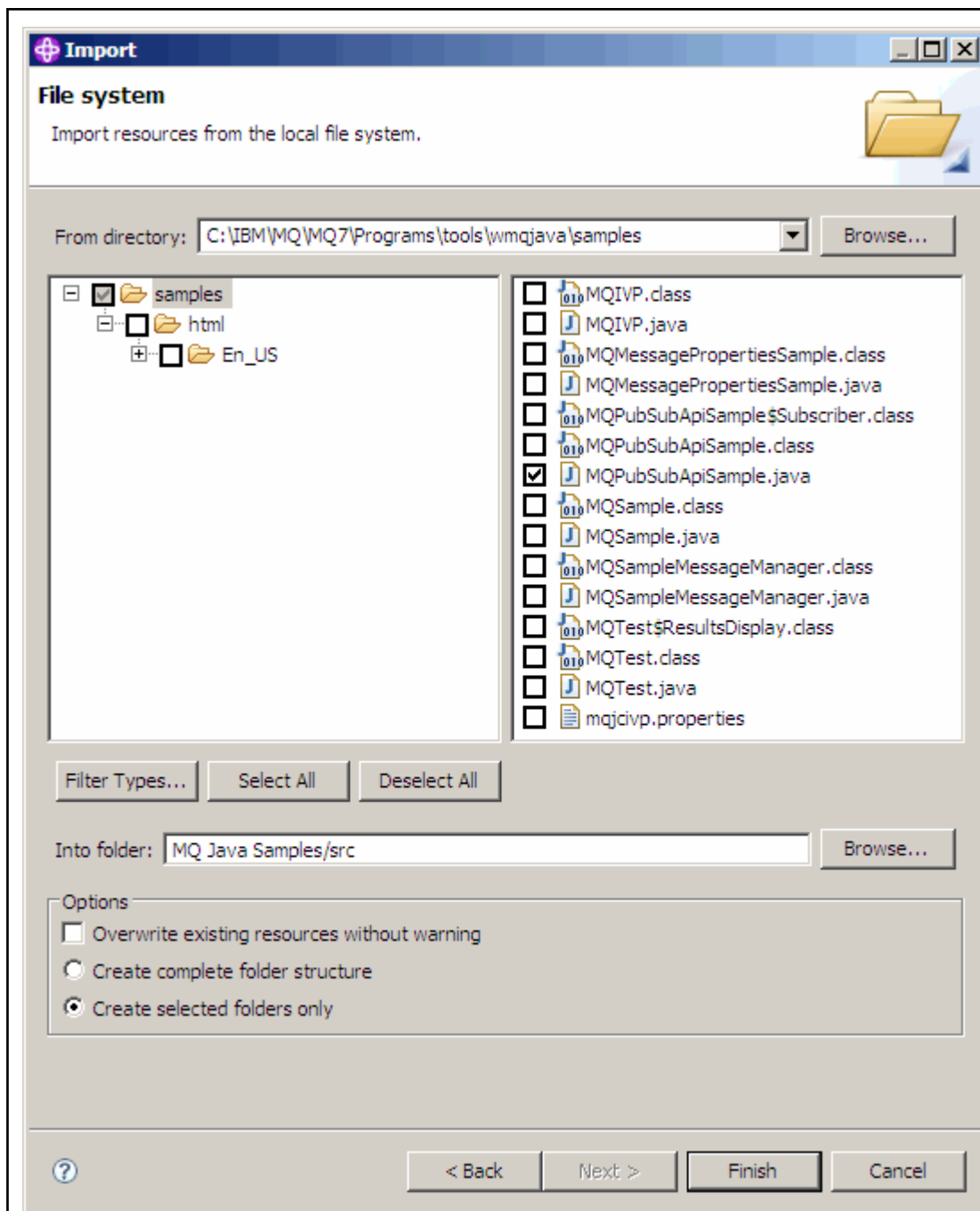
Rysunek 137. Import systemu plików
