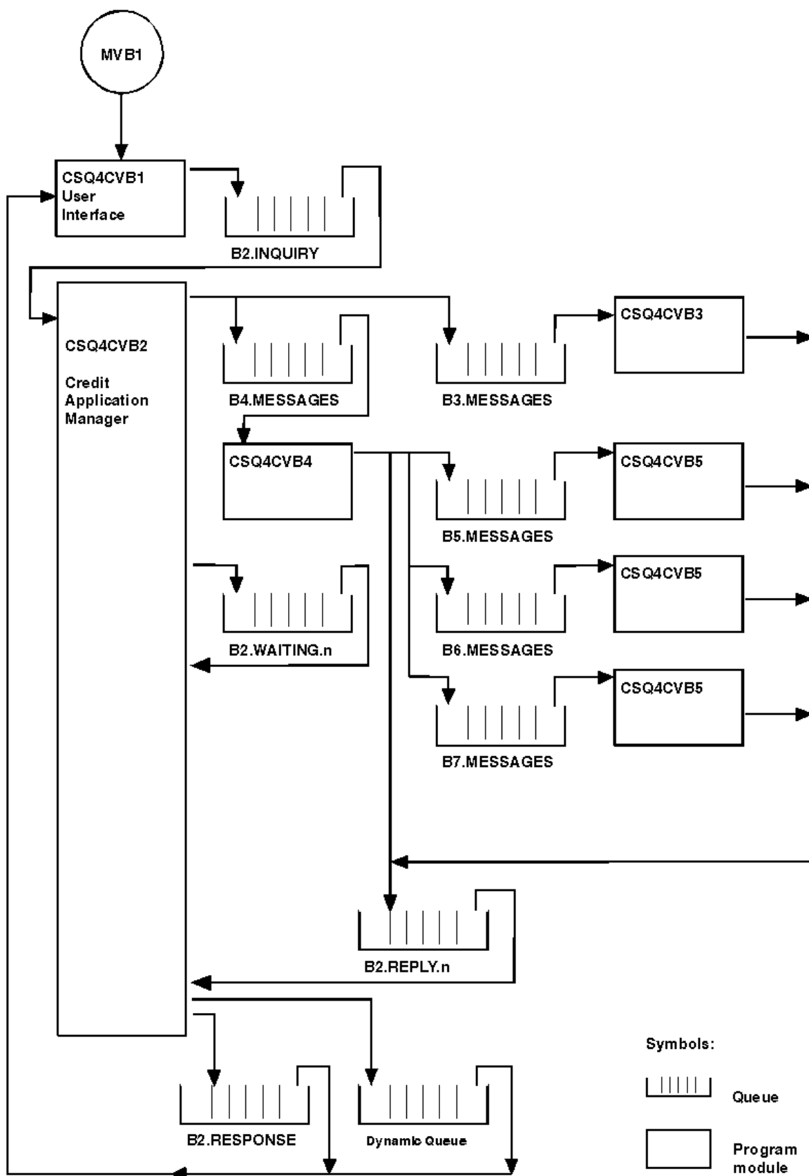
Rysunek 152. Programy i kolejki dla przykładowej aplikacji Sprawdzenie uznania (tylko programy w języku COBOL)
