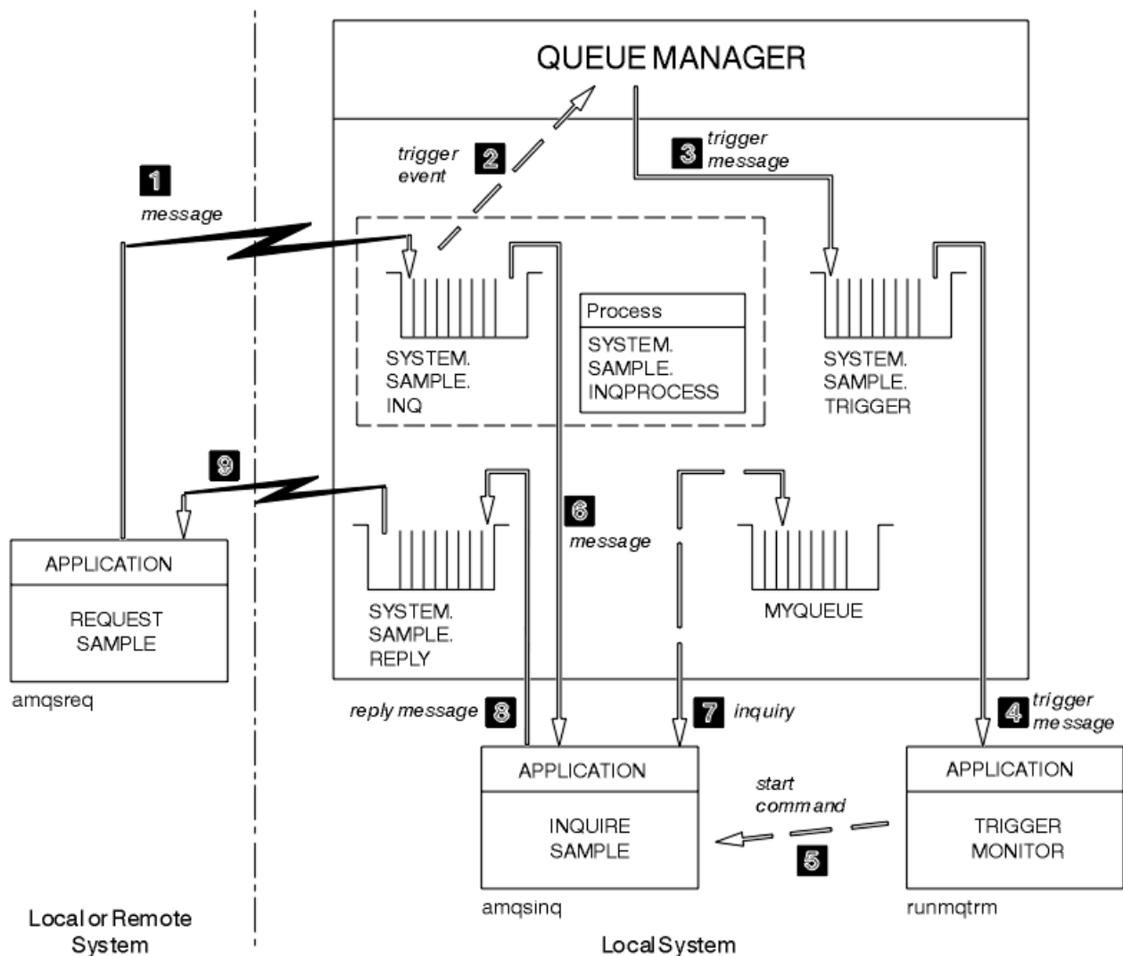
Rysunek 139. Przykłady żądań i uzyskiwania informacji przy użyciu wyzwalania
