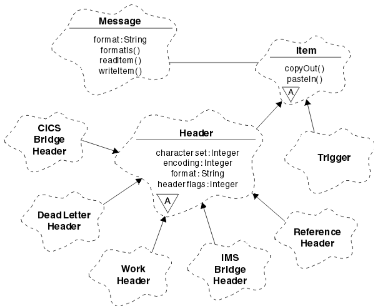
Rysunek 58. IBM MQ Klasy C++ (obsługa pozycji)
