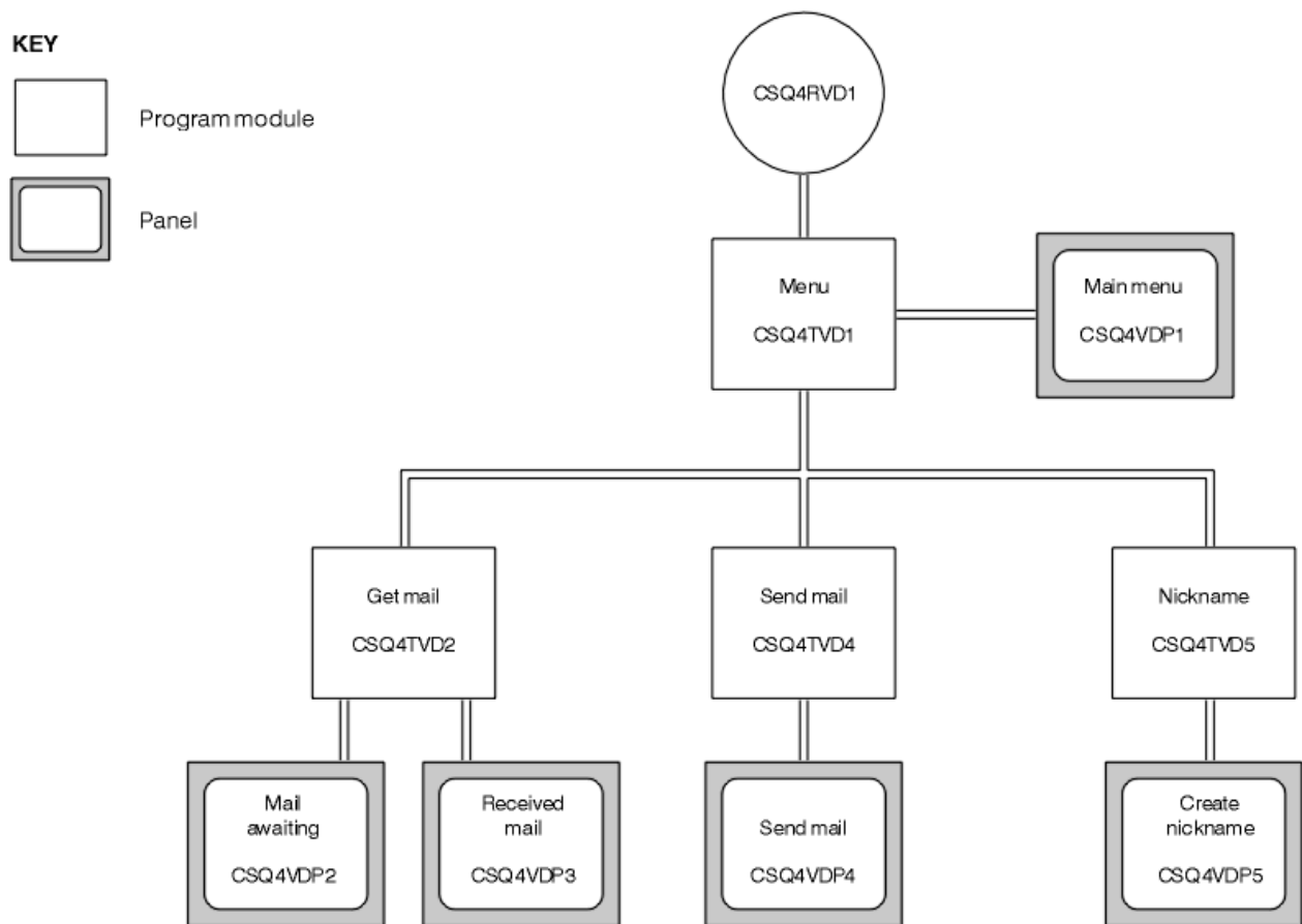
Rysunek 147. Programy i panele dla wersji TSO programu Mail Manager
