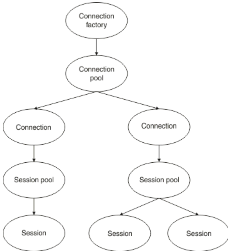
그림 10. 연결 풀 및 세션 풀
