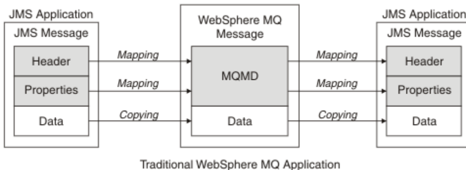
그림 13. JMS 메시지를 MQRFH2 헤더가 없는 IBM MQ 메시지로 변환하는 방법
