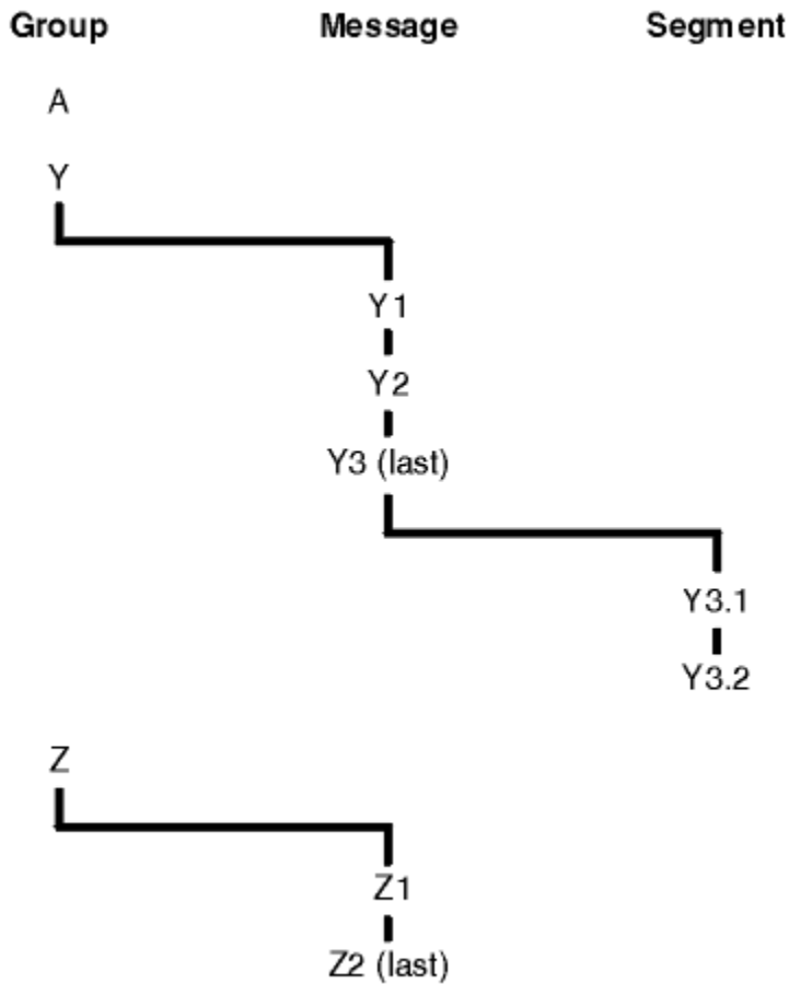
그림 66. 큐의 논리 순서
