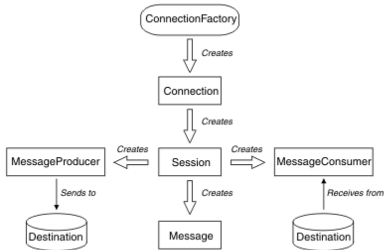
그림 11. JMS 오브젝트 및 해당 관계
