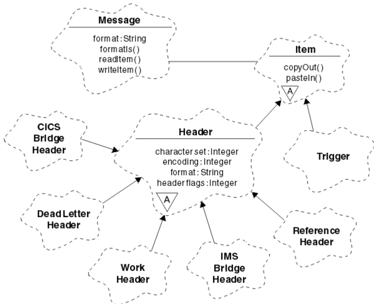
그림 58. IBM MQ C++ 클래스(항목 핸들링)
