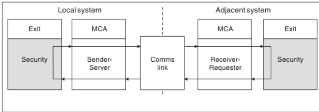
그림 110. 보안 엑시트 루프
