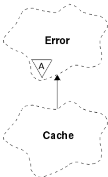
Figura 48. Classe ImqCache
