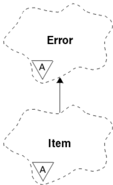
Figura 57. classe ImqItem
