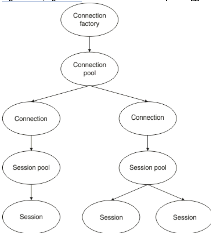
Figura 50. Pool di connessioni e pool di sessione
