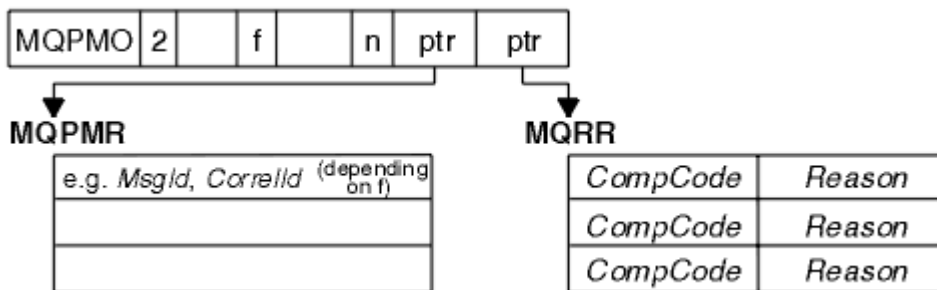
Figura 64. Inserimento di un messaggio in un elenco di distribuzione in C
