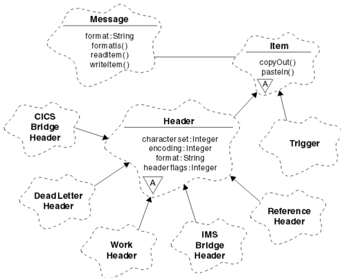
Figura 58. Classi C++ IBM MQ (gestione elementi)
