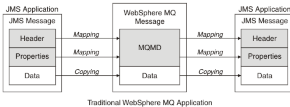
Figura 13. Come i messaggi JMS vengono trasformati in messaggi IBM MQ senza intestazione MQRFH2
