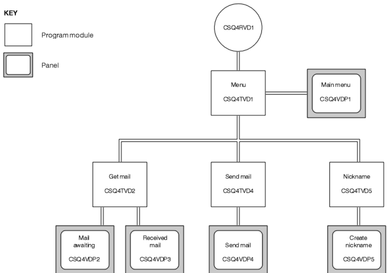
Figura 147. Programmi e pannelli per le versioni TSO di Mail Manager
