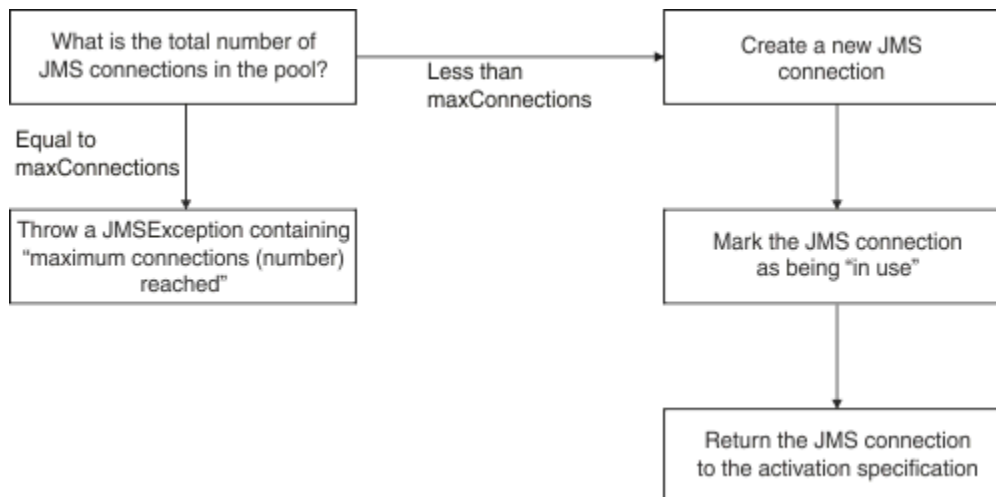
Figura 52. WebSphere Application Server V8.5 - funzionamento del pool di connessioni
