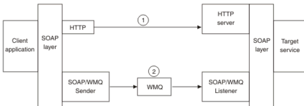
Figura 159. Panoramica del trasporto IBM MQ per SOAP
