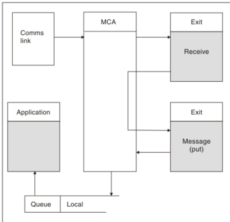
Figura 112. Esempio di un'uscita di ricezione all'estremità del destinatario del canale di messaggi
