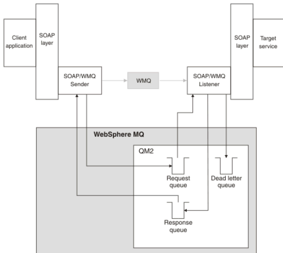
Figura 160. Code utilizzate da SOAP/IBM MQ (gestore code singolo)
