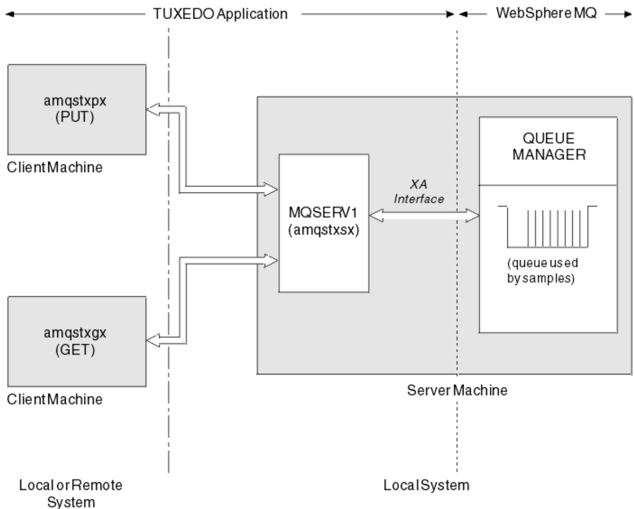
Figura 145. Funzionamento degli esempi TUXEDO
