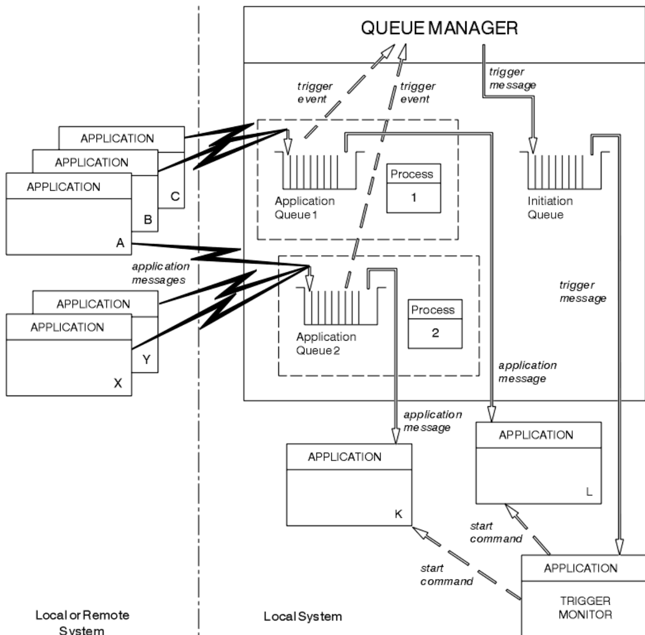
Figura 101. Relazione delle code all'interno del trigger
