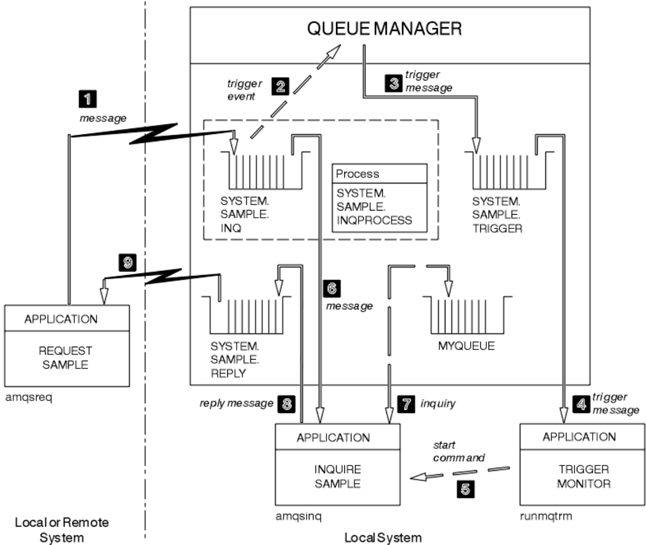
Figura 139. Richiedi e richiedi esempi utilizzando il trigger
