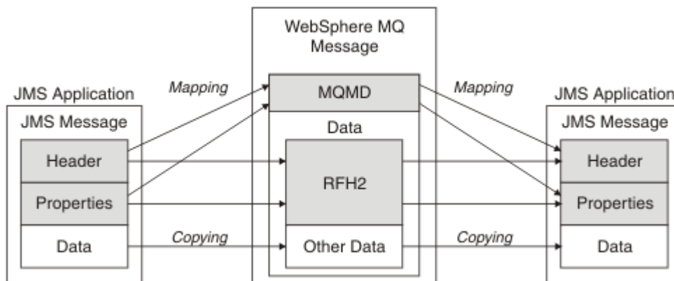
Figura 12. Come vengono trasformati i messaggi tra JMS e IBM MQ utilizzando l'intestazione MQRFH2
