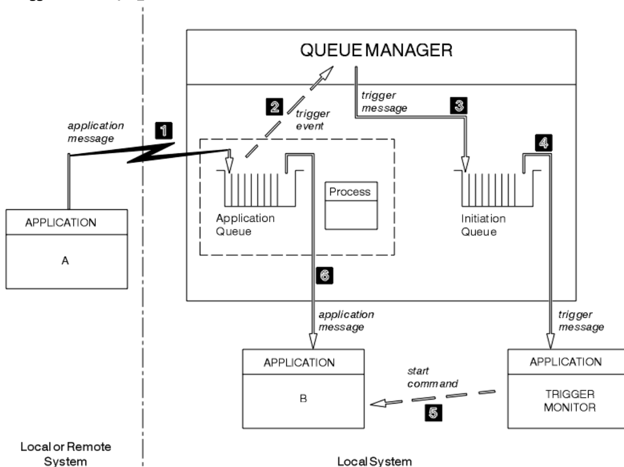
Figura 100. Flusso di messaggi di applicazione e trigger
