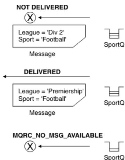
Figura 4. Selezione mediante chiamata MQOPEN
