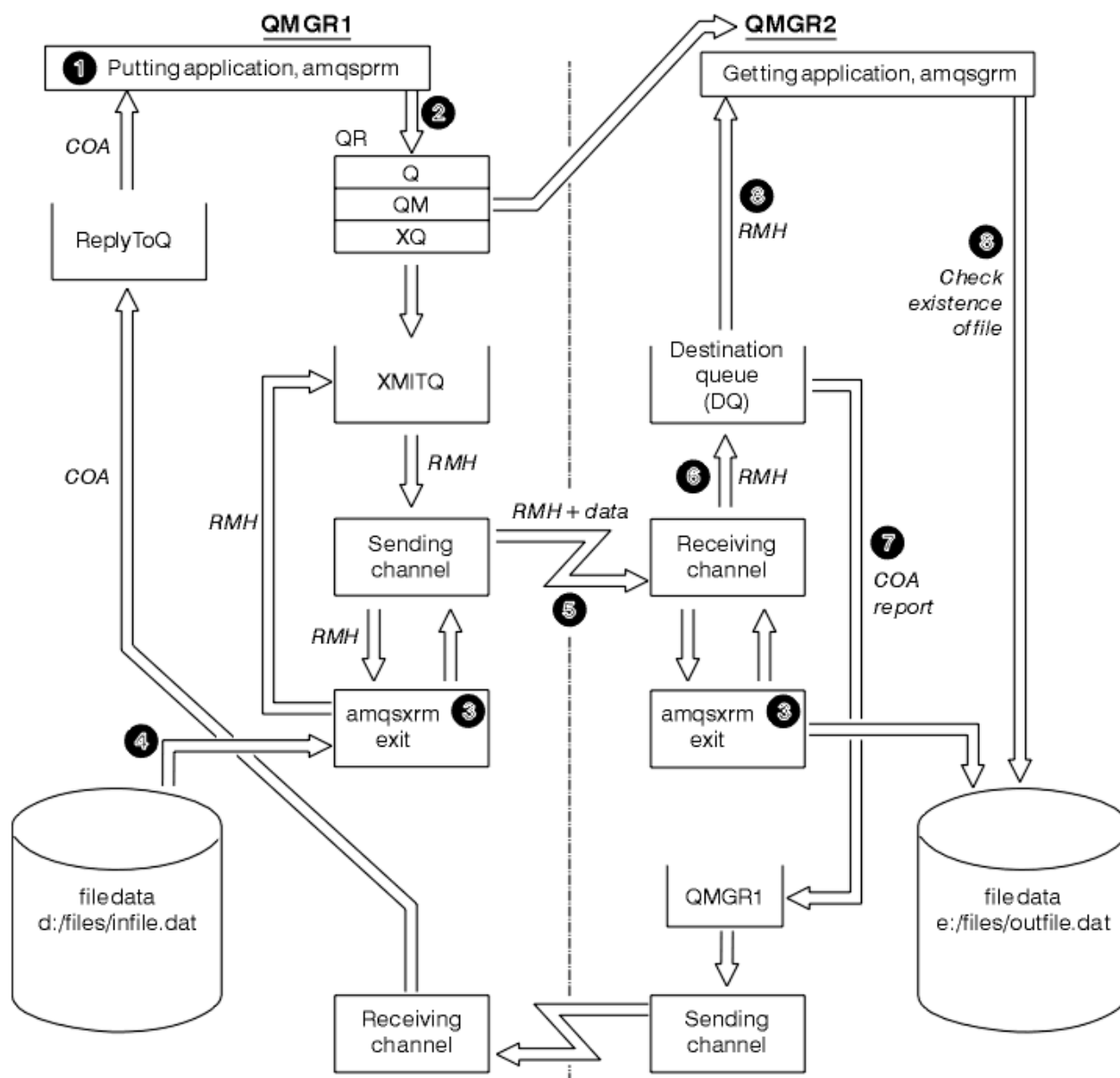
Figura 138. Esecuzione degli esempi del messaggio di riferimento
