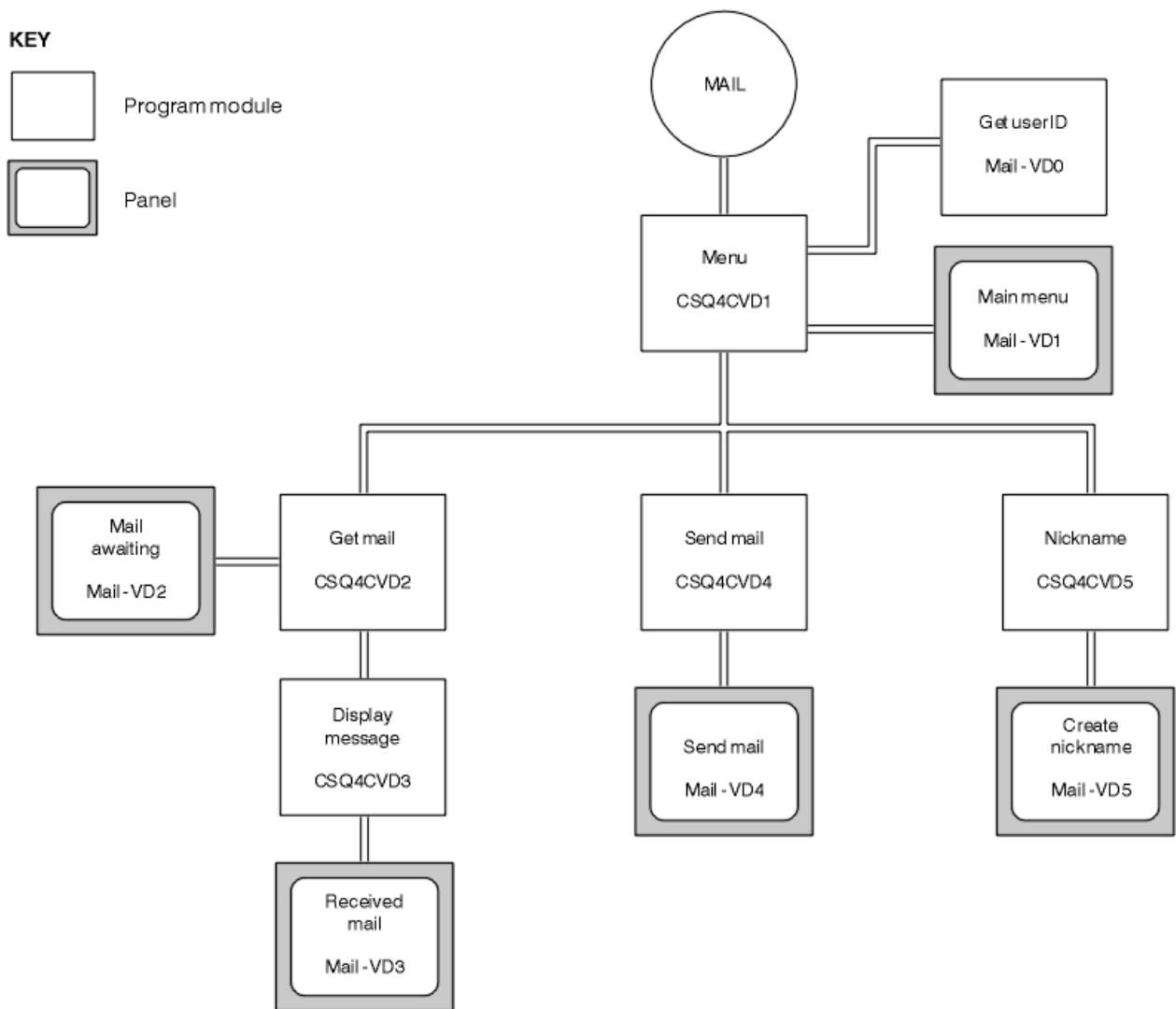
Figura 148. Programmi e pannelli per la versione CICS di Mail Manager
