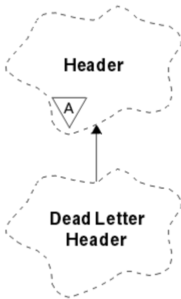
Figure 51. Classe ImqDeadLetterHeader
