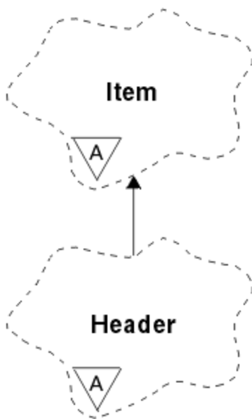
Figure 55. Classe ImqHeader
