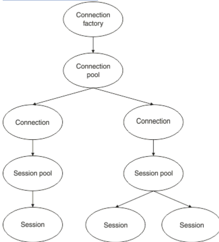
Figura 10. Agrupaciones de conexiones y agrupaciones de sesiones
