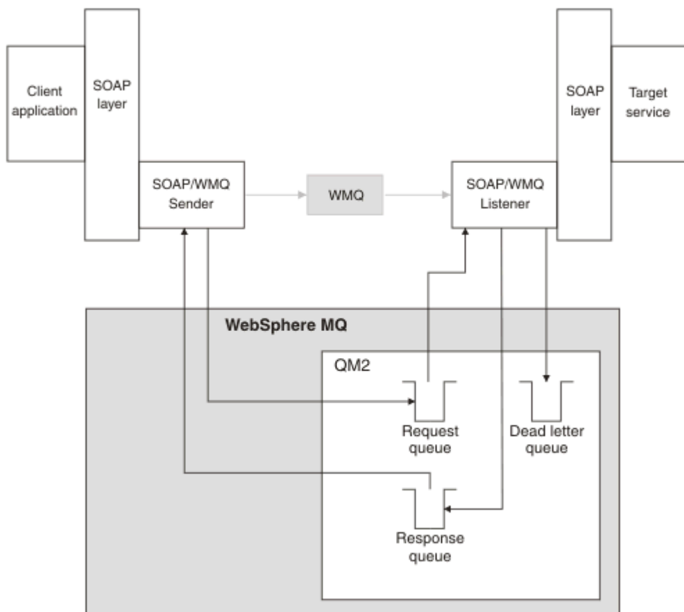
Figura 160. Colas utilizadas por SOAP/IBM MQ (gestor de colas único)
