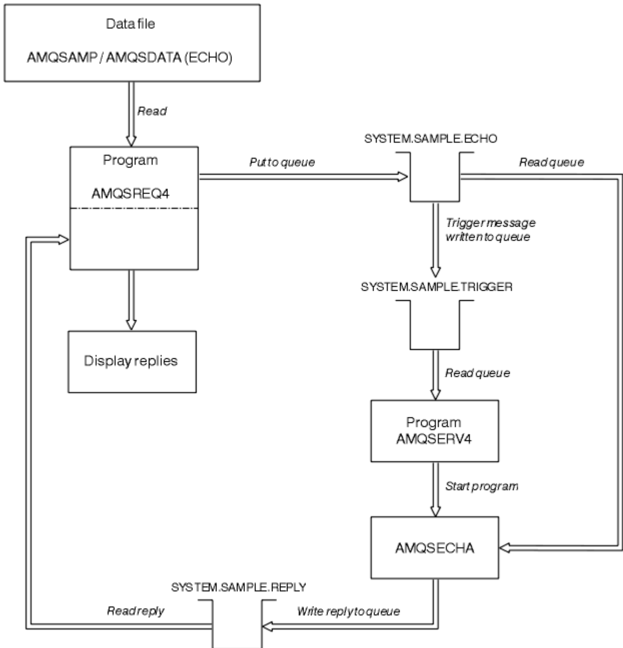
Figura 140. Diagrama de flujo del programa de ejemplo de cliente/servidor IBM i (eco)
