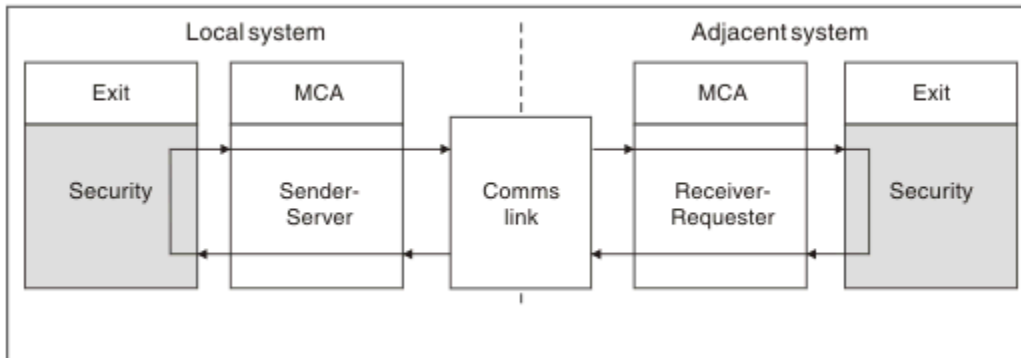
Figura 110. Bucle de salida de seguridad
