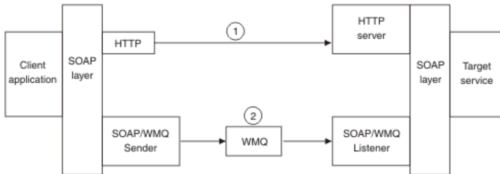
Figura 159. Visión general del transporte IBM MQ para SOAP
