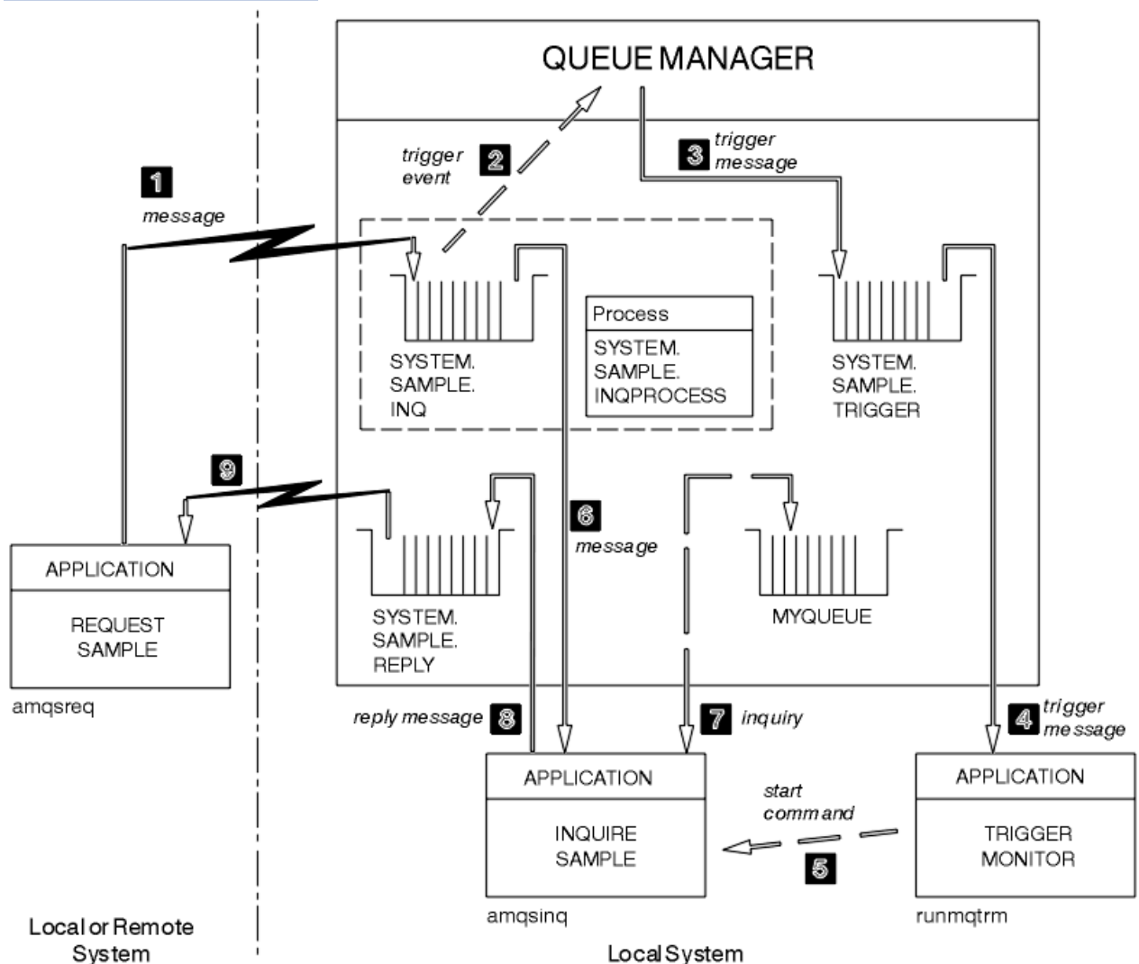
Figura 139. Ejemplos de solicitud y consulta que utilizan el desencadenamiento
