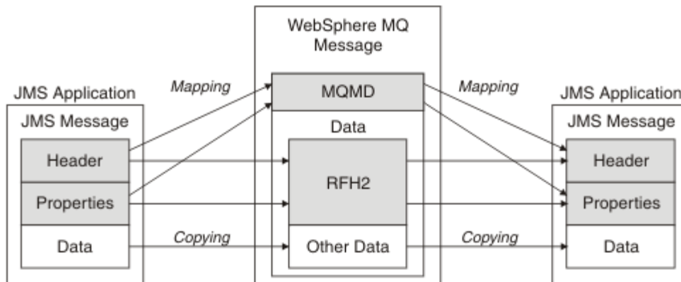
Figura 12. Cómo los mensajes entre JMS y IBM MQ se transforman utilizando la cabecera MQRFH2.
