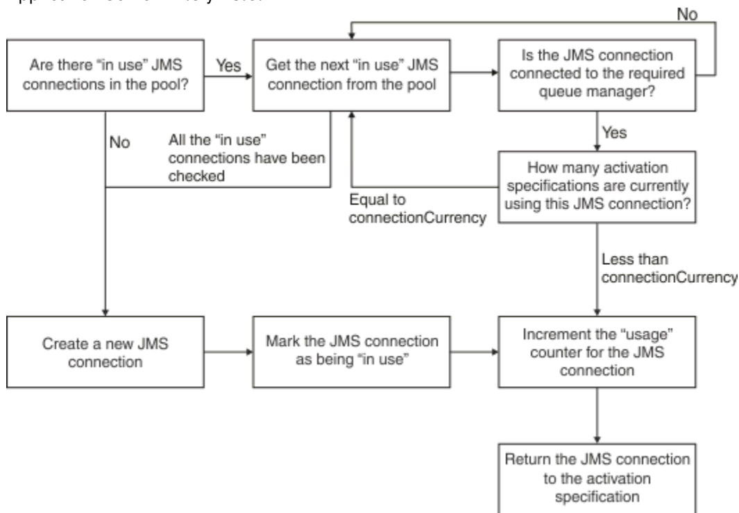
Figura 51. WebSphere Application Server V7.5 y V8.0 - cómo funciona la agrupación de conexiones
