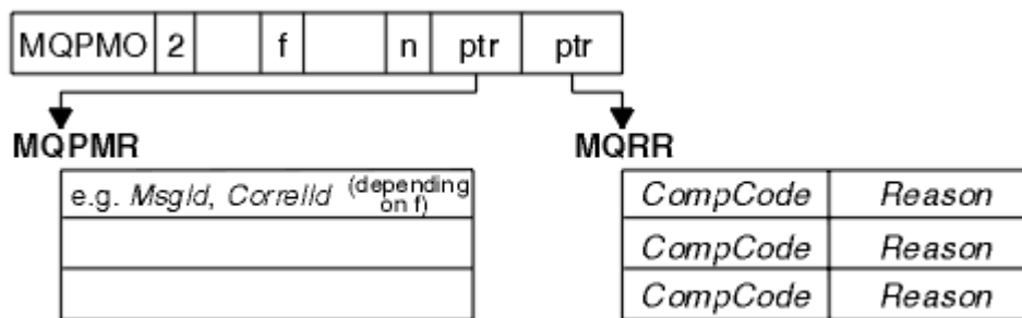
Figura 64. Colocación de un mensaje en una lista de distribución en C
