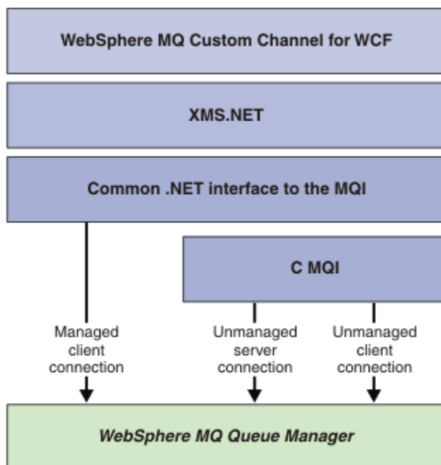
Figura 156. Arquitectura WCF para la interfaz SOAP/JMS
