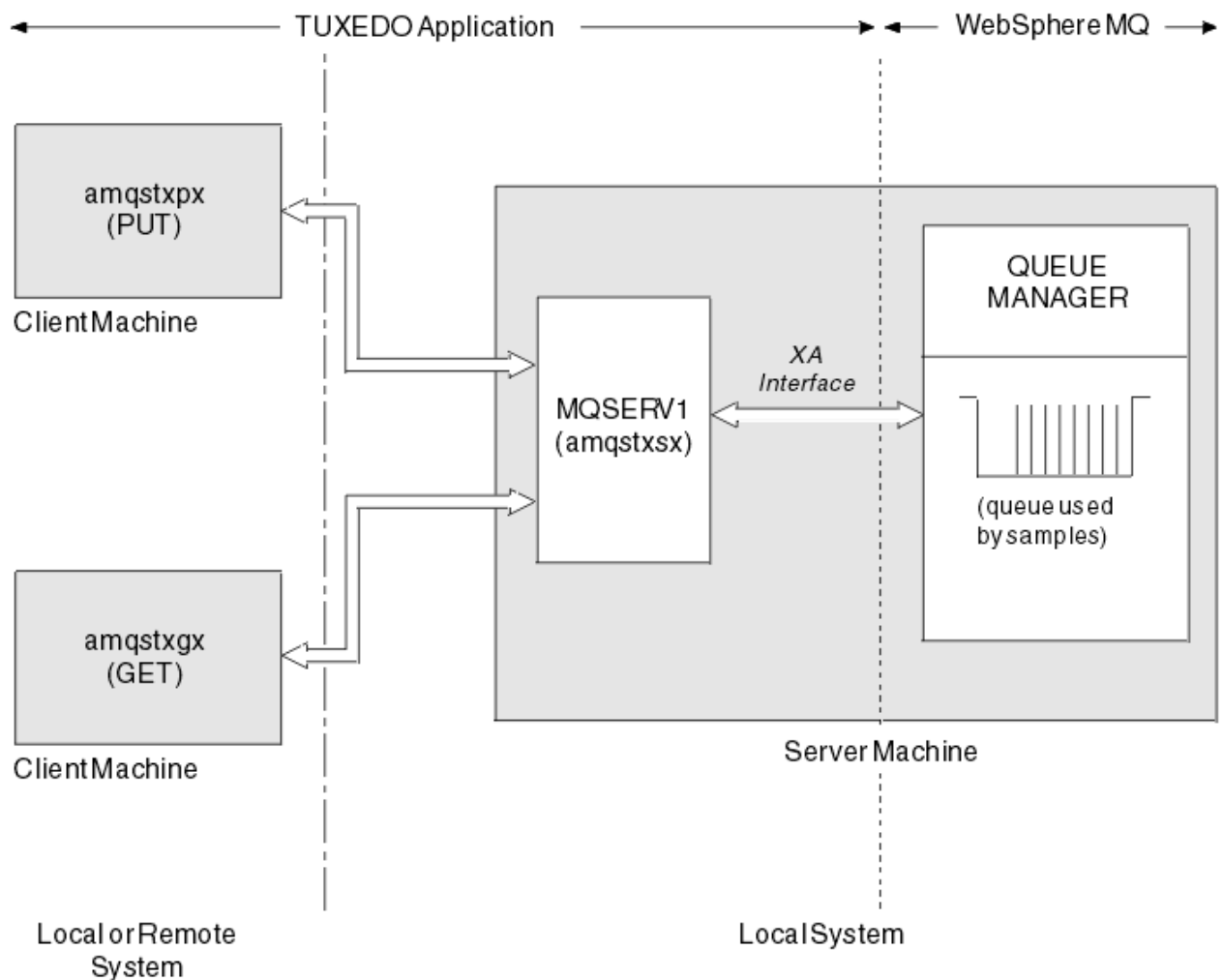
Figura 145. Cómo funcionan juntos los ejemplos de TUXEDO
