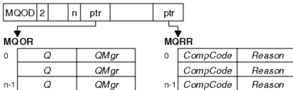
Figura 62. Apertura de una lista de distribución en C
