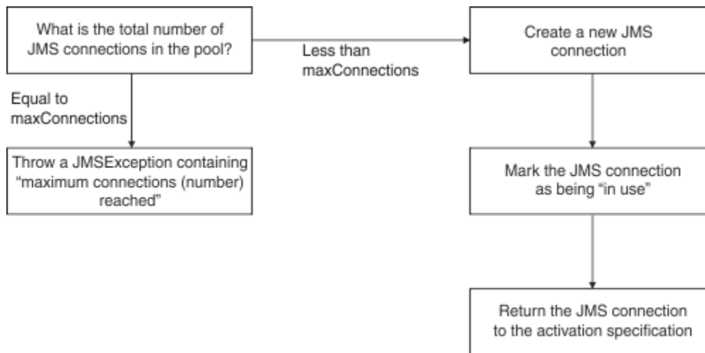
Figura 52. WebSphere Application Server V8.5 - cómo funciona la agrupación de conexiones
