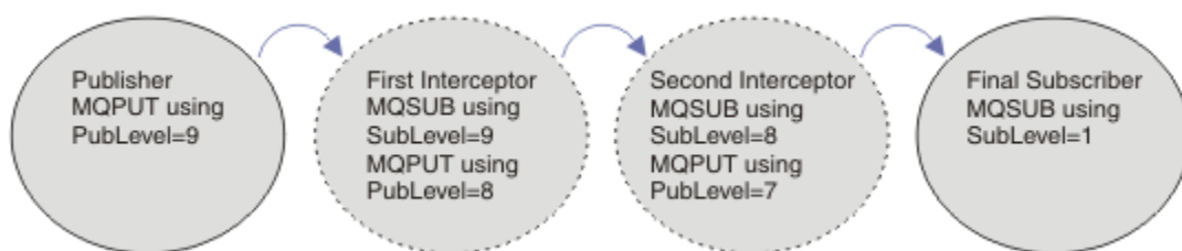
Figura 91. Secuencia de suscriptores de interceptación
