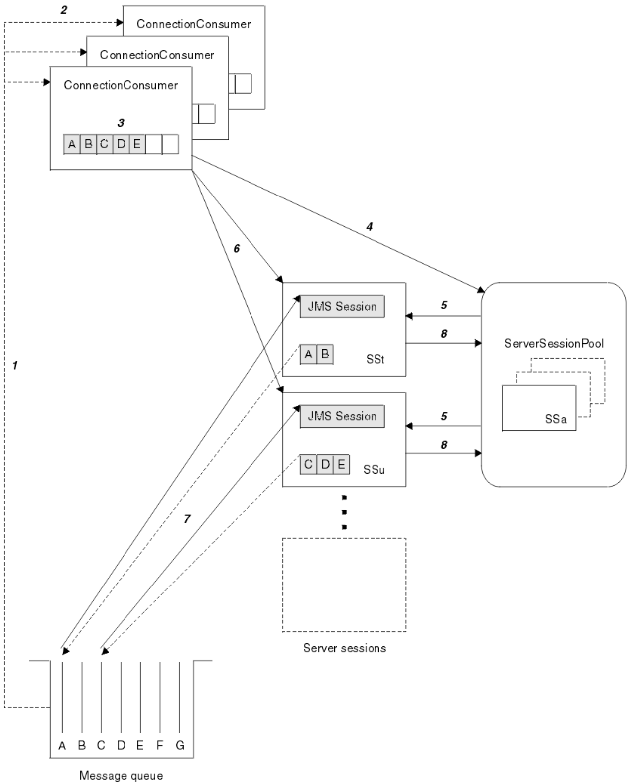
Figura 53. Funciones de ServerSessionPool y ServerSession
