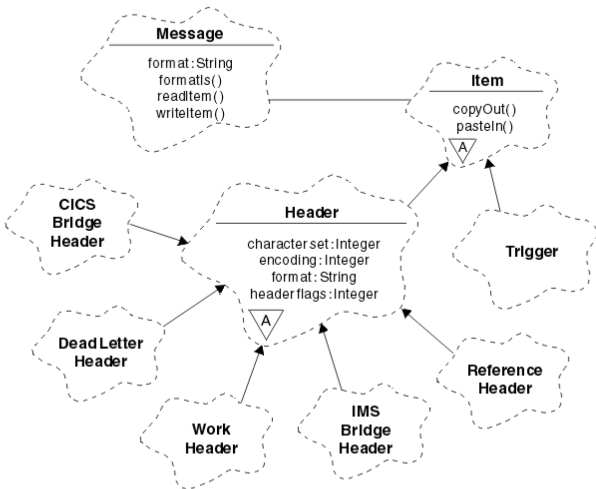
Figura 58. Clases C++ de IBM MQ (manejo de elementos)
