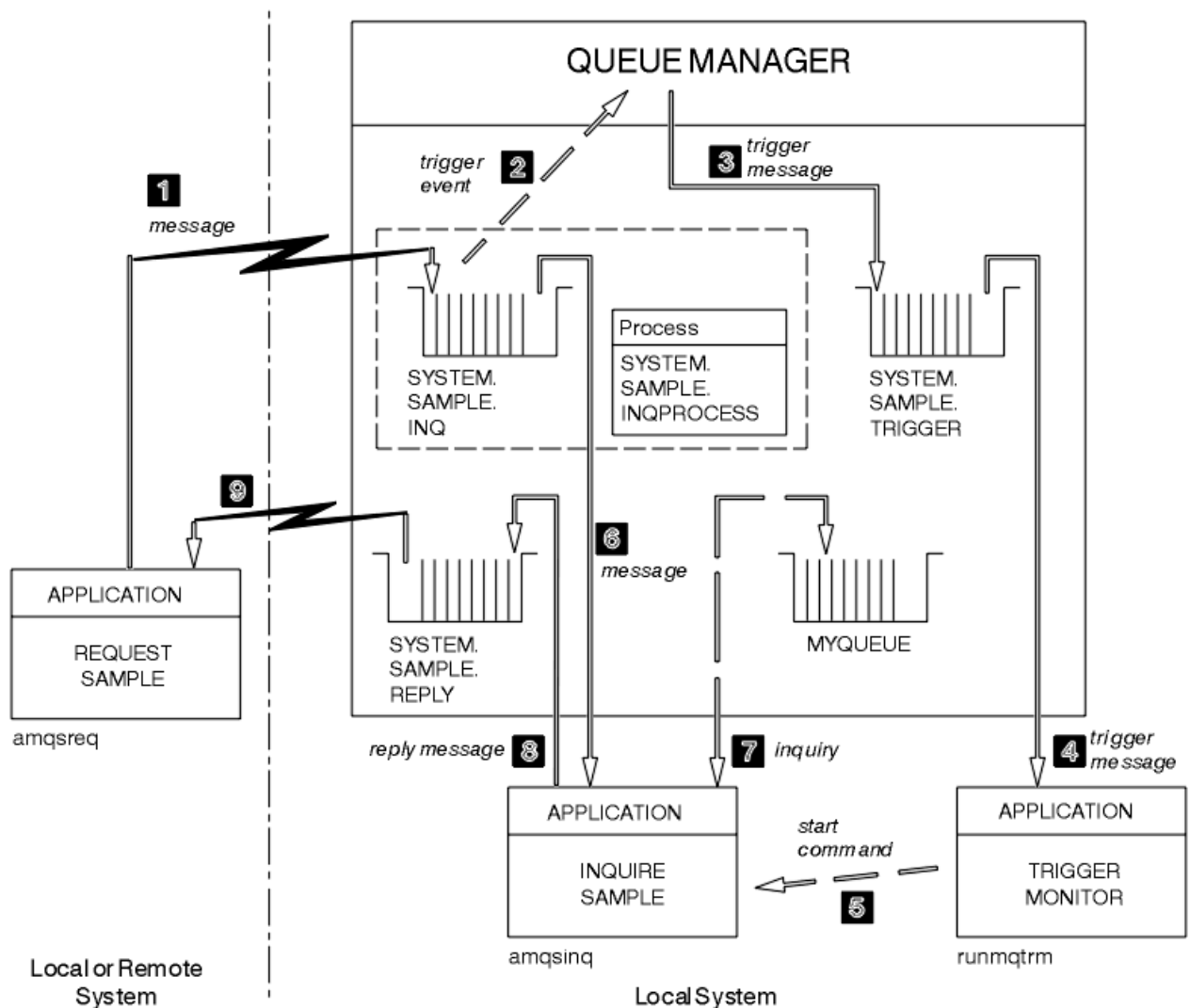
Abbildung 139. Request- und Inquire-Beispielprogramme mittels Triggering ausführen
