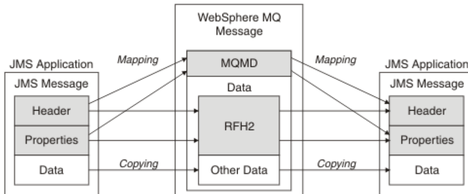
Abbildung 12. Verfahren für die Transformation von Nachrichten zwischen JMS und IBM MQ unter Verwendung des MQRFH2-Headers
