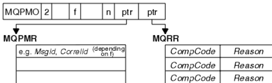
Abbildung 64. Nachricht in C in eine Verteilerliste einreihen
