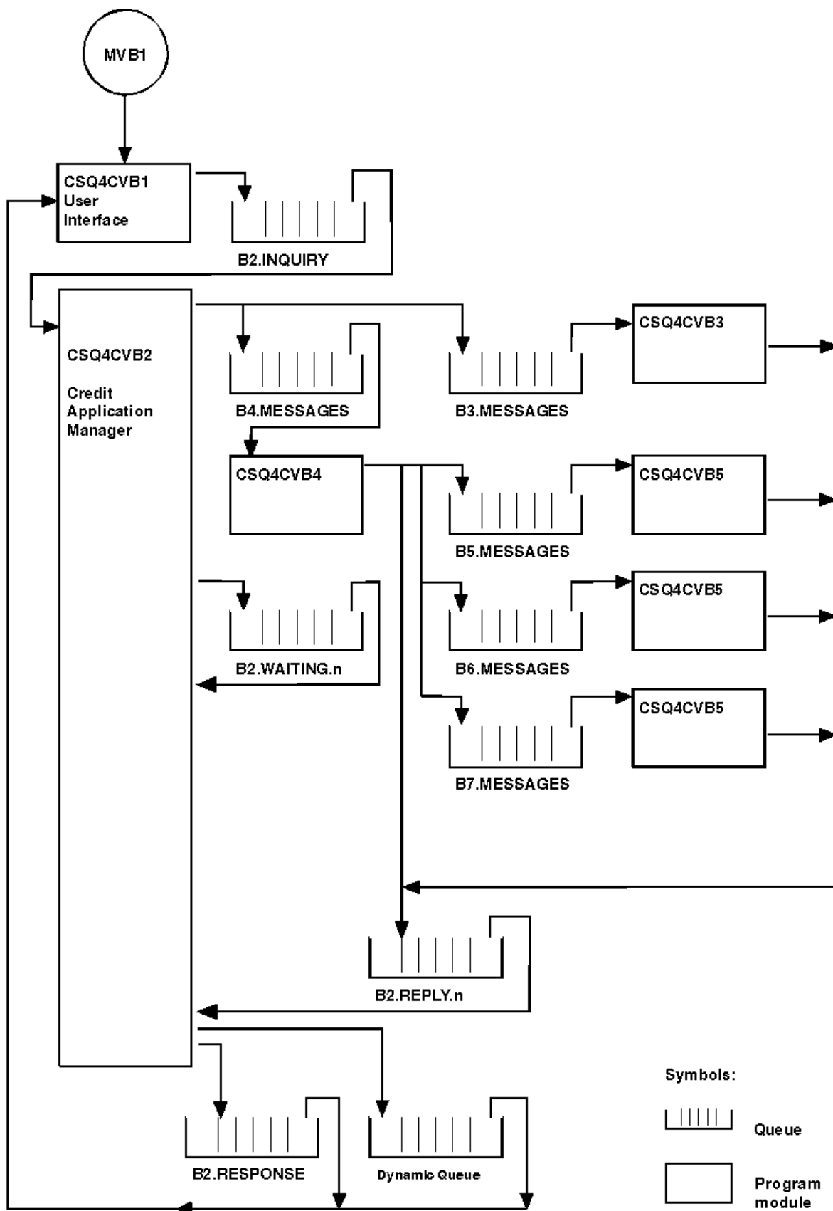
Abbildung 152. Programme und Warteschlangen für die Beispielanwendung zur Prüfung der Kreditwürdigkeit (nur COBOL-Programme)
