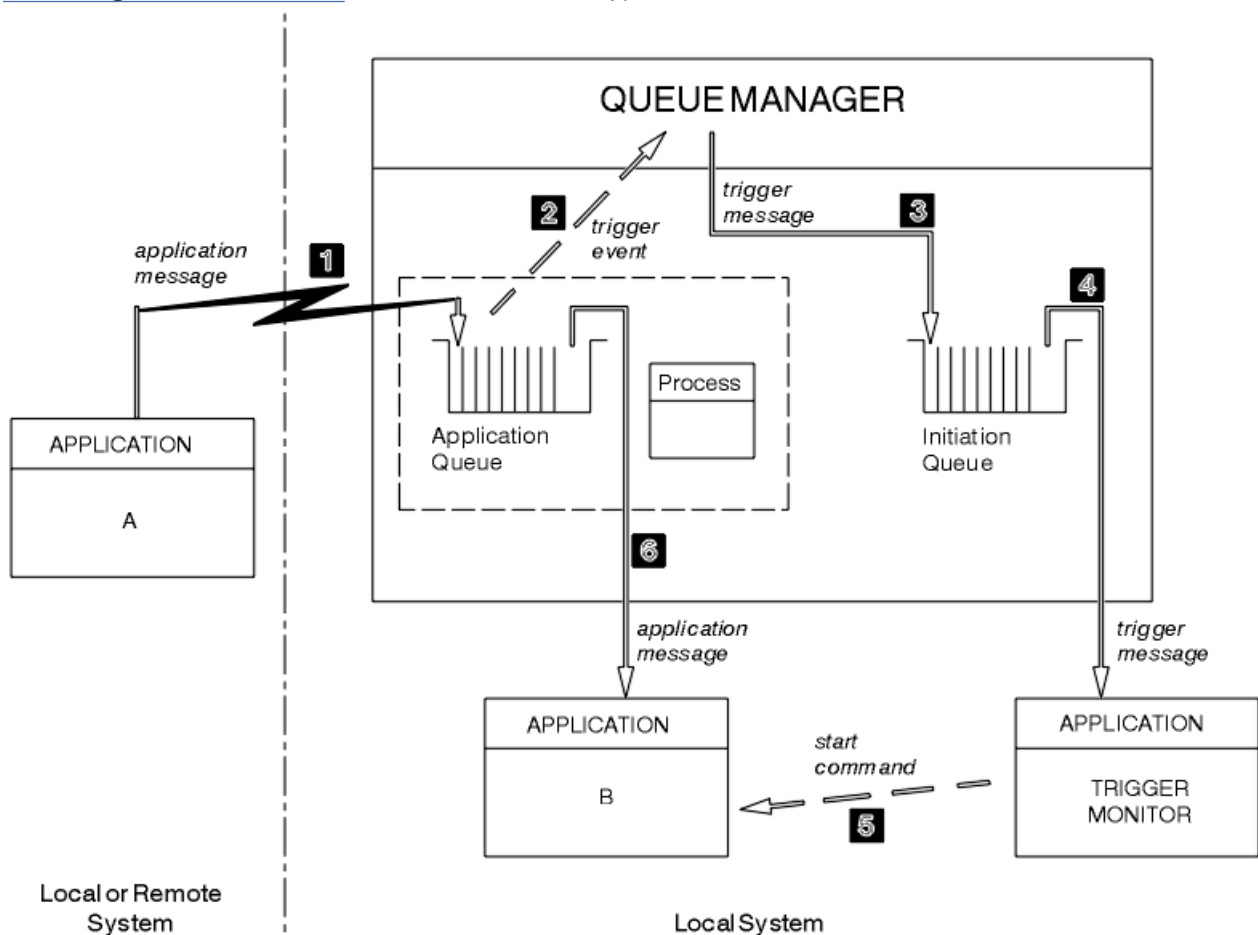
Abbildung 100. Ablauf von Anwendungs- und Auslösenachrichten
