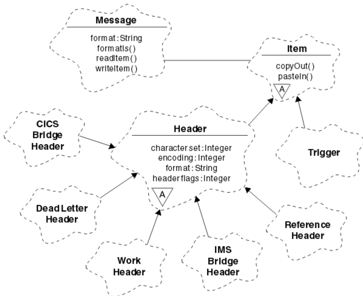
Abbildung 58. IBM MQ C++-Klassen (Behandlung von Elementen)
