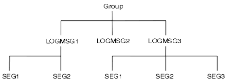
Abbildung 8. Segmentierte Nachrichten
