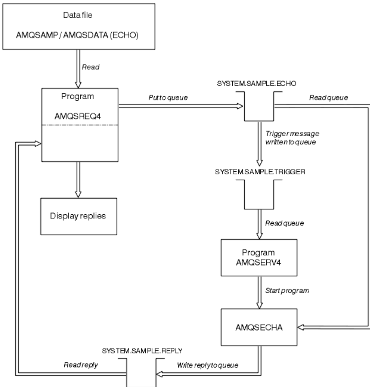
Abbildung 140. Ablaufdiagramm des IBM i Client/Server (Echo)-Beispielprogramms
