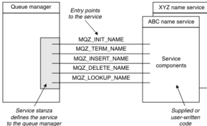
Abbildung 104. Zusammenhang zwischen Services, Komponenten und Eingangspunkten
