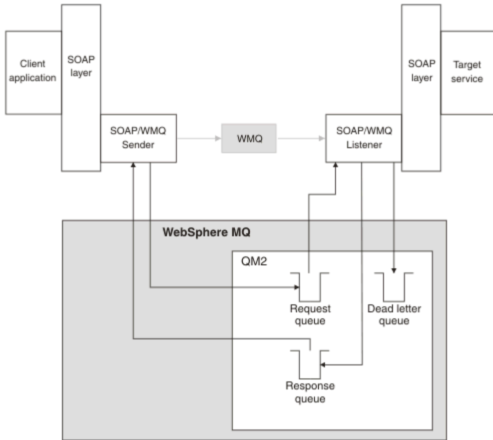
Abbildung 160. Von SOAP/IBM MQ verwendete Warteschlangen (einzelner Warteschlangenmanager)
