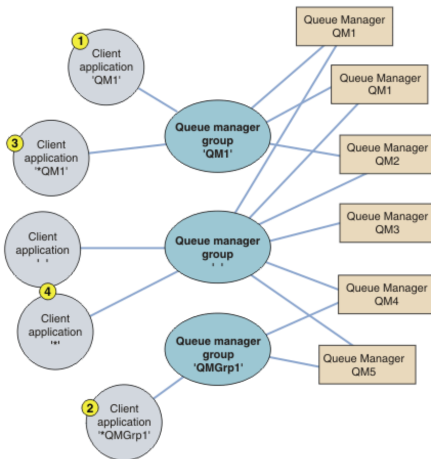
Abbildung 102. WS-Manager-Gruppen
