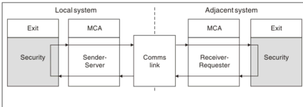
Abbildung 110. Sicherheitsexitschleife
