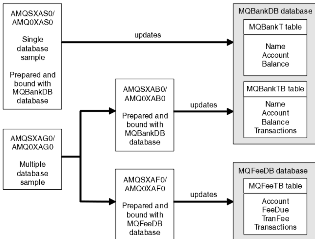
Obrázek 135. Ukázky koordinace databází
