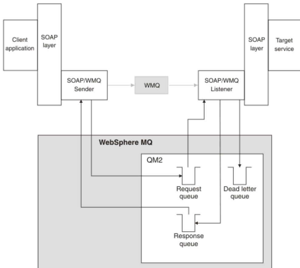
Obrázek 160. Fronty použité SOAP/IBM MQ (jednotlivý správce front)
