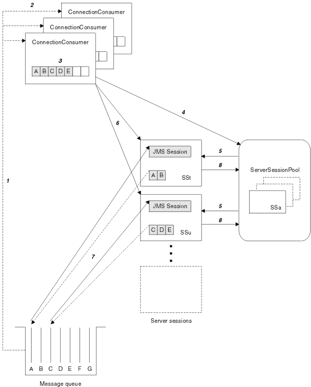
Obrázek 53. Funkčnost ServerSessionPool a ServerSession
