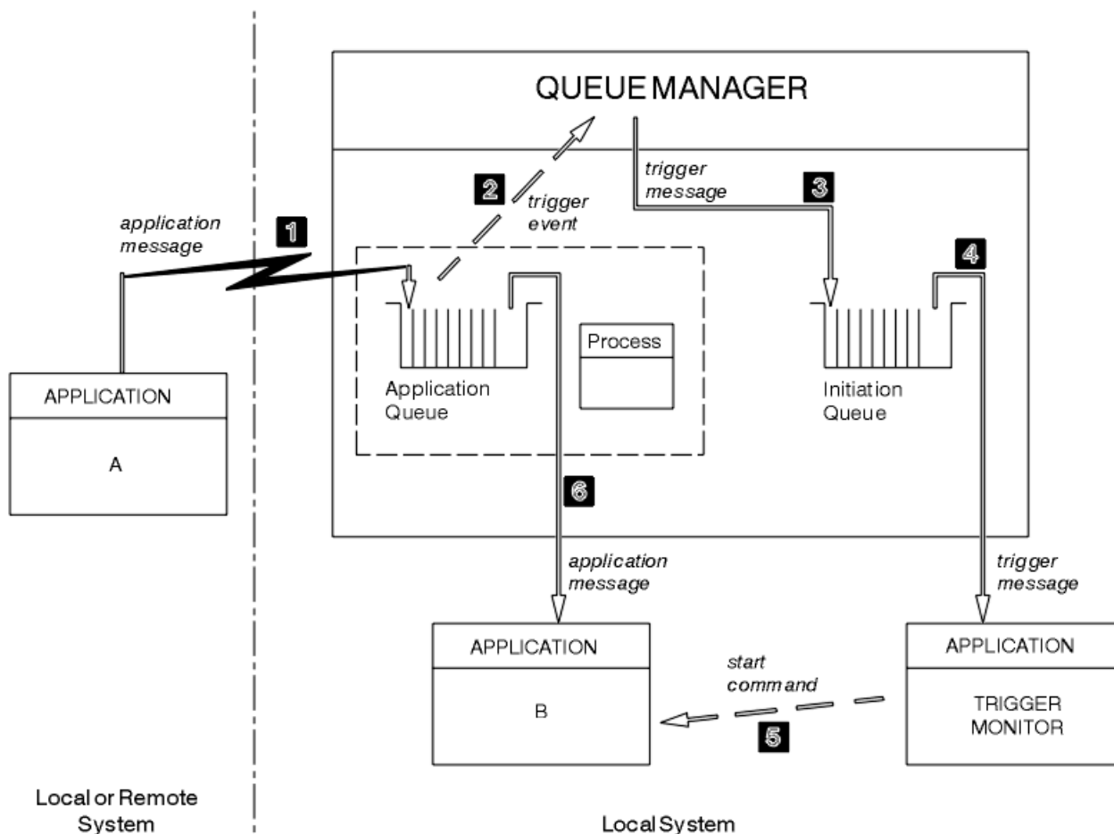
Obrázek 100. Tok zpráv aplikace a spouštěče
