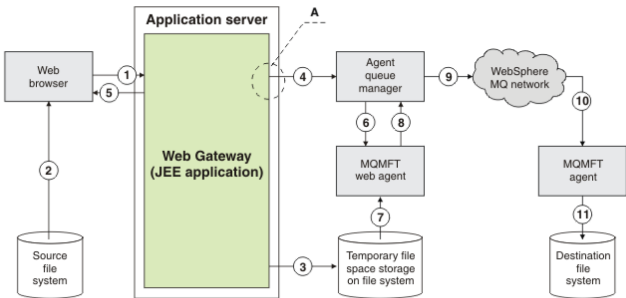
圖 4: 透過 Web 閘道上傳的檔案所涉及的 WebSphere MQ Managed File Transfer 元件
