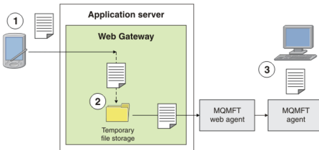
圖 1: 使用 Web 閘道將檔案上傳至 IBM WebSphere MQ Managed File Transfer 網路
