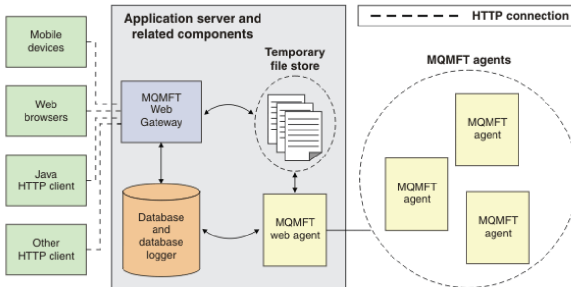
圖 3: Web 閘道架構的概觀
