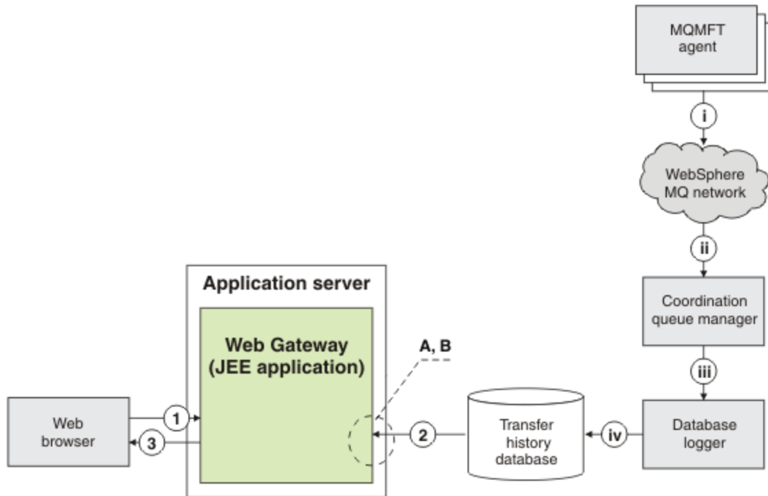
圖 6: 透過 Web 閘道要求檔案傳送的状态
