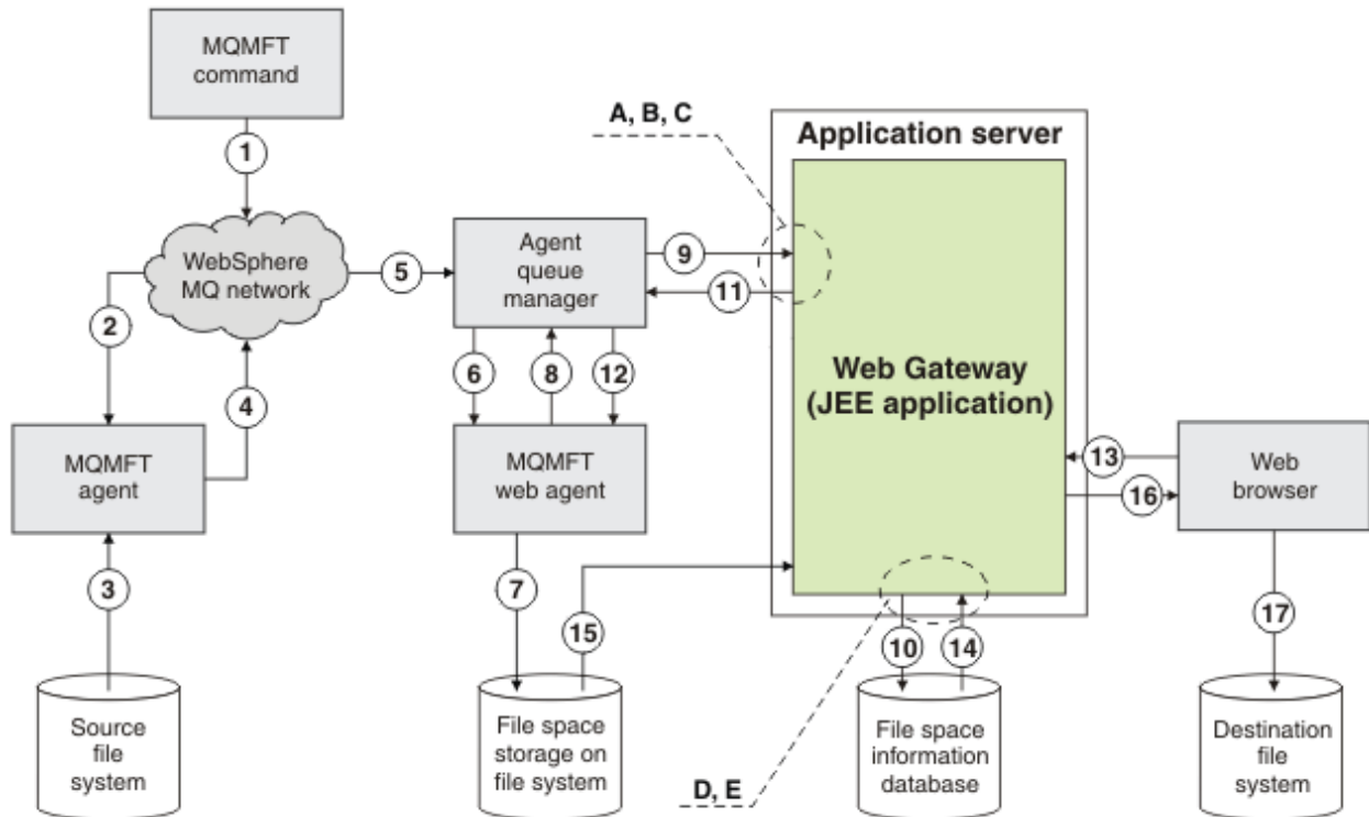
圖 5: 檔案上傳至檔案空間以及後續從檔案空間下載所涉及的 IBM WebSphere MQ Managed File Transfer 元件
