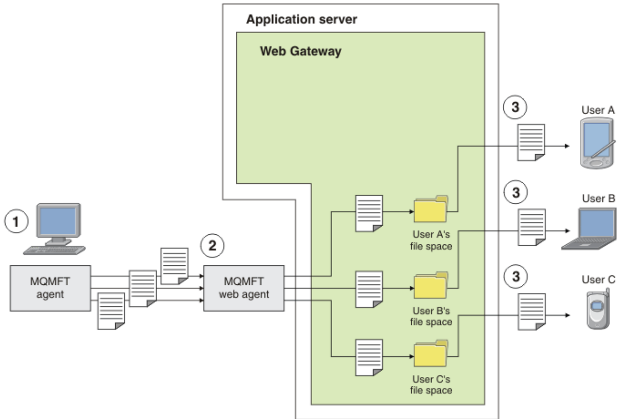
圖 2: 使用 Web 閘道從檔案空間下載檔案
