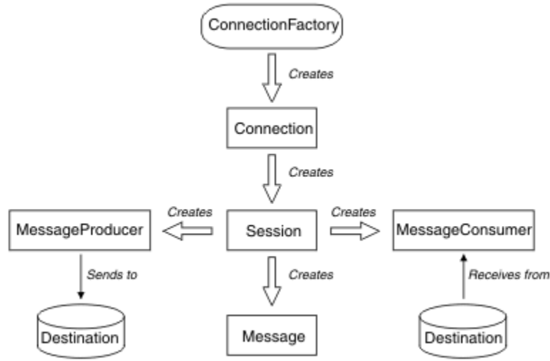
Şekil 1. XMS nesneleri ve ilişkileri
