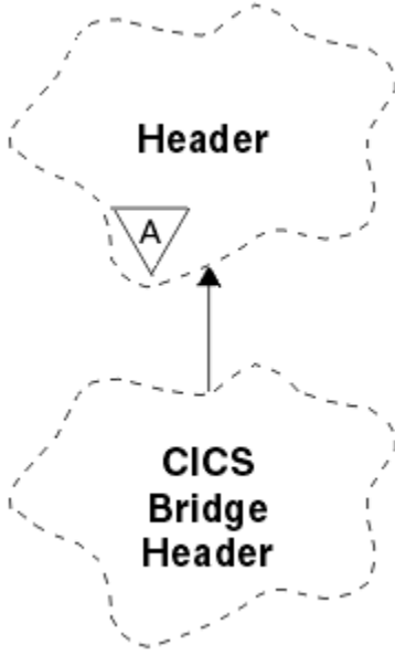
Şekil 50. ImqCICSBridgeÜstbilgi sınıfı
