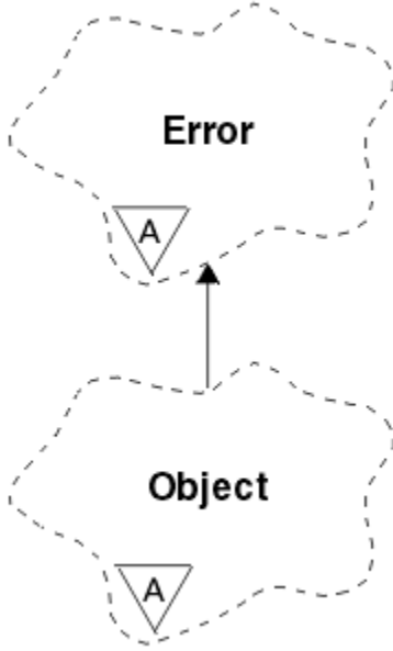
Şekil 61. ImqObject sınıfı
