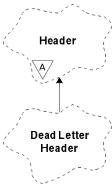
Şekil 51. ImqDeadLetterHeader sınıfı
