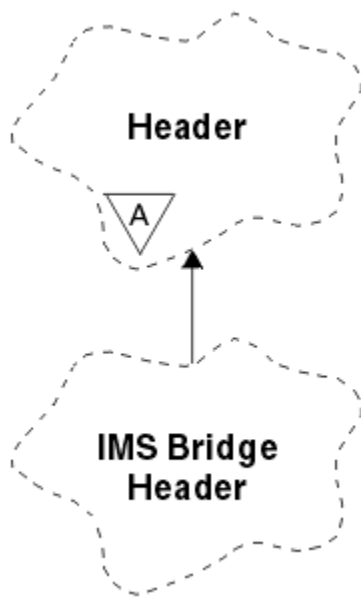
図 23. ImqIMSBridgeHeader クラス
