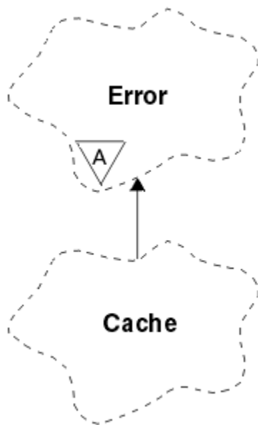
図 15. ImqCache クラス
