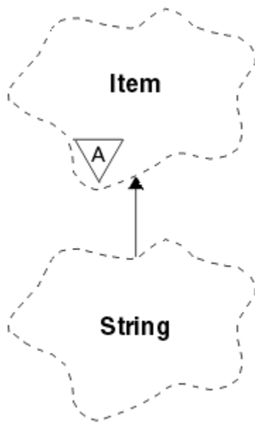
図 34. ImqString クラス
