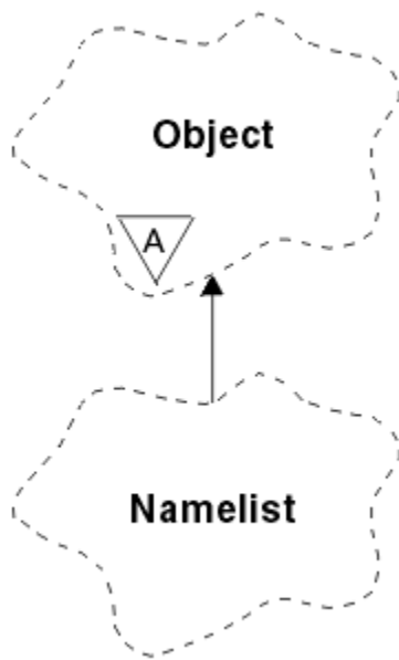
図 27. ImqNamelist クラス
