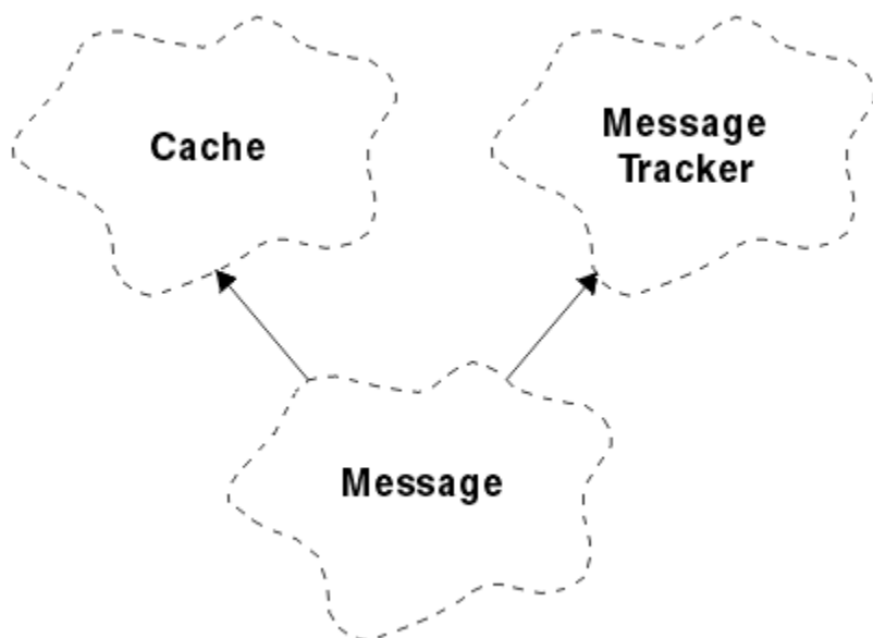
図 25. ImqMessage クラス
