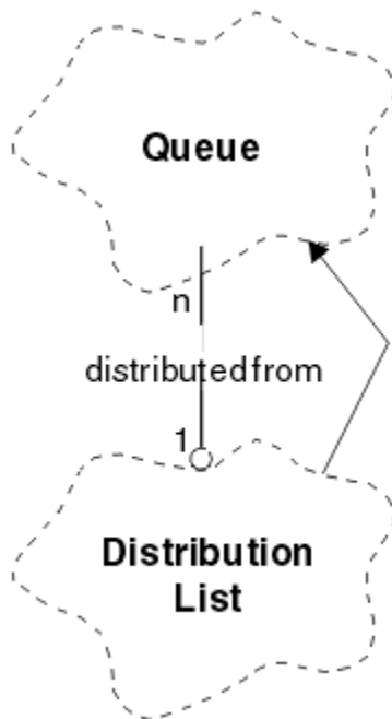
図 19. ImqDistributionList クラス
