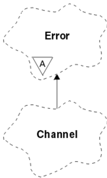
図 16. ImqChannel クラス
