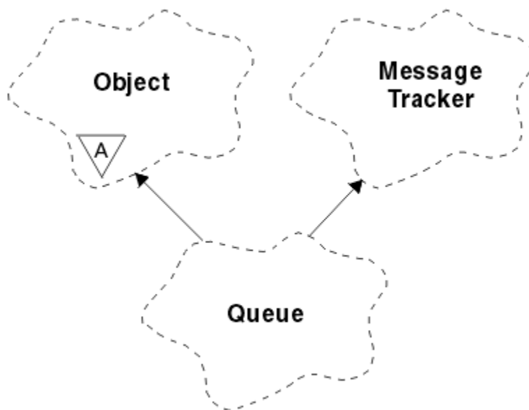
図 31. ImqQueue クラス
