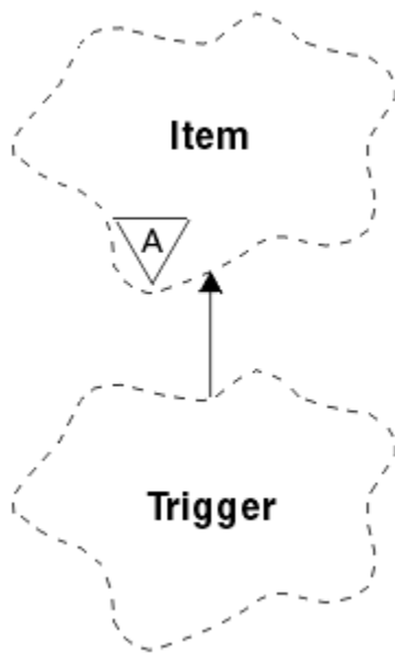
図 35. ImqTrigger クラス
