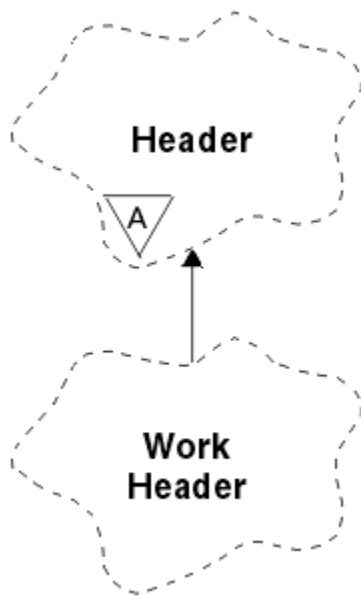
図 36. ImqWorkHeader クラス
