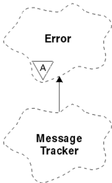
図 26. ImqMessageTracker クラス
