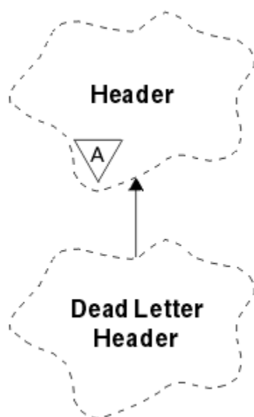
図 18. ImqDeadLetterHeader クラス
