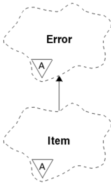
図 24. ImqItem クラス
