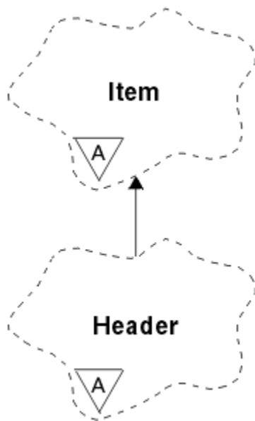
図 22. ImqHeader クラス
