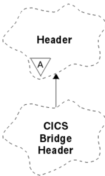
図 17. ImqCICSBridgeHeader クラス
