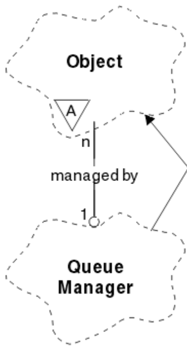
図 32. ImqQueueManager クラス
