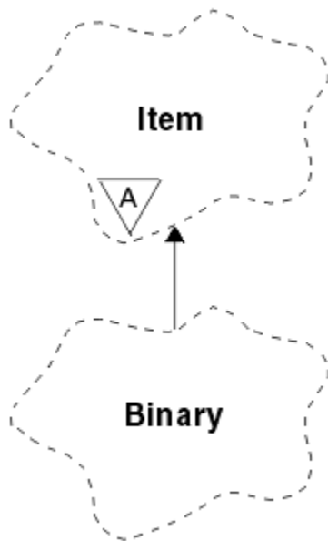
図 14. ImqBinary クラス
