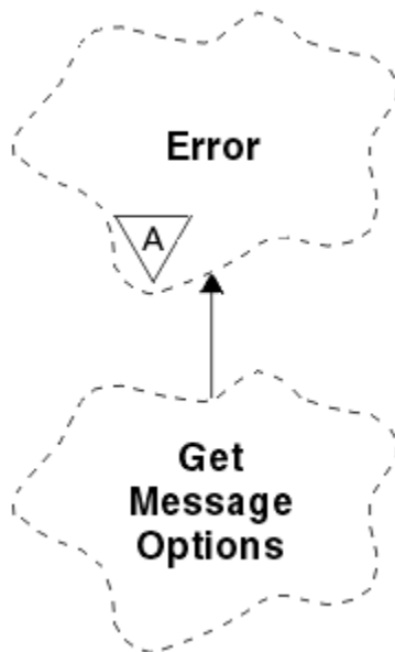
図 21. ImqGetMessageOptions クラス
