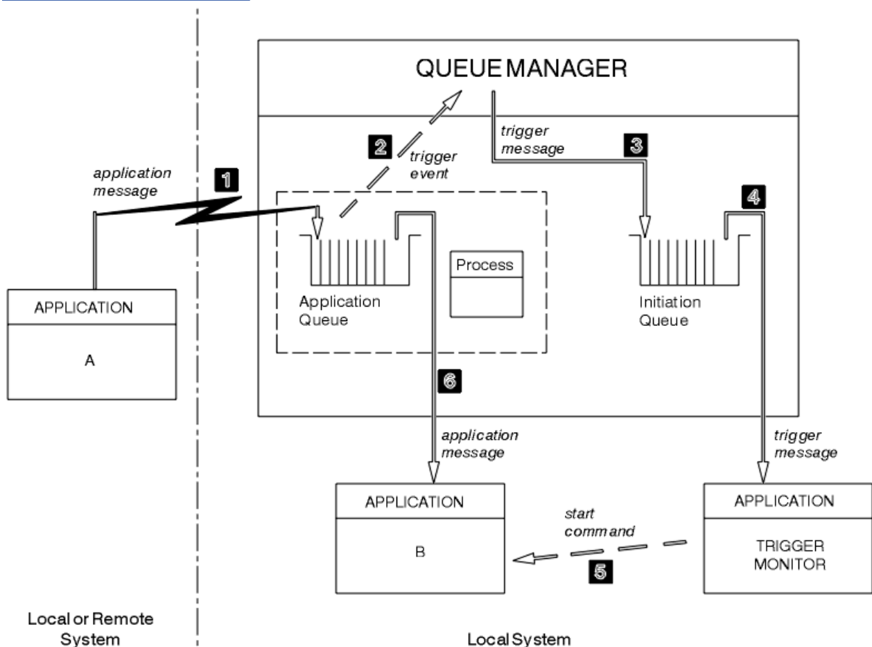
Abbildung 125. Ablauf von Anwendungs- und Auslösenachrichten
