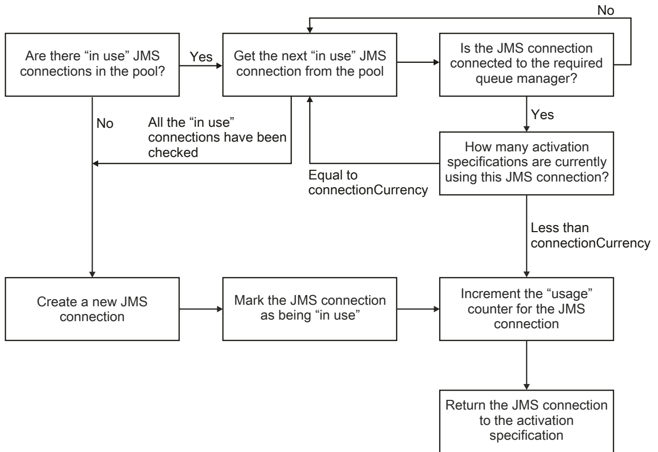
Abbildung 43. WebSphere Application Server V7.5 und V8.0 - Funktionsweise des Verbindungspools
