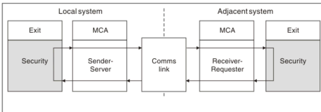
Abbildung 76. Sicherheitsexitschleife
