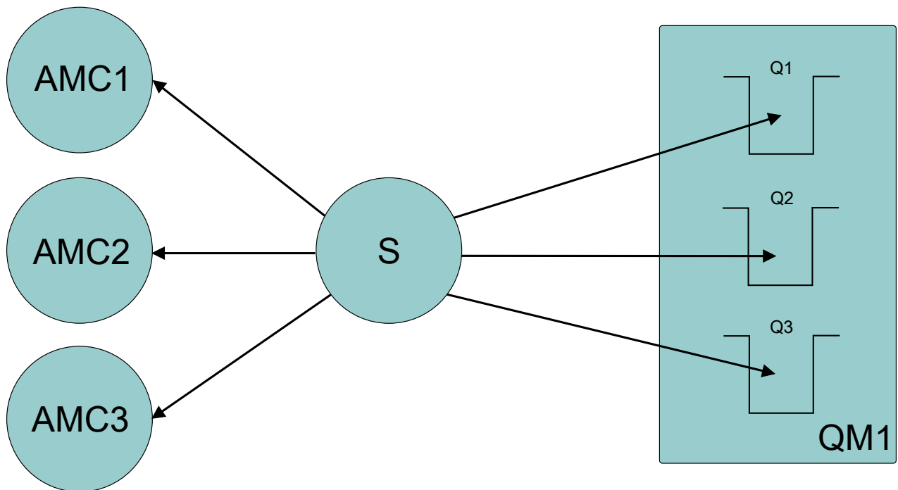
Abbildung 70. Eine Sitzung mit drei asynchronen Nachrichtenkonsumenten
