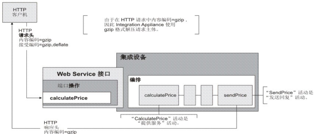
图 1. HTTP 请求
