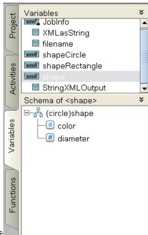
图 3. 变量选项卡
