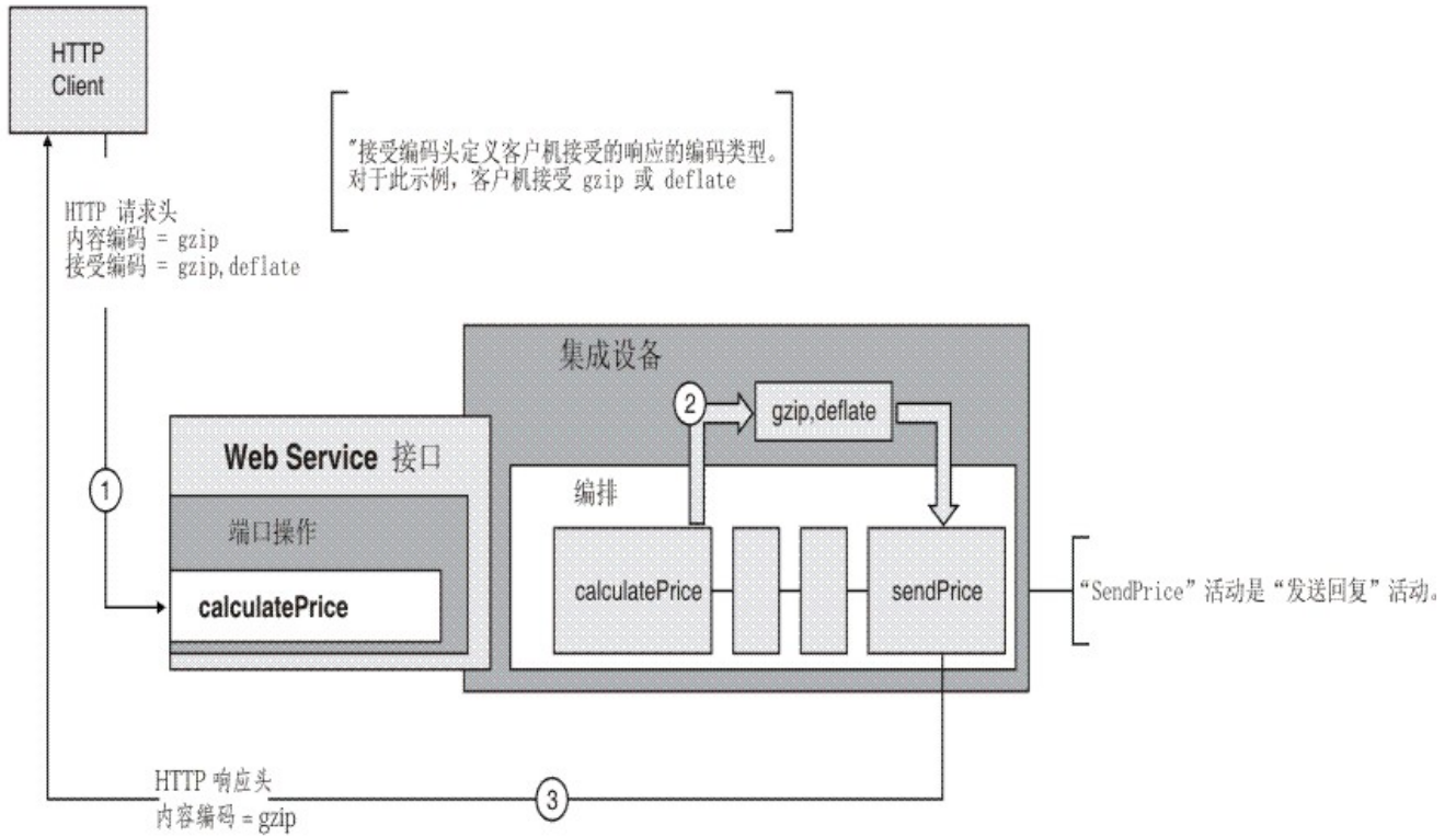
图 1. 接受编码头
