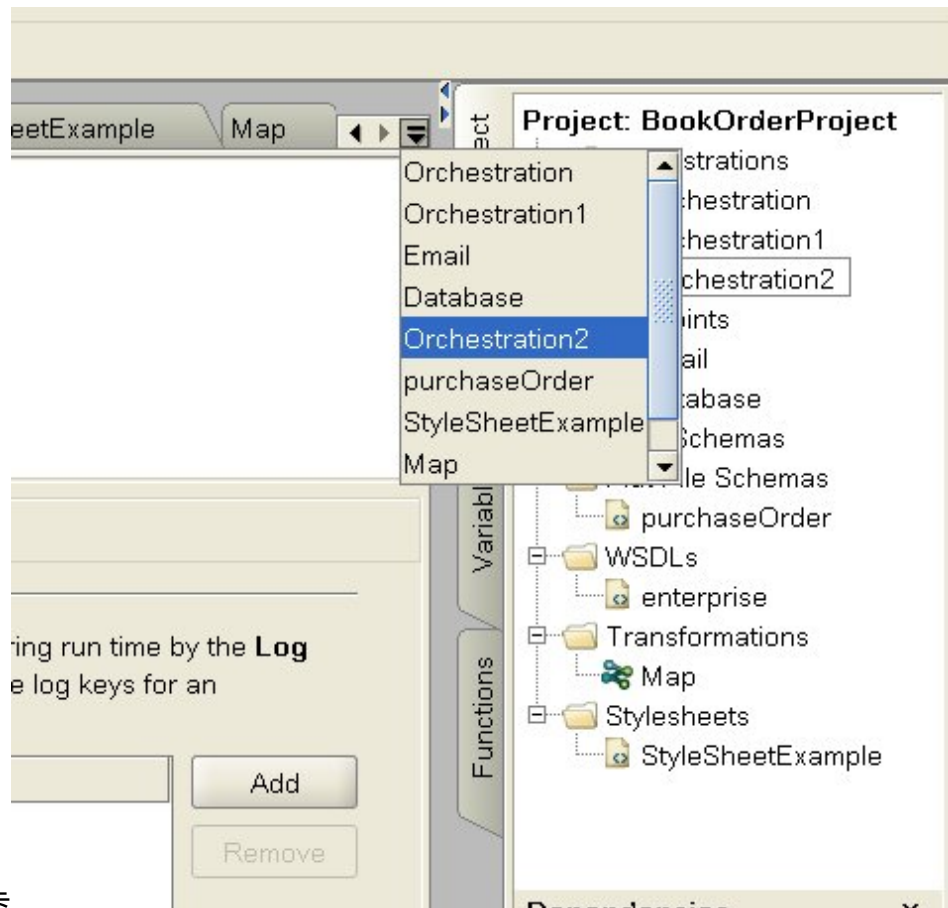
图 2. 隐藏选项卡
