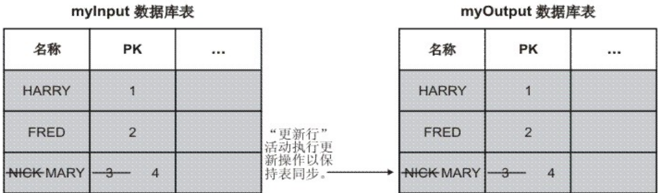
图 3. 示例 2
