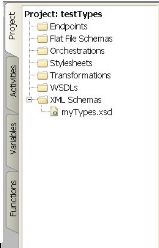
图 3. 示例
