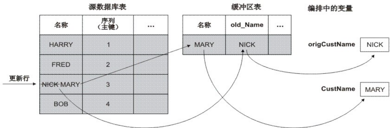
图 1. 更新旧列
