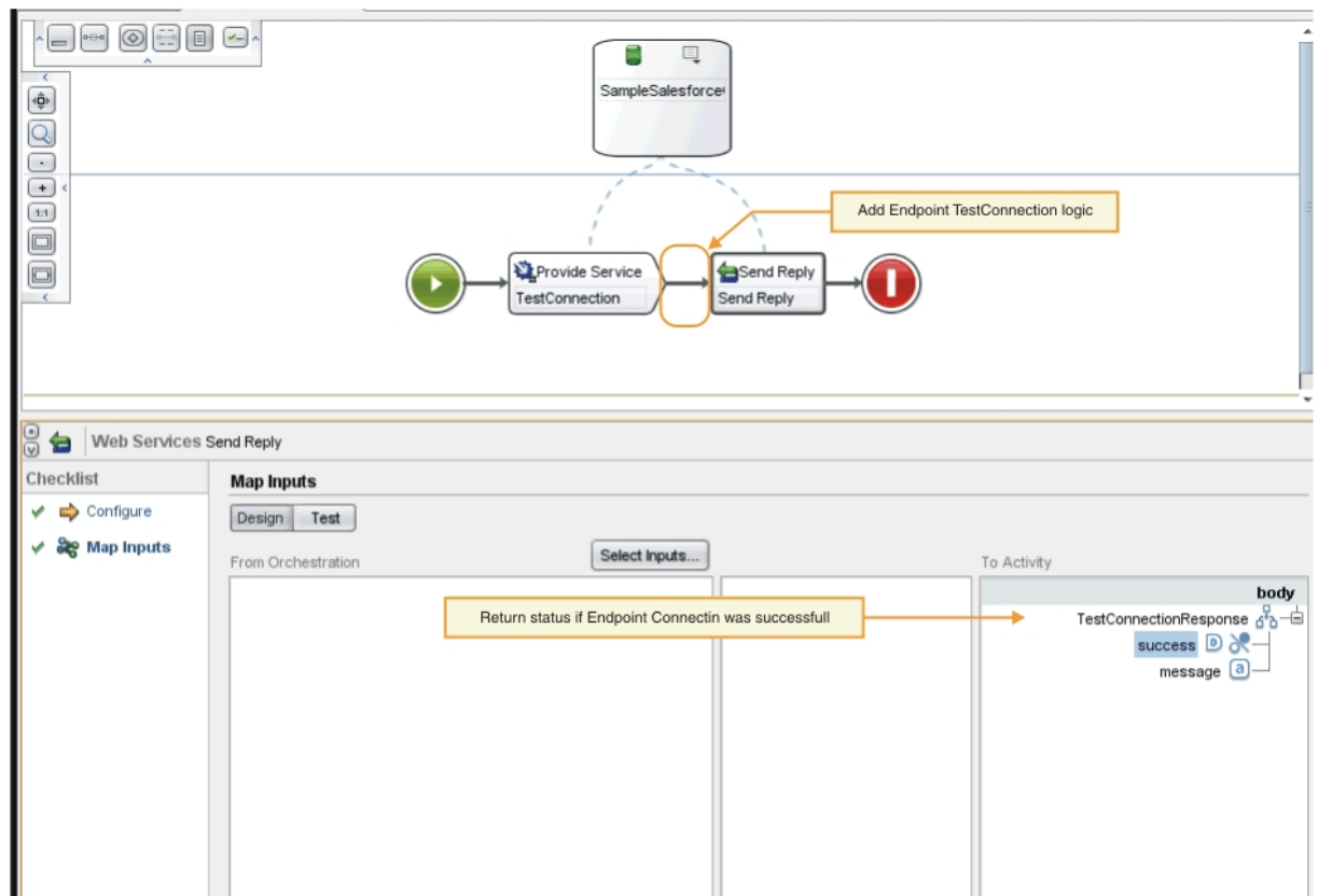
图 1. TestConnection
