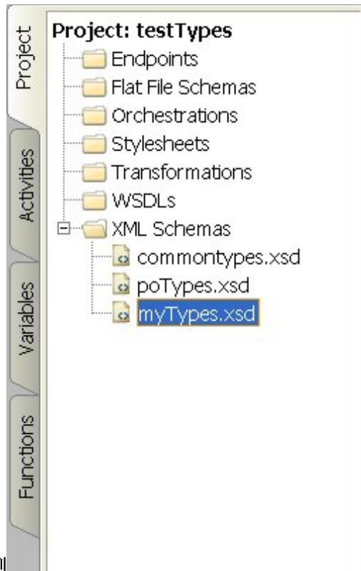
图 4. 示例
