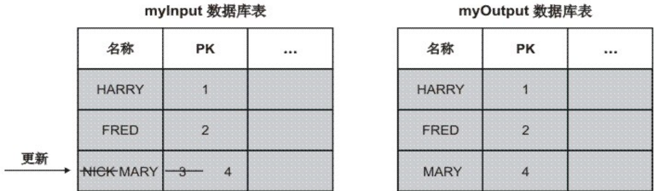
图 2. 示例 1
