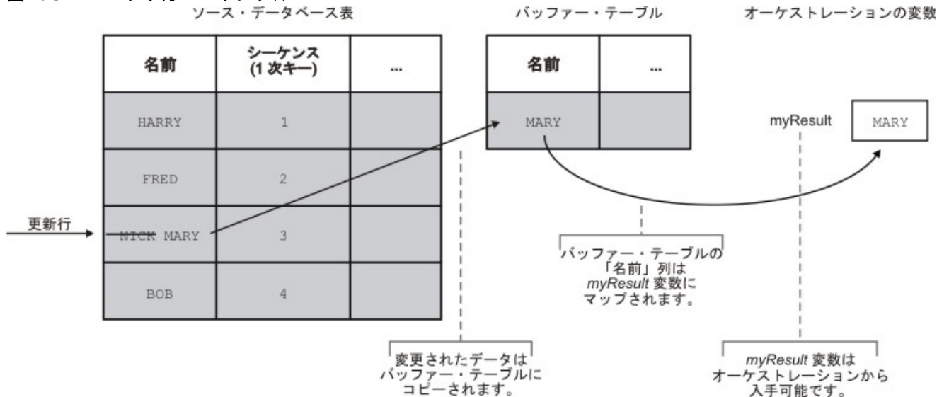
図 1. UPDATE トリガー・サンプル
