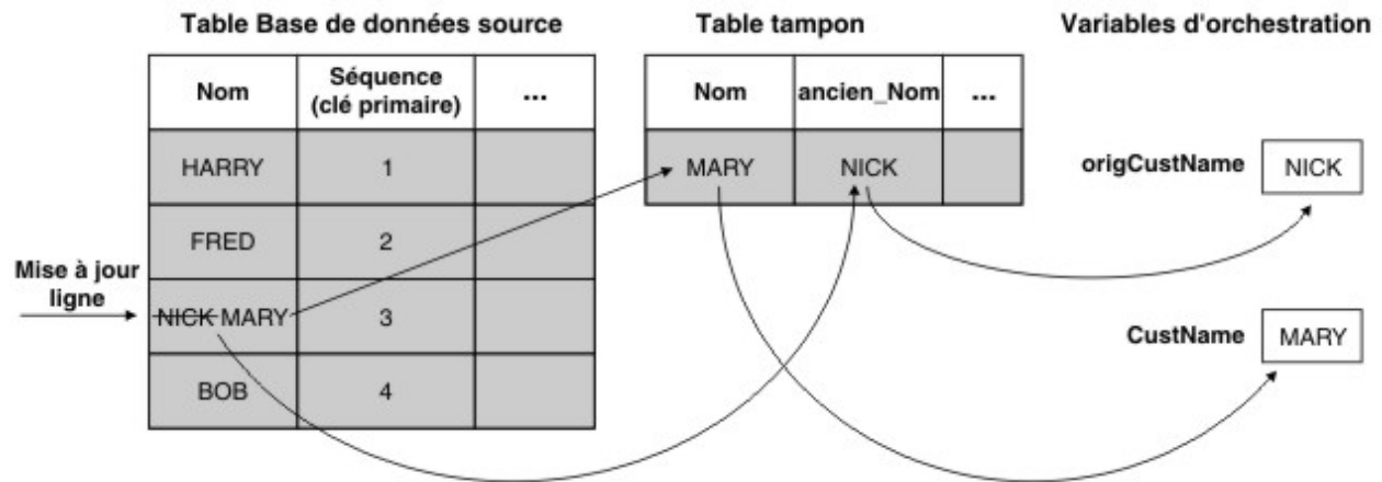
Figure 1. Mettre à jour les colonnes d'anciennes valeurs
