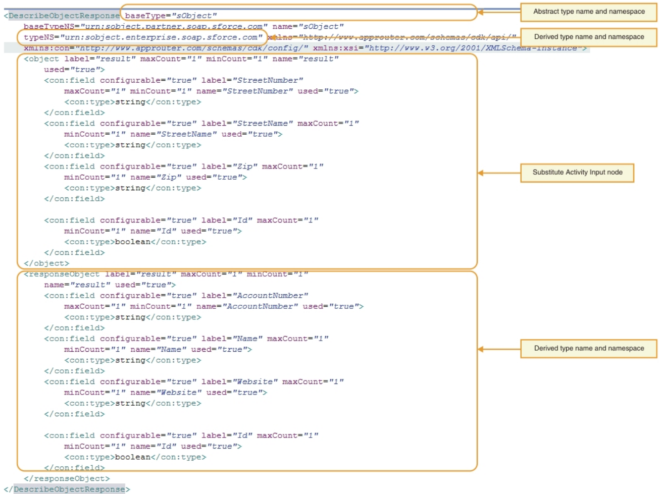
Figure 1. Fichier WSDL avec définition abstraite
