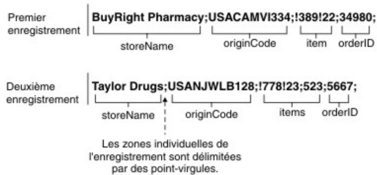
Figure 3. Exemple de combinaison 2 : Les zones individuelles de l'enregistrement sont délimitées par
