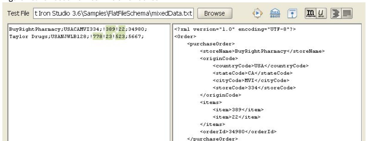
Figure 10. Le noeud item est mis en évidence
