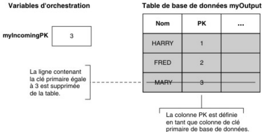
Figure 2. La ligne contenant la clé primaire égale à 3 est supprimée
