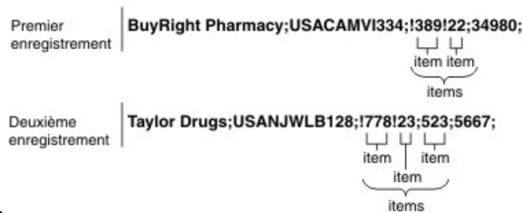
Figure 7. Exemple de combinaison 5 où les données délimitées sont indiquées par des points
