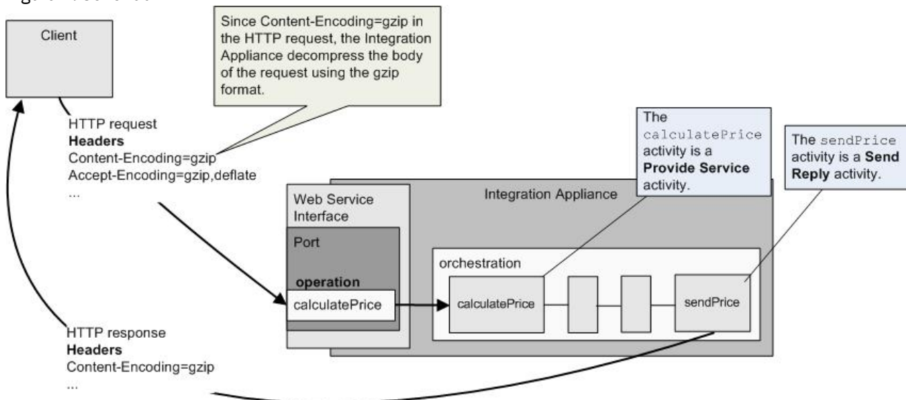
Figura 1. Solicitud HTTP
