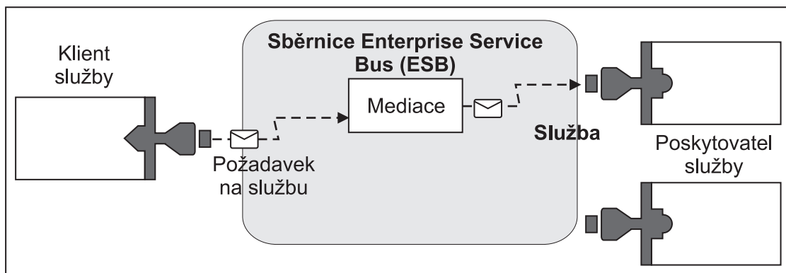
Obrázek 87. Sběrnice Enterprise Service Bus. Sběrnice Enterprise Service Bus trasuje zprávy mezi aplikacemi, které jsou žadateli nebo poskytovateli služeb. Sběrnice převádí přenosové protokoly a transformuje formát zpráv mezi žadatelem a poskytovateli. Na tomto obrázku používá každá aplikace jiný protokol (reprezentovaný jiným geometrickým tvarem konektoru) a jiný formát zpráv.
