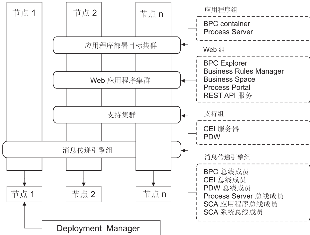
图 7. “远程消息传递、远程支持和 Web”拓扑模式
