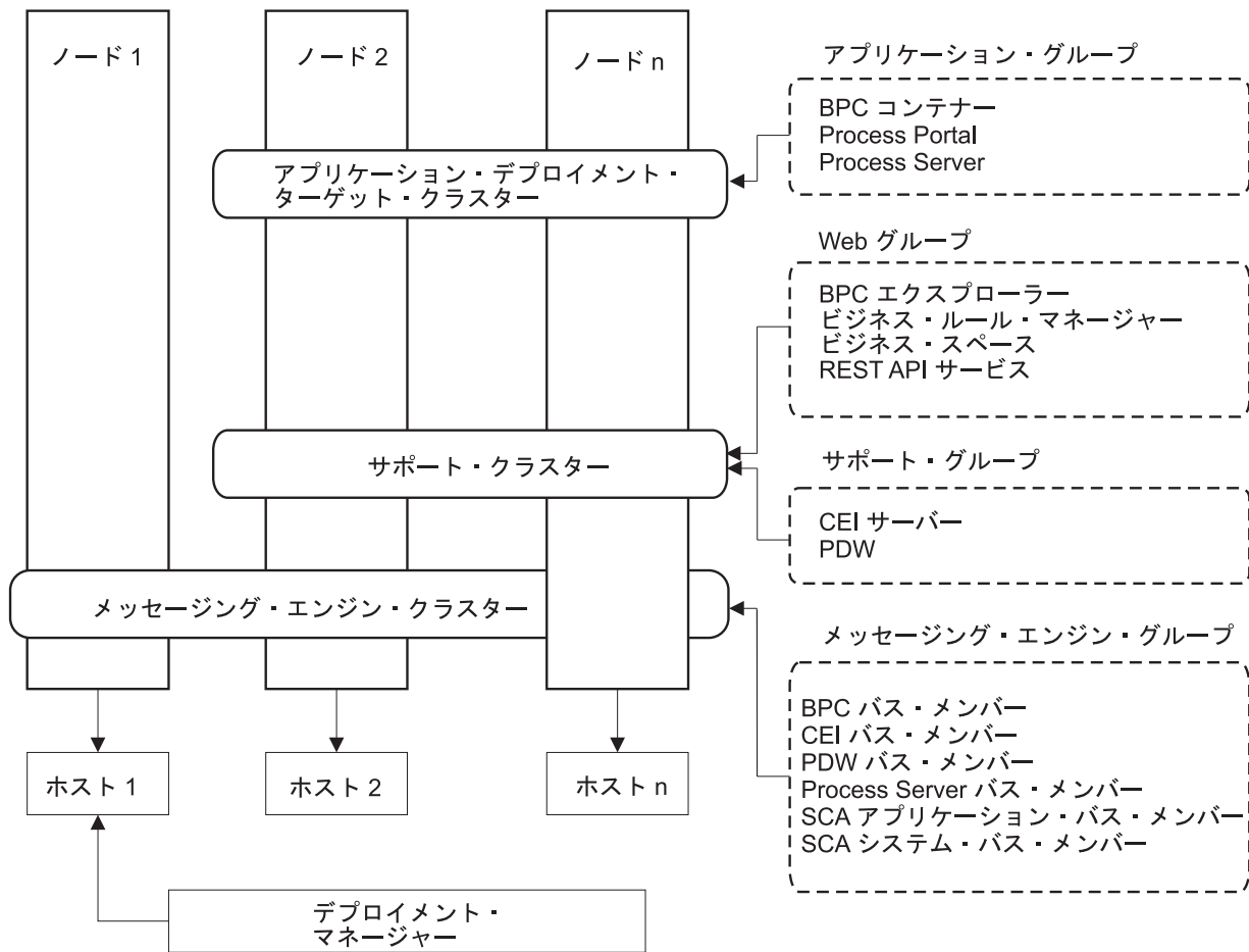
図5. リモート・メッセージングおよびリモート・サポート・トポロジー・パターン
