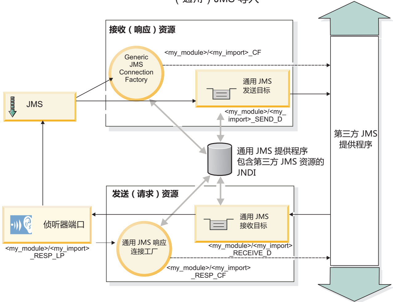
图 80. 通用 JMS 导入绑定资源
