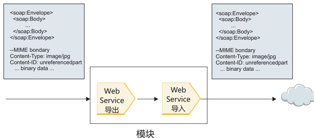
图 68. 通过 SCA 模块传递的附件
