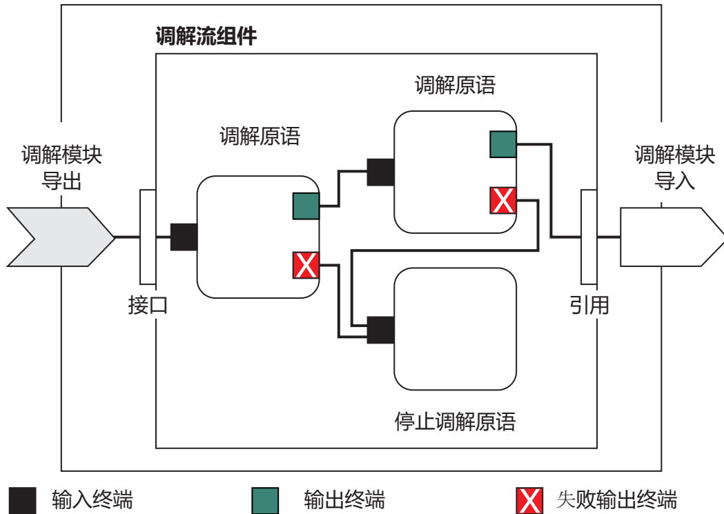
图 43. 调解模块的简单示例. 调解模块中包含一个调解流组件, 该调解流组件中包含调解原语。
