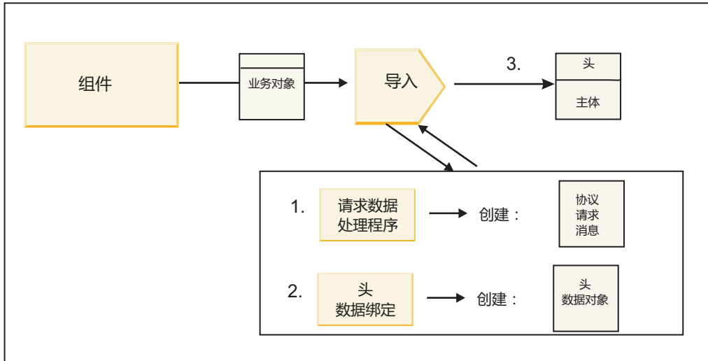
图 50. 从组件通过导入到服务的流
