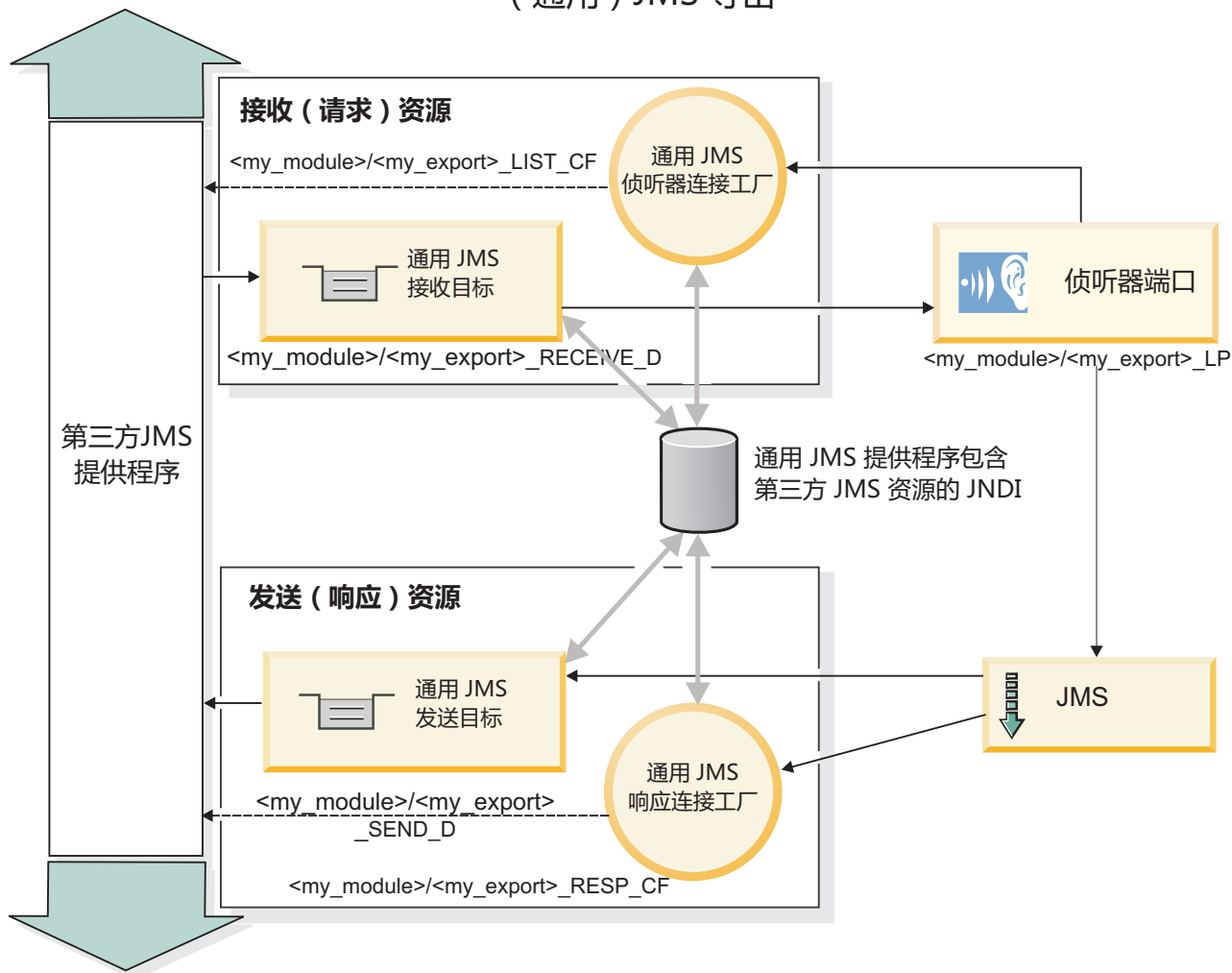
图 81. 通用 JMS 导出绑定资源
