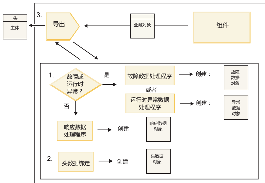
图 49. 通过导出返回的响应流
