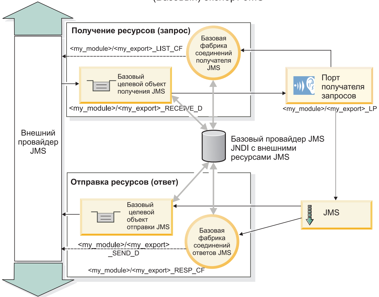
Рисунок 81. Ресурсы базовых привязок экспортов JMS
