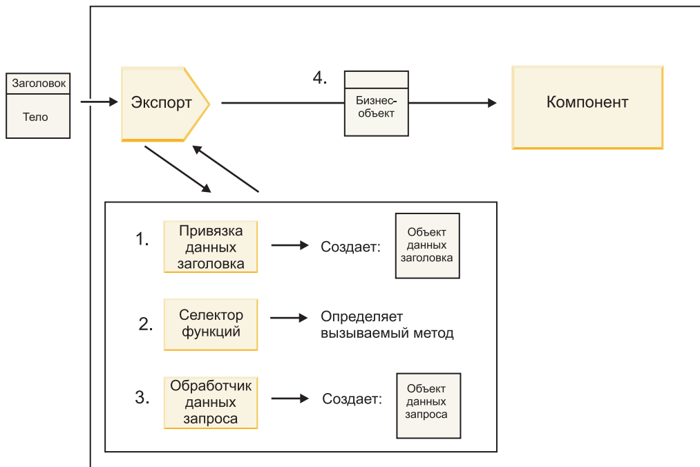
Рисунок 3. Передача запроса в компонент через объект экспорта
