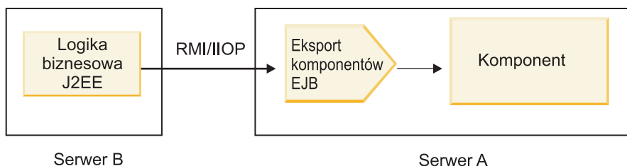
Rysunek 30. Zdalne wywołanie z klienta do komponentu SCA za pośrednictwem eksportu EJB
