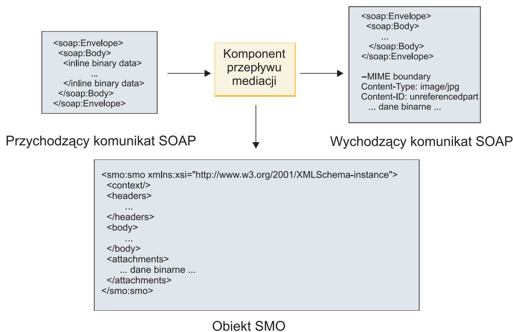
Rysunek 24. Komunikat przetworzony przez komponent przepływu mediacji
