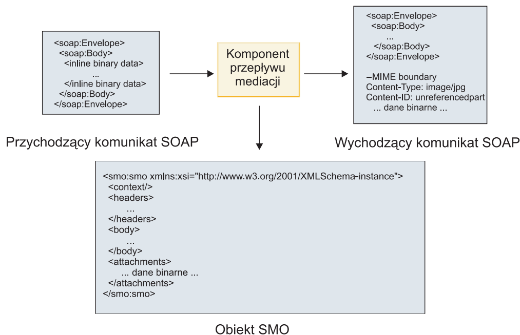
Rysunek 69. Komunikat przetworzony przez komponent przepływu mediacji
