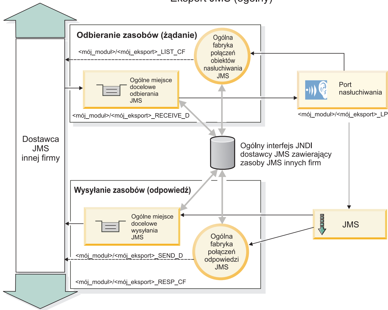
Rysunek 81. Zasoby ogólnego powiązania eksportu JMS
