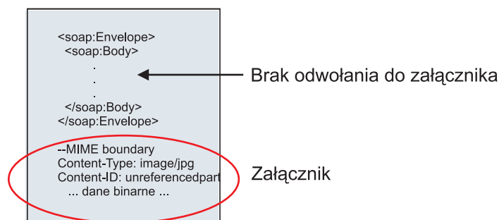
Rysunek 22. Komunikat SOAP z załącznikiem nieprzywoływanym
