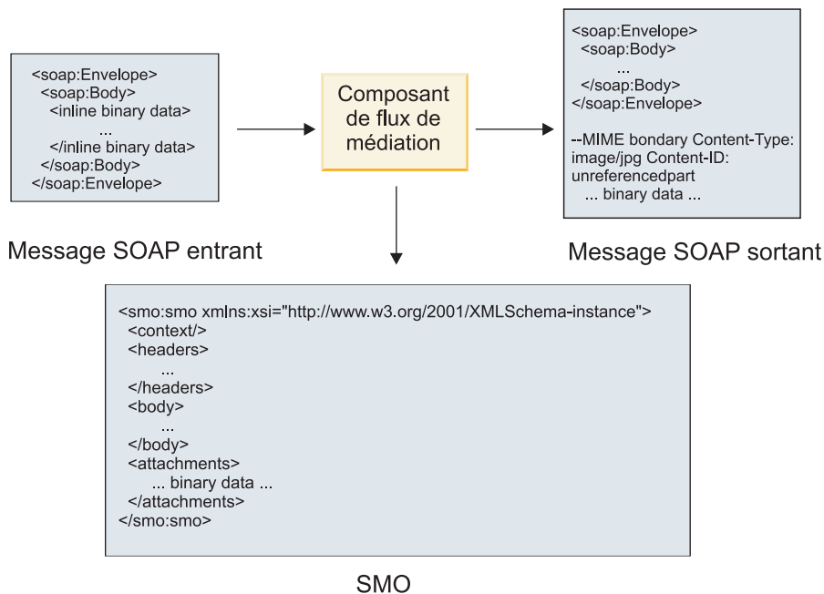
Figure 69. Message traité par un composant de flux de médiation
