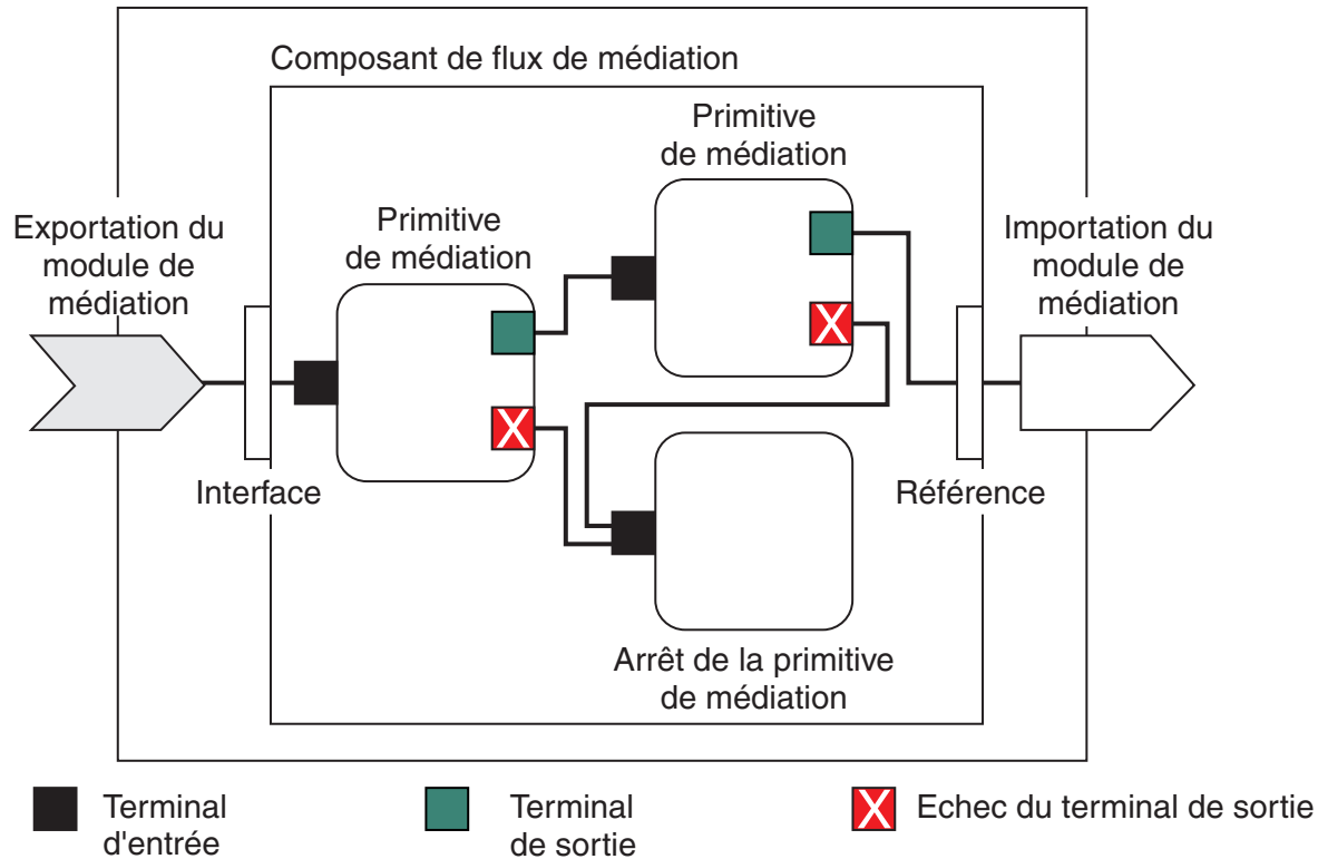
Figure 88. Exemple simplifié d'un module de médiation. Le module de médiation contient un composant de flux de médiation, qui contient des primitives de médiation.
