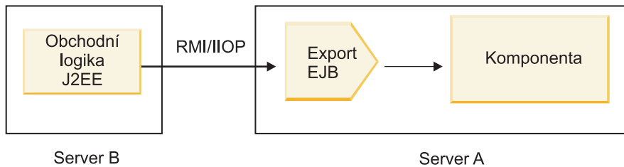
Obrázek 75. Vzdálené volání z klienta do komponenty SCA prostřednictvím exportu EJB
