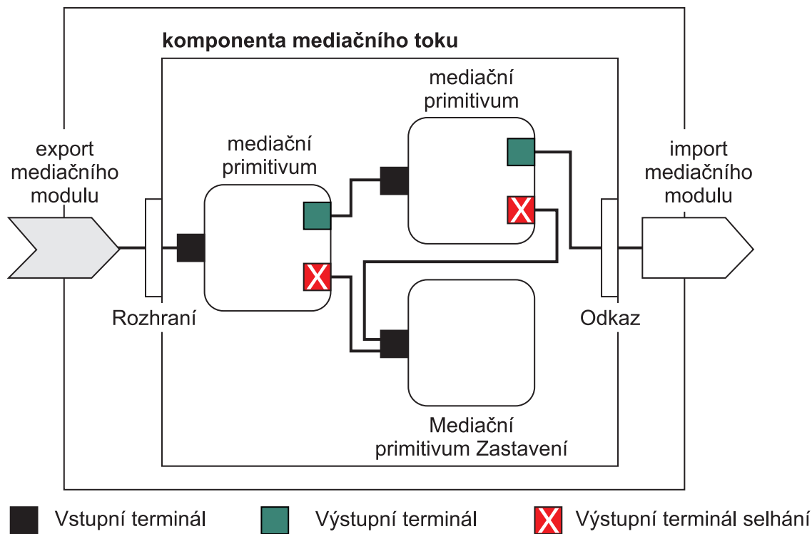
Obrázek 88. Zjednodušený příklad mediálního modulu. Mediační modul obsahuje jednu komponentu mediálního toku, která obsahuje mediální primitiva.
