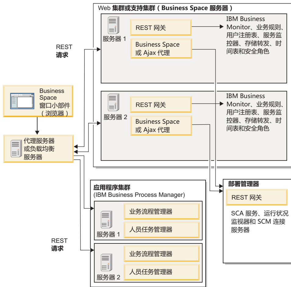
图 1. 典型拓扑
