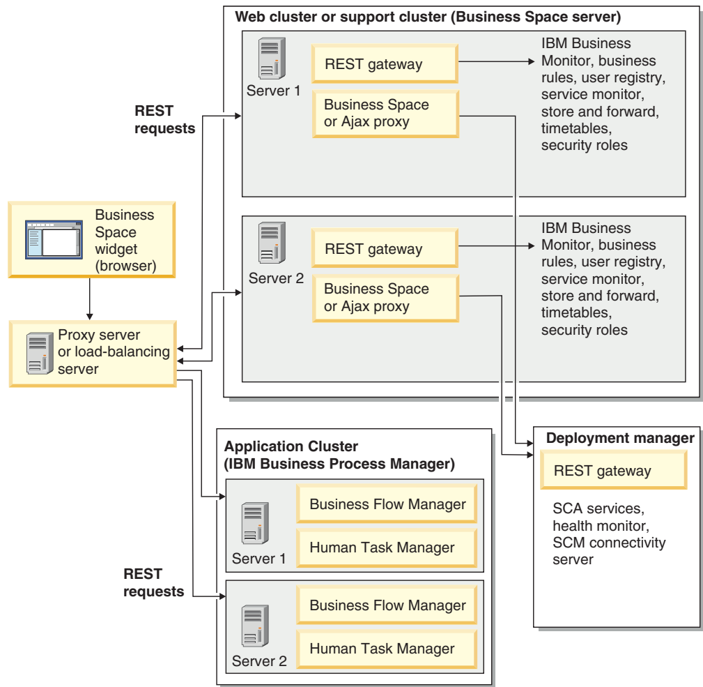
Figura 1. Topologia Típica
