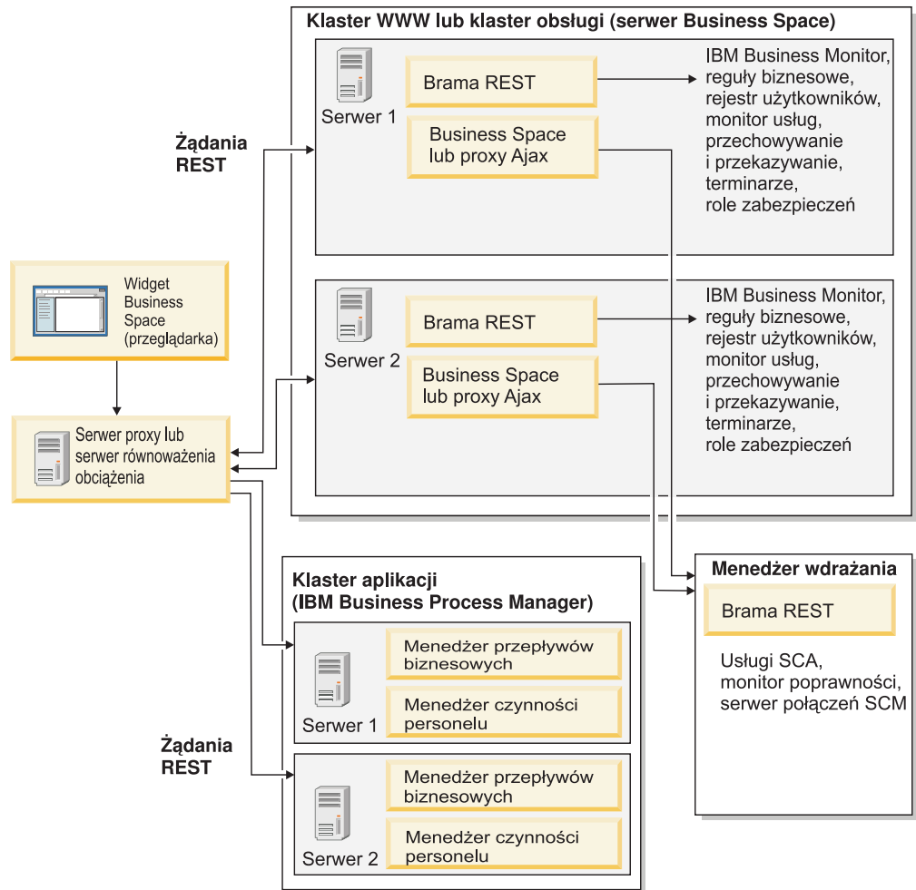
Rysunek 1. Typowa topologia
