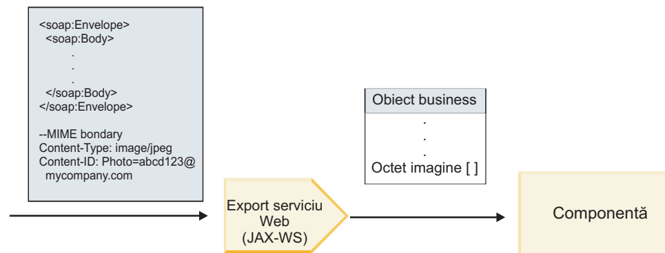
Figura 64. Modul în care legarea de export a serviciului Web (JAX-WS) procesează un mesaj SOAP conform cu WS-I ce are un atașament cu referință
