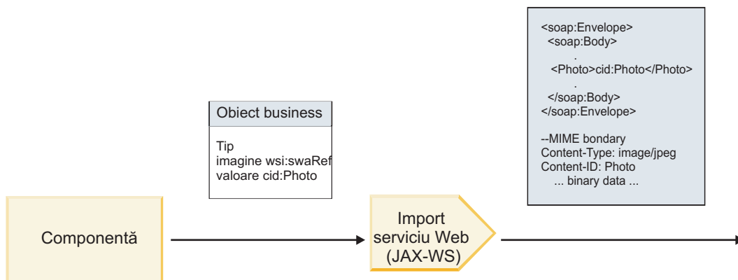
Figura 17. Modul în care legarea de import a serviciului Web (JAX-WS) generează un mesaj SOAP cu un atașament swaRef
