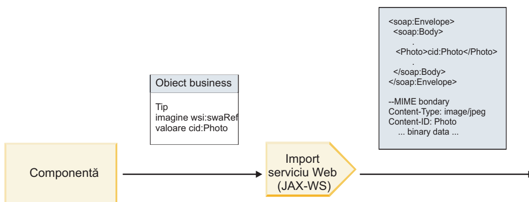
Figura 62. Modul în care legarea de import a serviciului Web (JAX-WS) generează un mesaj SOAP cu un atașament swaRef
