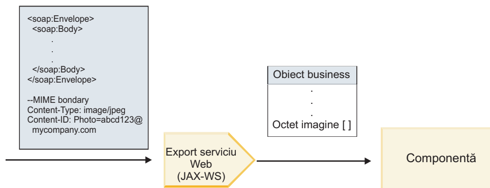
Figura 13. Cum procesează legarea de export a serviciului web (JAX-WS) un mesaj SOAP cu atașament cu referință
