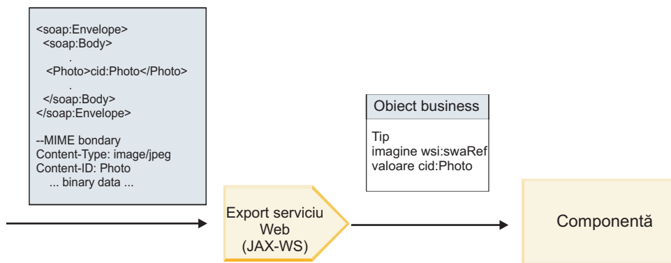
Figura 15. Modul în care legarea de export a serviciului Web (JAX-WS) procesează un mesaj de tip SOAP care conține un atașament de tip swaRef
