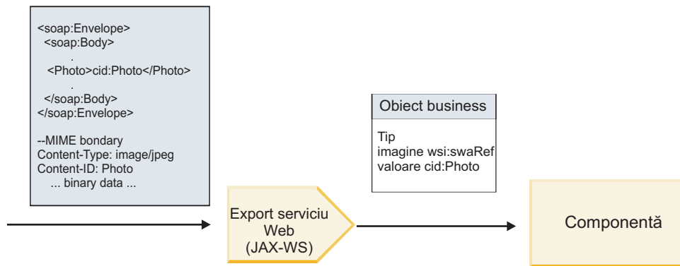
Figura 60. Modul în care legarea de export a serviciului Web (JAX-WS) procesează un mesaj de tip SOAP care conține un atașament de tip swaRef
