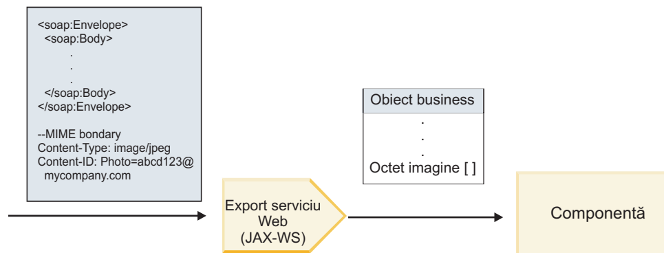
Figura 19. Modul în care legarea de export a serviciului Web (JAX-WS) procesează un mesaj SOAP conform cu WS-I ce are un atașament cu referință
