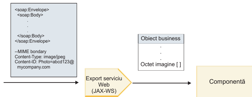
Figura 58. Cum procesează legarea de export a serviciului web (JAX-WS) un mesaj SOAP cu atașament cu referință
