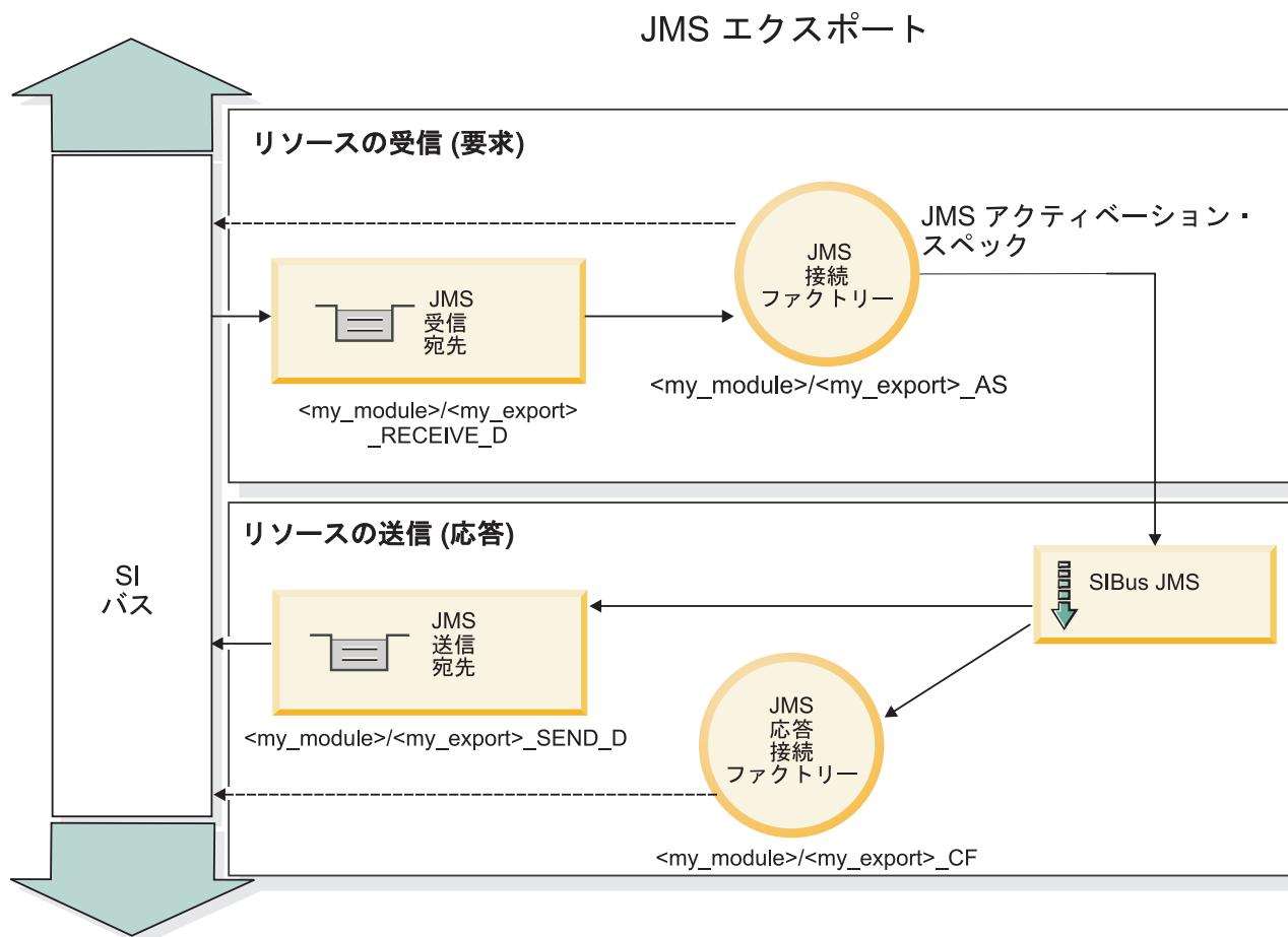
図 78. JMS エクスポート・バインディングのリソース
