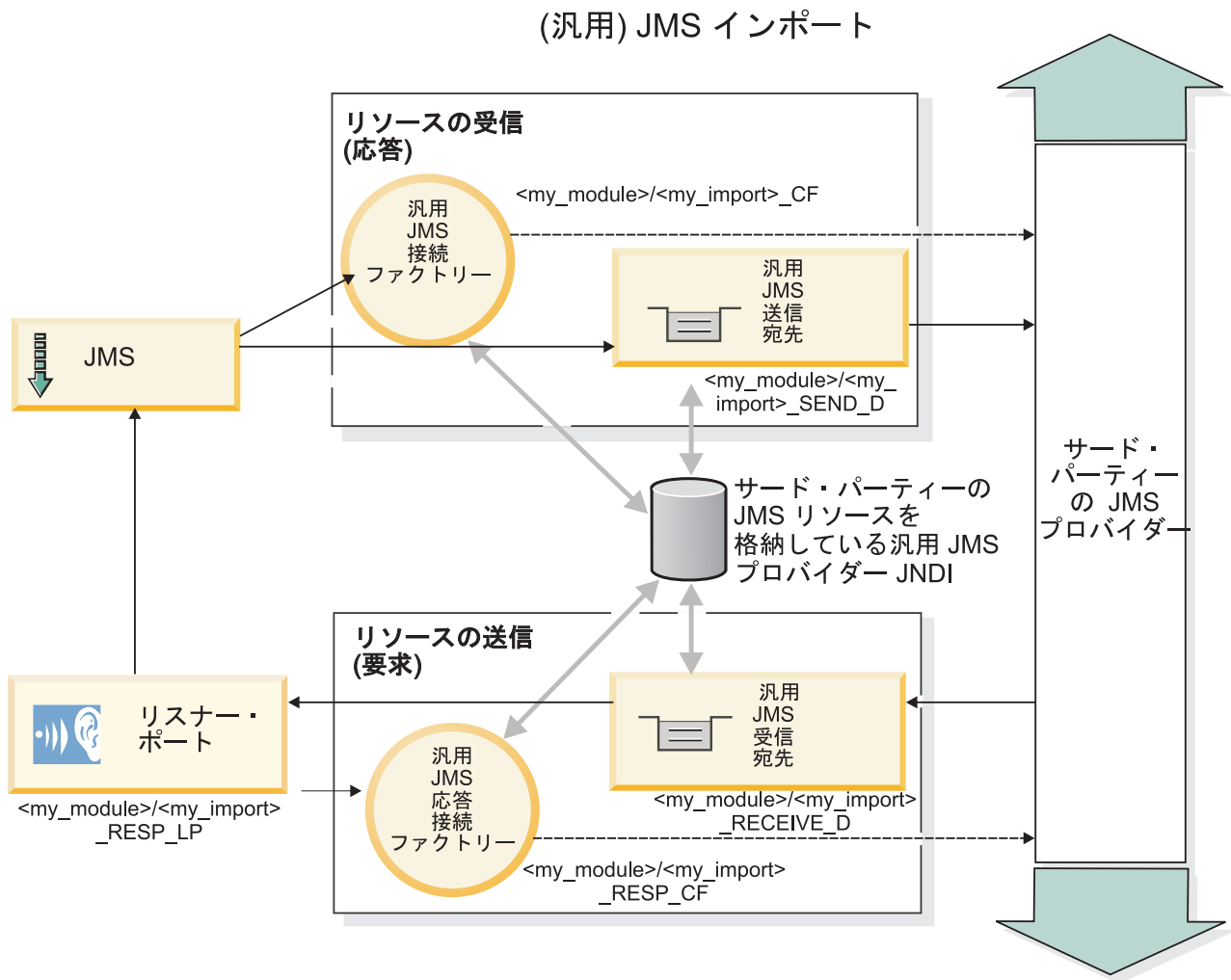
図 35. 汎用 JMS インポート・バインディング・リソース
