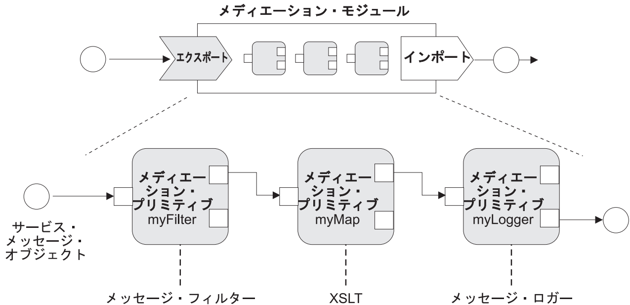
図 45. 3 つのメディエーション・プリミティブから成るメディエーション・モジュール
