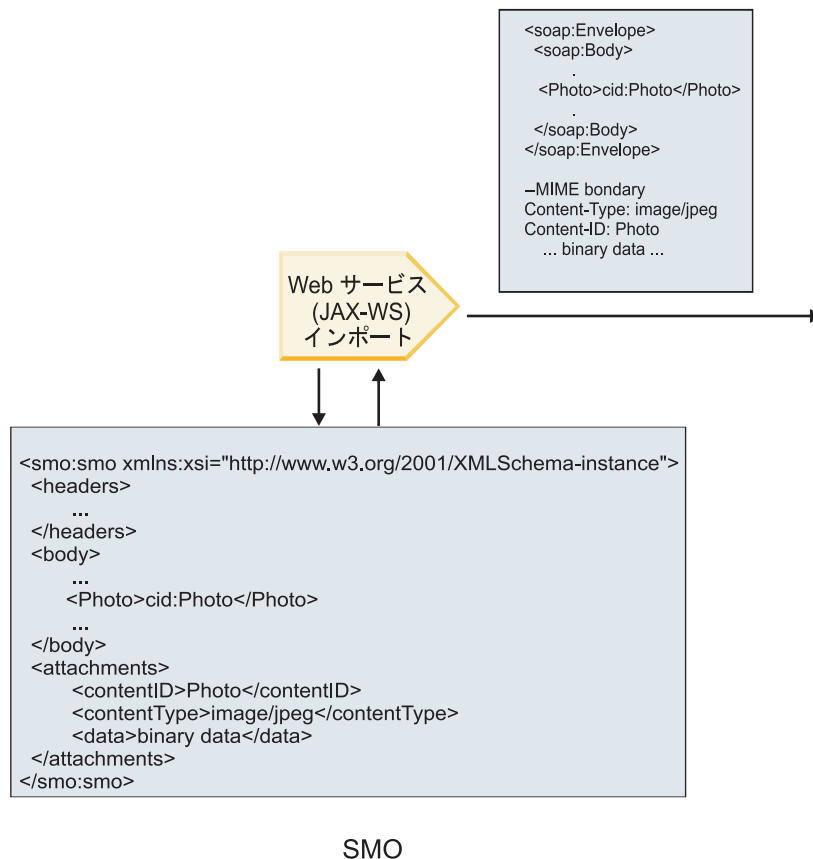
図 63. SOAP メッセージを作成するために SMO 内の swaRef 添付ファイルがアクセスされる方法
