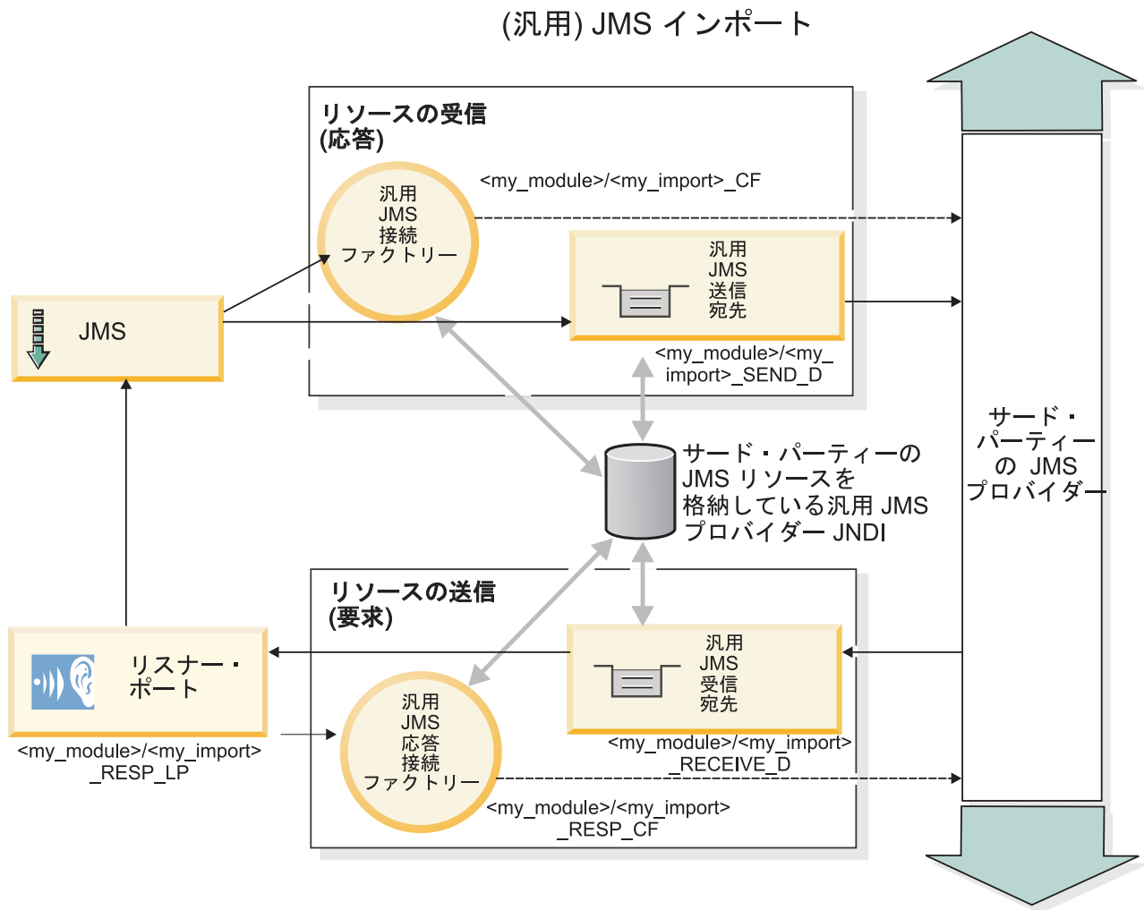
図 80. 汎用 JMS インポート・バインディング・リソース
