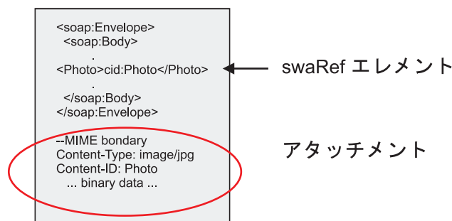
図 59. swaRef エレメントが含まれている SOAP メッセージ
