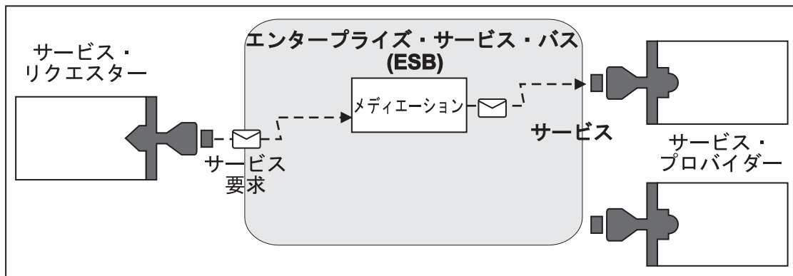
図 87. エンタープライズ・サービス・バス： エンタープライズ・サービス・バスは、サービスのリクエスターまたはプロバイダーであるアプリケーション間で、メッセージをルーティングしています。このバスはトランスポート・プロトコルを変換し、リクエスターとプロバイダーの間でメッセージ・フォーマットを変換しています。この図では、それぞれのアプリケーションは、(コネクタの異なる形状で表されている) 異なるプロトコルを使用し、異なるメッセージ・フォーマットを使用します。
