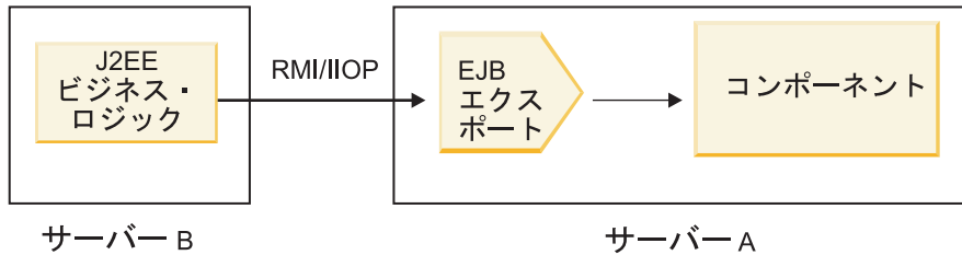
図 75. EJB エクスポートによるクライアントから SCA コンポーネントに対するリモート呼び出し
