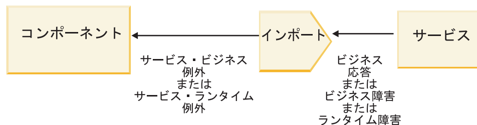
図 55. 障害情報をインポートを経由してサービスからコンポーネントに送信する方法
