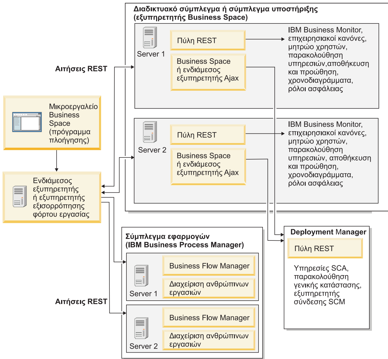
Σχήμα 1. Τυπική τοπολογία
