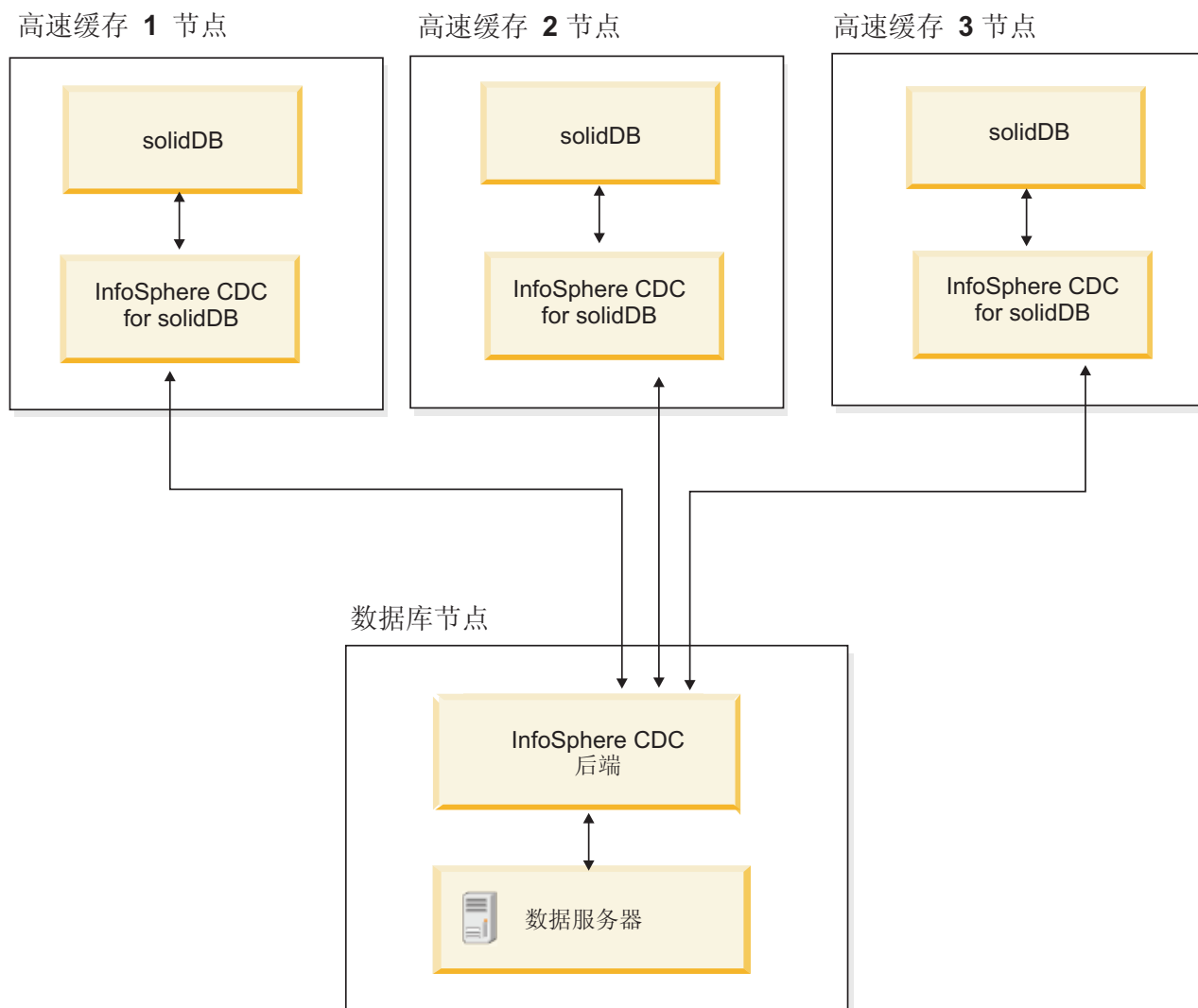
图 4. 使用多个 solidDB 服务器进行 Universal Cache 部署
