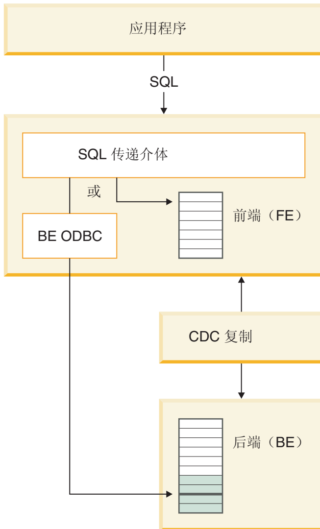
图 8. SQL 传递
