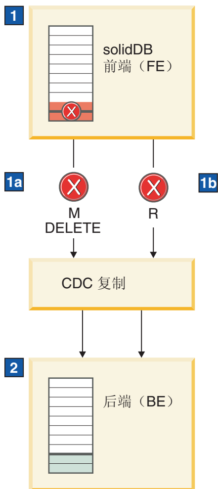
图 10. 数据帐龄体系结构
