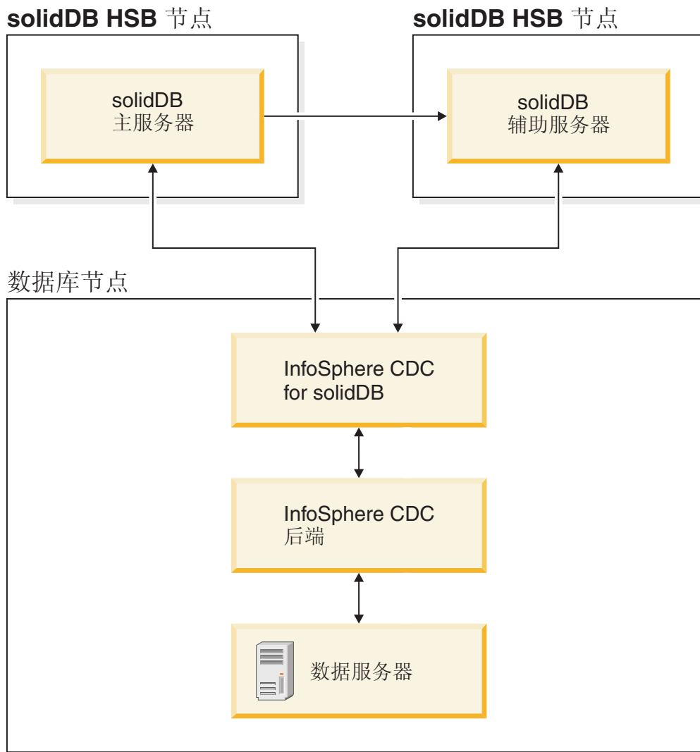
图 5. 示例: 具有 solidDB 高可用性的 Universal Cache
