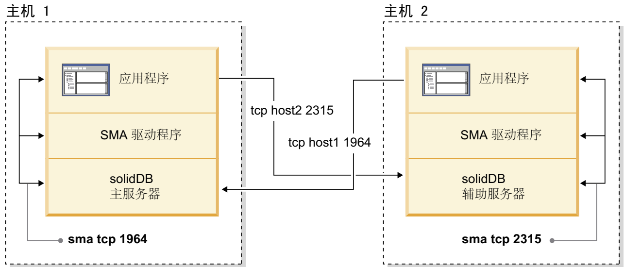
图 4. 示例: HotStandby 与 SMA 配置
