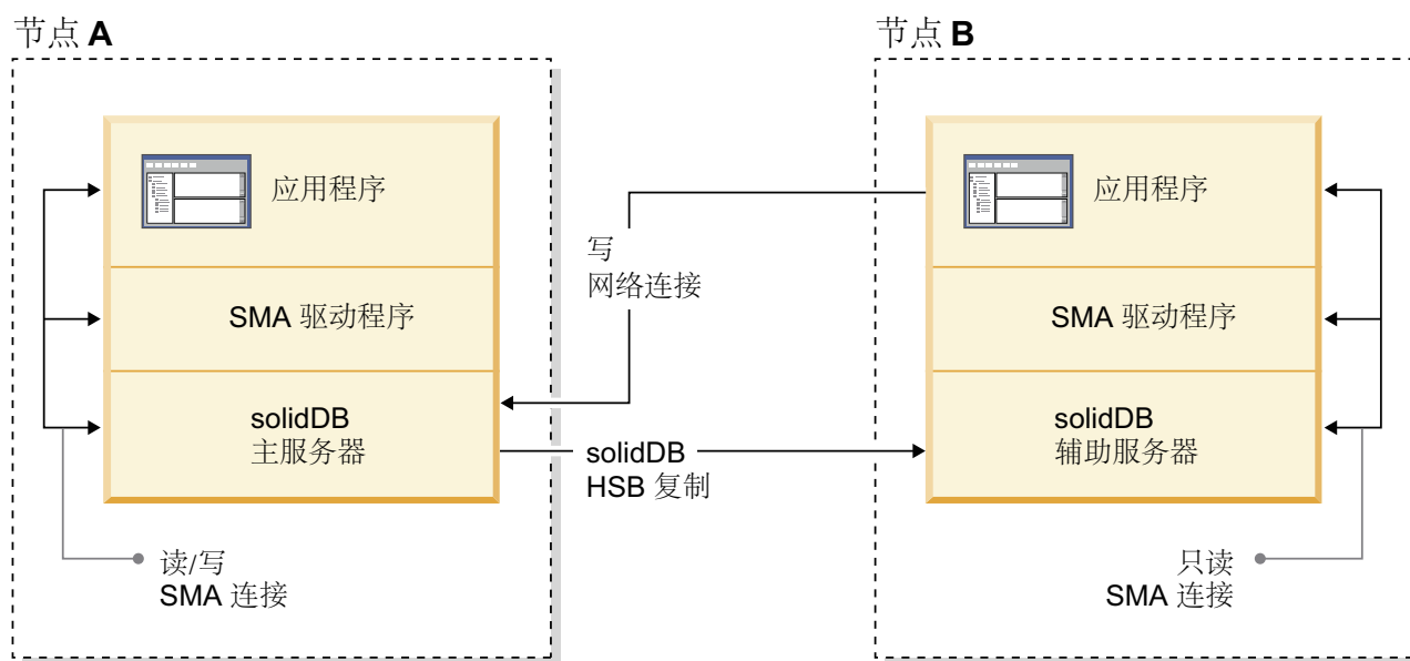
图 3. SMA 透明连接与 HotStandby 的体系结构
