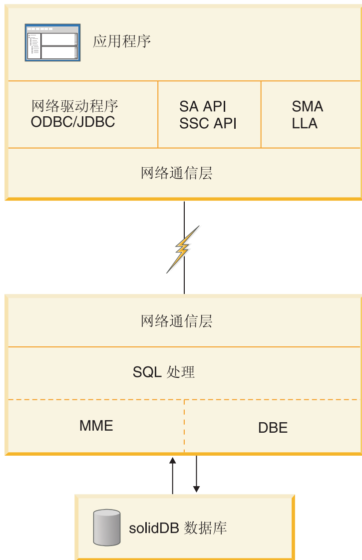
图 3. solidDB 组件
