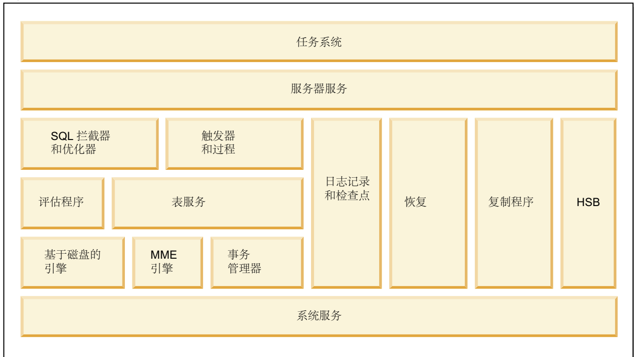
图 7. solidDB 组件
