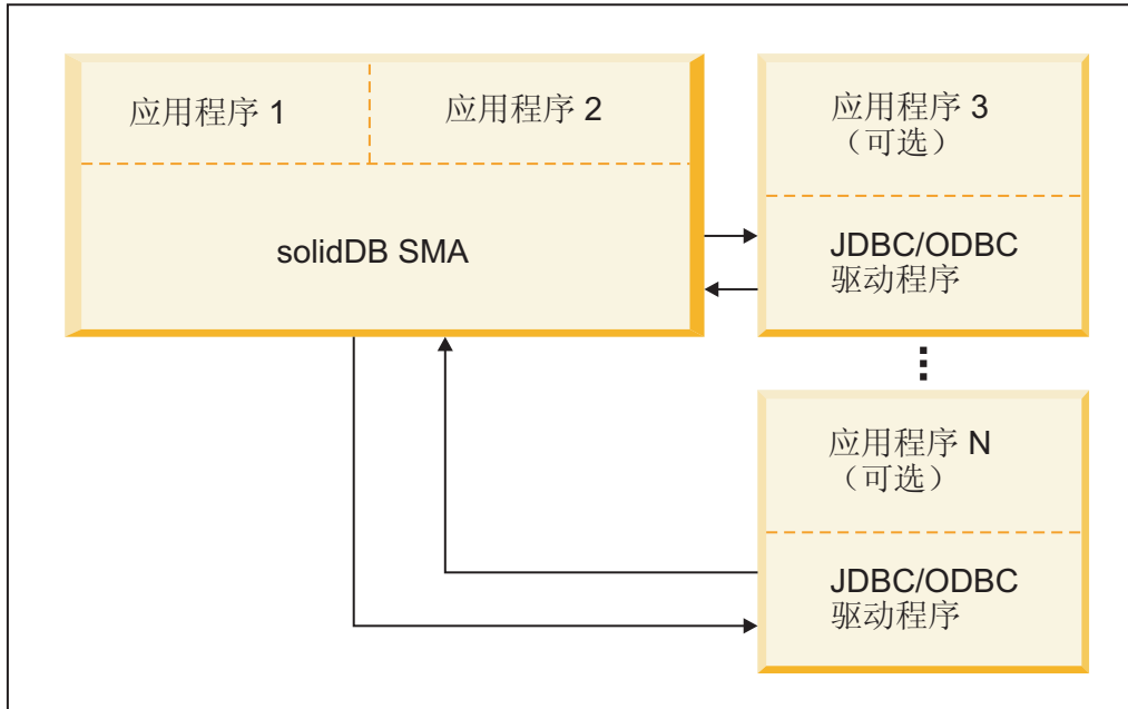
图 5. SMA 和 LLA 访问方法
