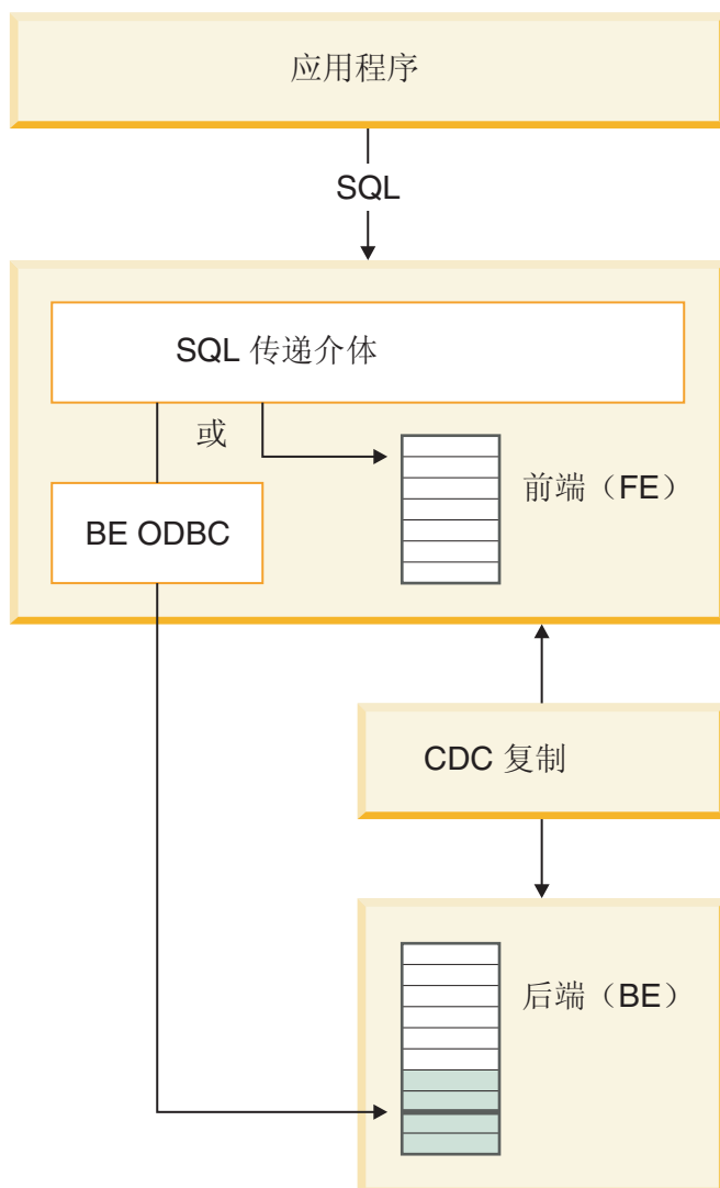
图 6. SQL 传递
