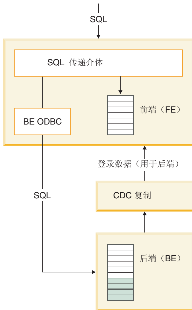
图 7. SQL 传递体系结构
