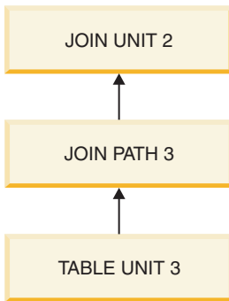
图 4. 执行图 1
