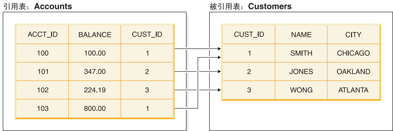
图 2. 引用约束
