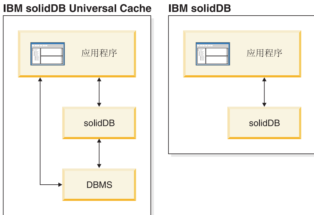
图 1. solidDB 6.5 产品
