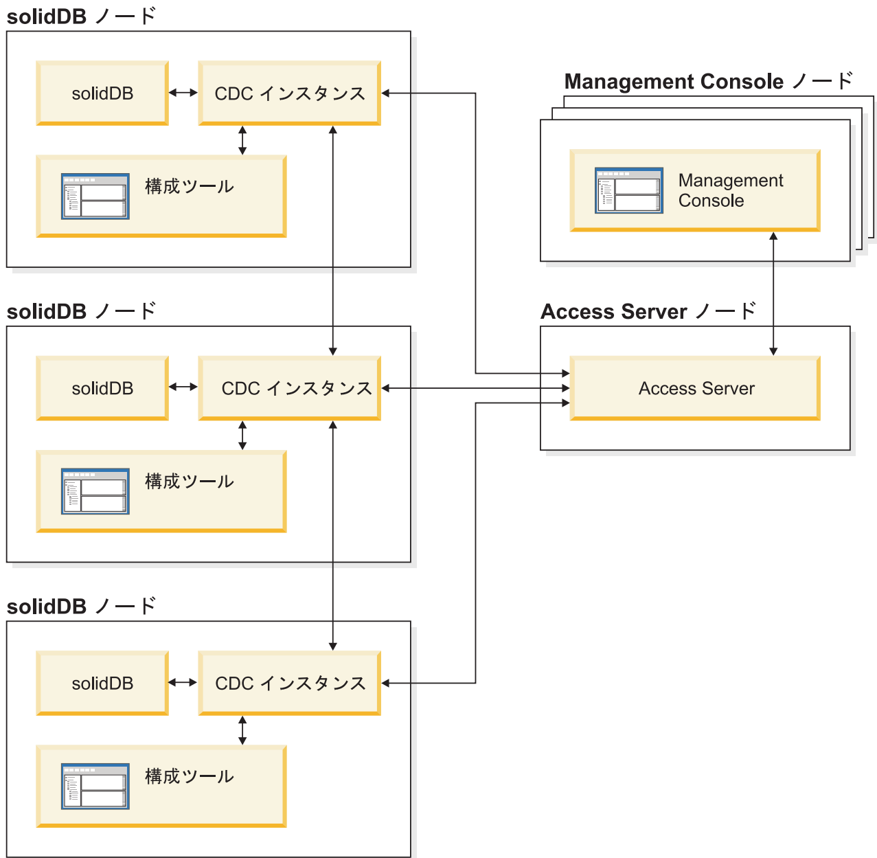
図1. CDC レプリケーションのアーキテクチャー
