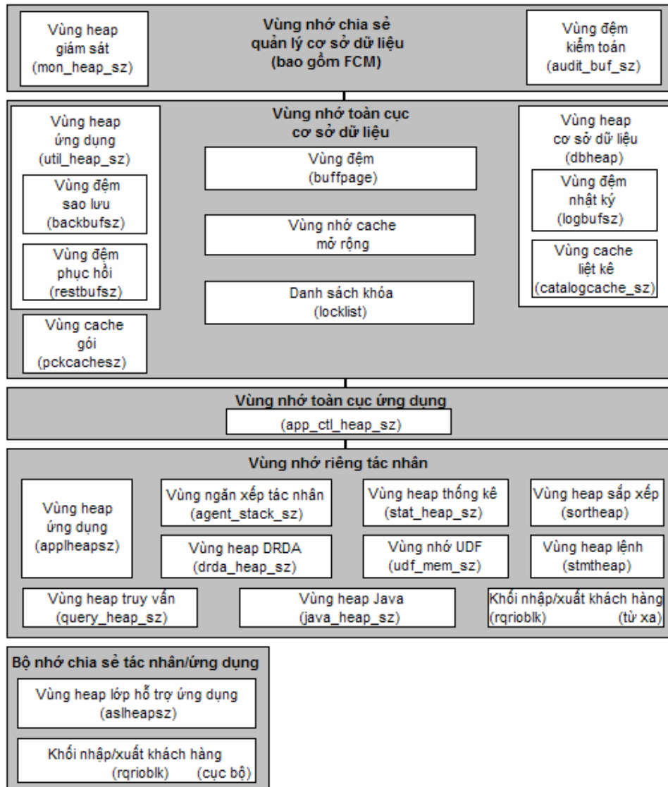
Hình 6.2 – Mô hình bộ nhớ của DB2
