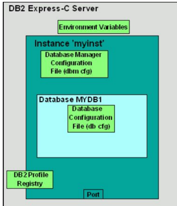
Hình 4.12 – Cấu hình DB2
