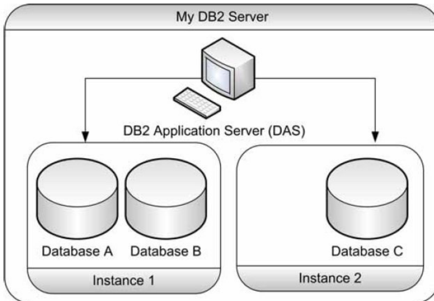
Hình 4.16 – Máy chủ quản trị DB2 (DAS).
