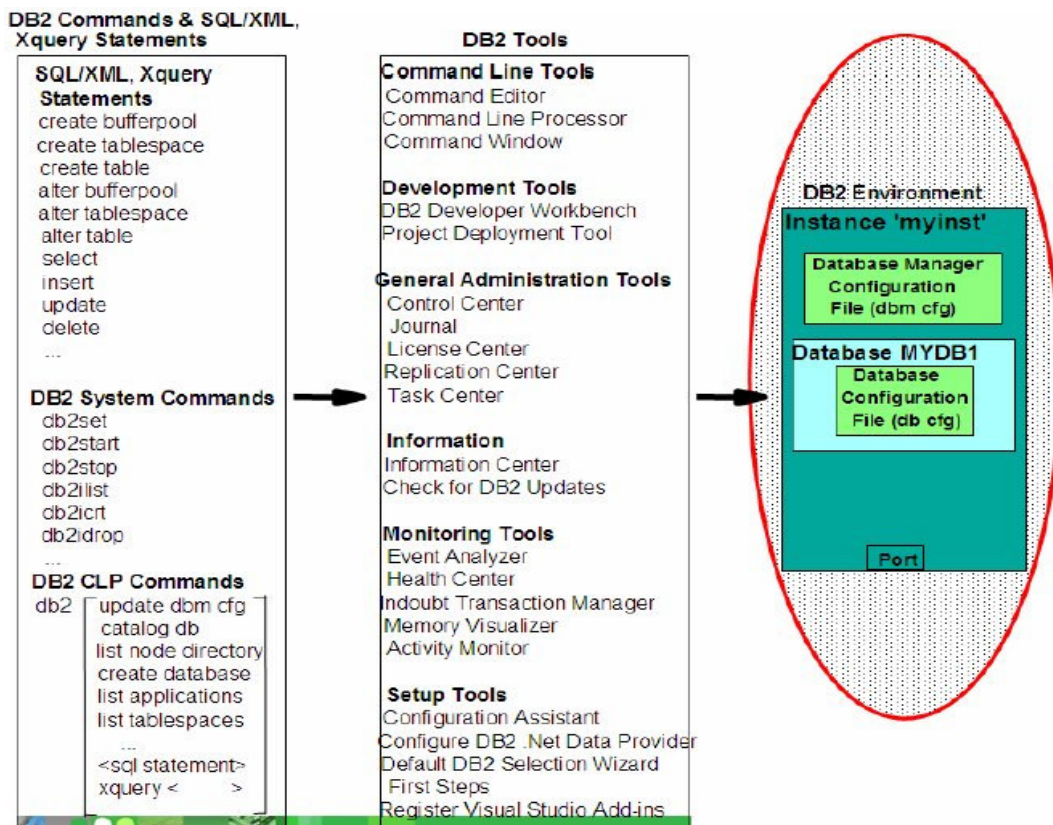
Hình 4.1 - Bức tranh tổng thể về DB2: Môi trường DB2
