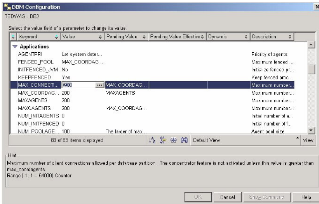
Hình 4.14 – Danh sách dbm cfg.
