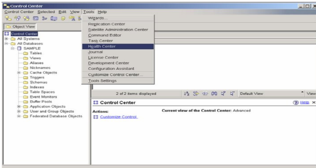
Hình 5.20 – Khởi chạy Trung tâm sức khỏe
