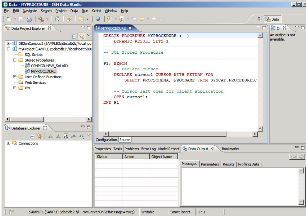
Hình 14.5 – Một thủ tục mẫu
