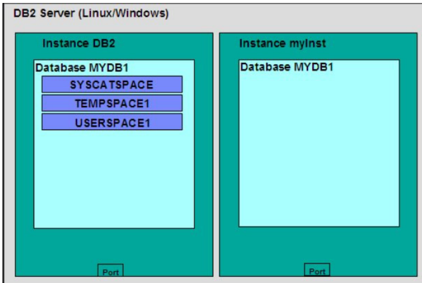
Hình 4.8 – Không gian bảng được tạo mặc định khi một CSDL được tạo ra.
