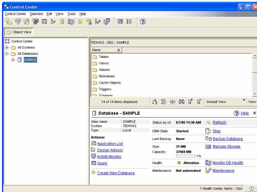
Hình 12.4 – Hiện thị thông số cơ sở dữ liệu từ Trung tâm điều khiển
