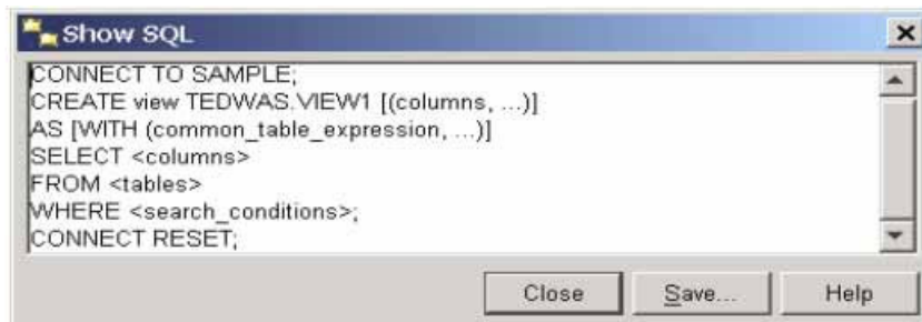
Hình 5.14 – Đầu ra của một phần trình bày về nút “Show SQL”
