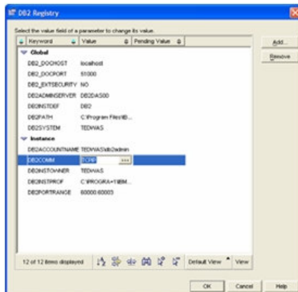
Hình 7.3 – Kiểm chứng giá trị của biến DB2COMM trong thư mục DB2
