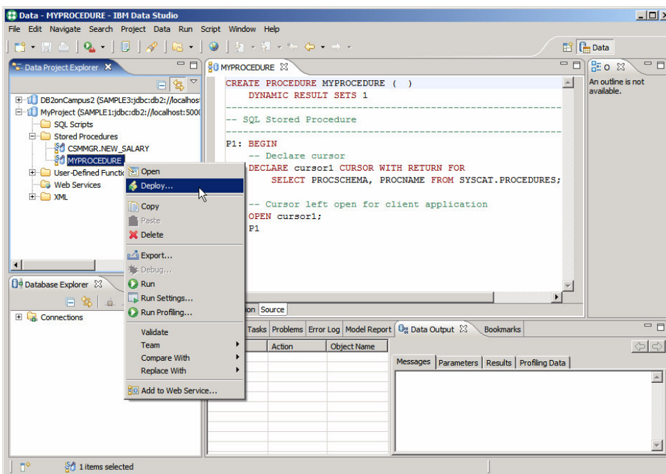
Hình 14.6 – Triển khai một thủ tục
