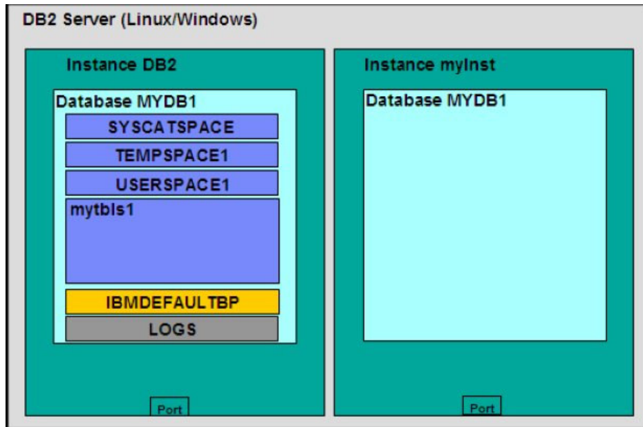
Hình 4.9 – Vùng đệm dữ liệu và các tệp nhật ký.
