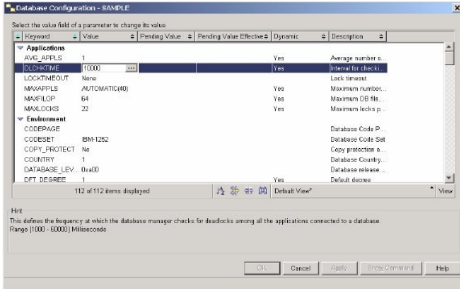
Hình 4.16 – Cấu hình cơ sở dữ liệu db cfg.
