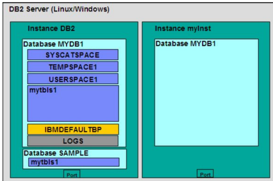
Hình 4.10 – Không gian bảng có cùng tên trong các cơ sở dữ liệu khác nhau.
