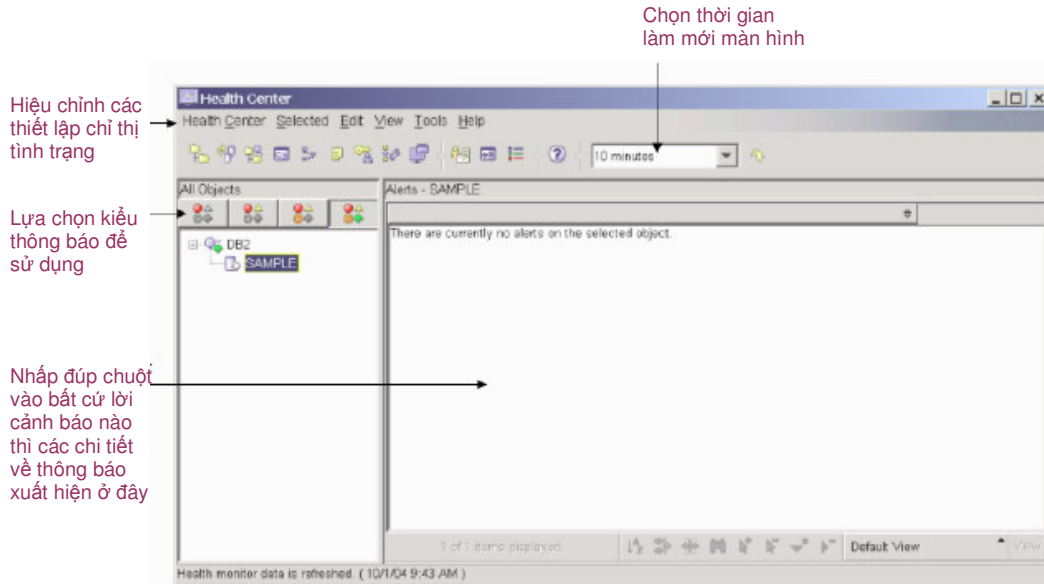
Hình 5.19 – Công cụ Trung tâm tình trạng
