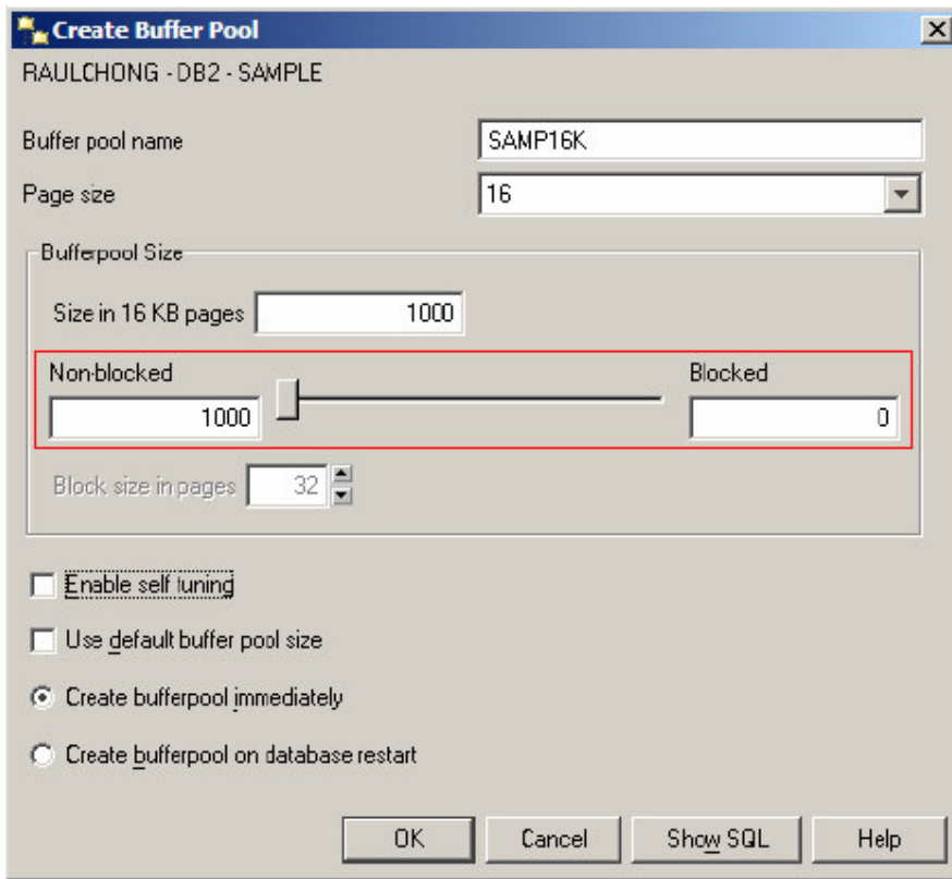
Hình 6.4 - Hộp thoại tạo vùng nhớ đệm
