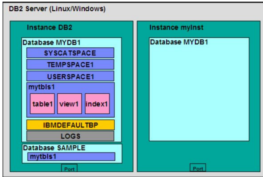
Hình 4.11 – Bảng, khung nhìn và chỉ mục được tạo trong vùng bảng.
