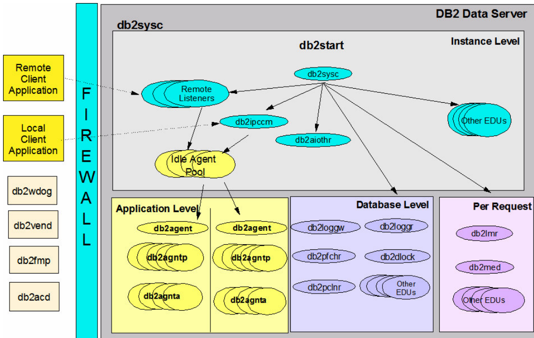
Hình 6.1 – Mô hình quy trình xử lý của DB2
