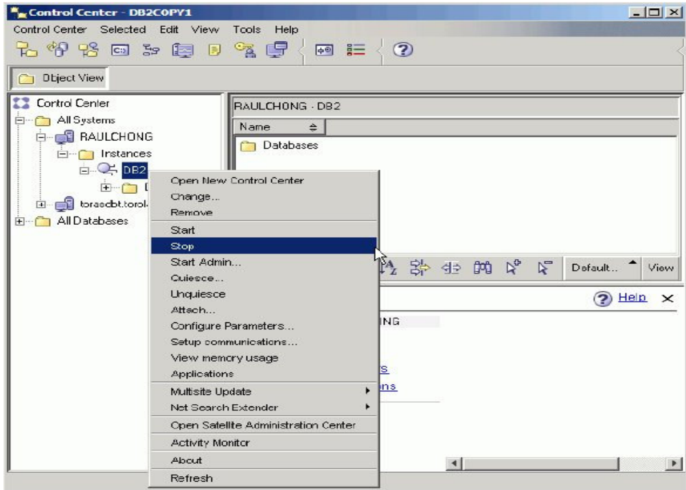
Hình 4.5 – Các lệnh trên thẻ hiện trong cửa sổ Control Center
