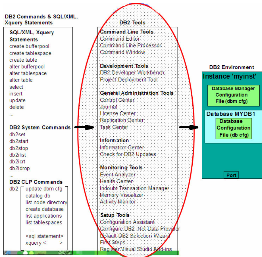
Hình 5.1 - Bức tranh tổng thể DB2: Công cụ của DB2
