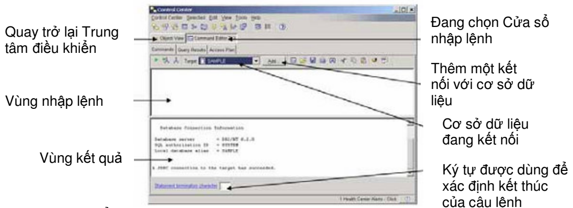
Hình 5.7 - Cửa sổ nhập lệnh của DB2
