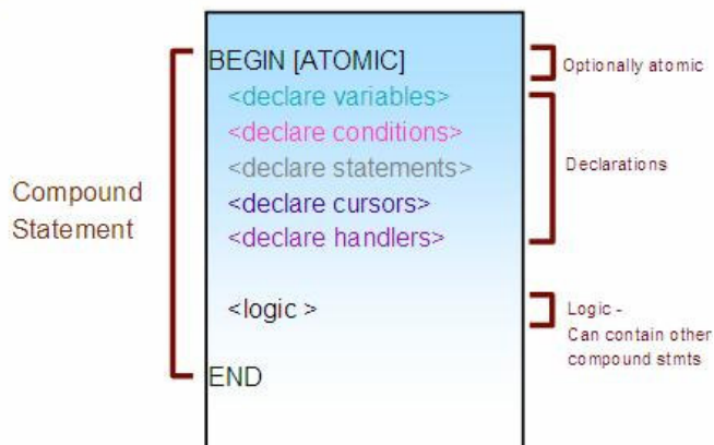
Hình 14.7 – Câu lệnh ghép
