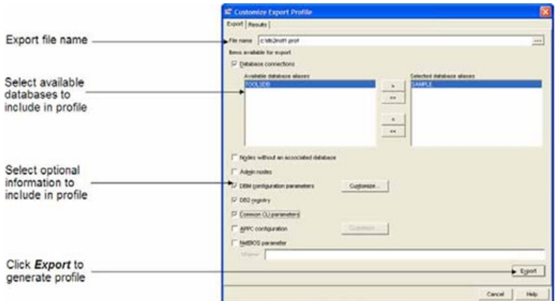
Hình 7.11 – Hộp thoại tùy chỉnh xuất lý lịch
