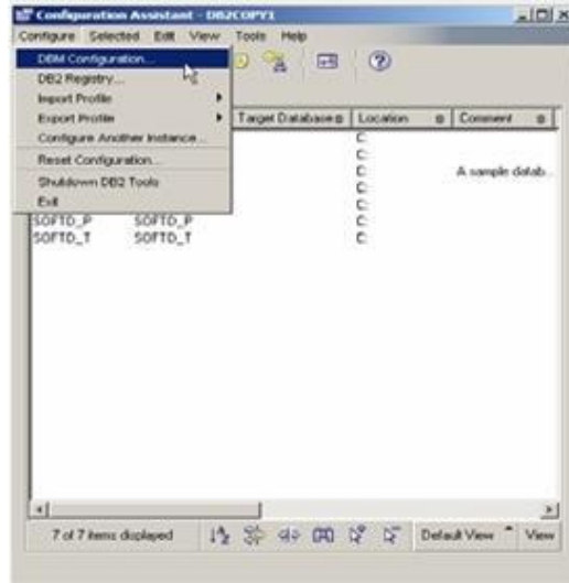
Hình 7.4 – Xem xét dbm cfg từ Trợ giúp cấu hình
