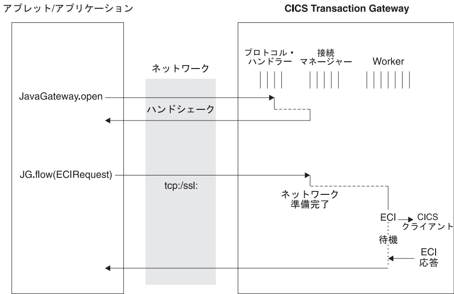
図2. CICS Transaction Gateway スレッド化モデル (TCP/IP および SSL 用). これらのプロトコルは、永続ソケットを持っています。
