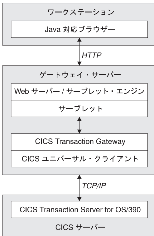
図 8. URL によって起動される端末サーブレットを使用する CICS Transaction Gateway
