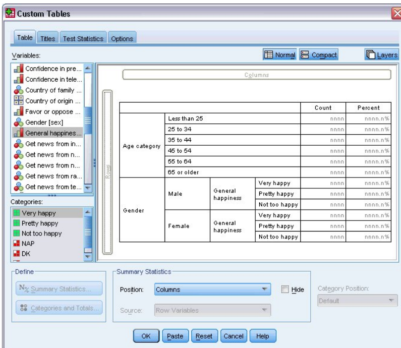
그림 1. 사용자 정의 표 대화 상자, 테이블 탭
