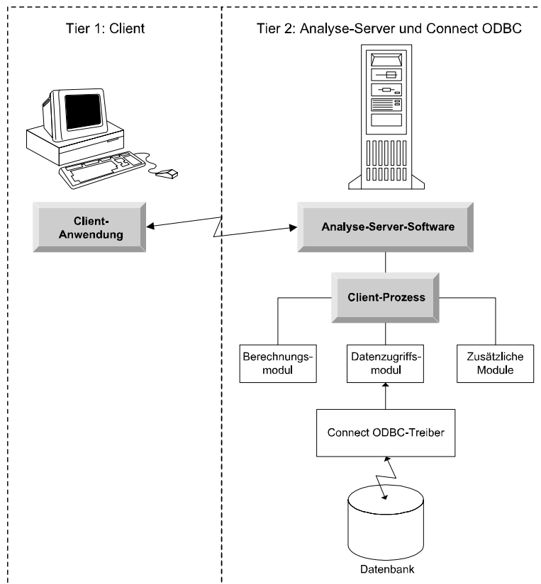
Abbildung 1-1 Connect ODBC im verteilten Analysemodus
