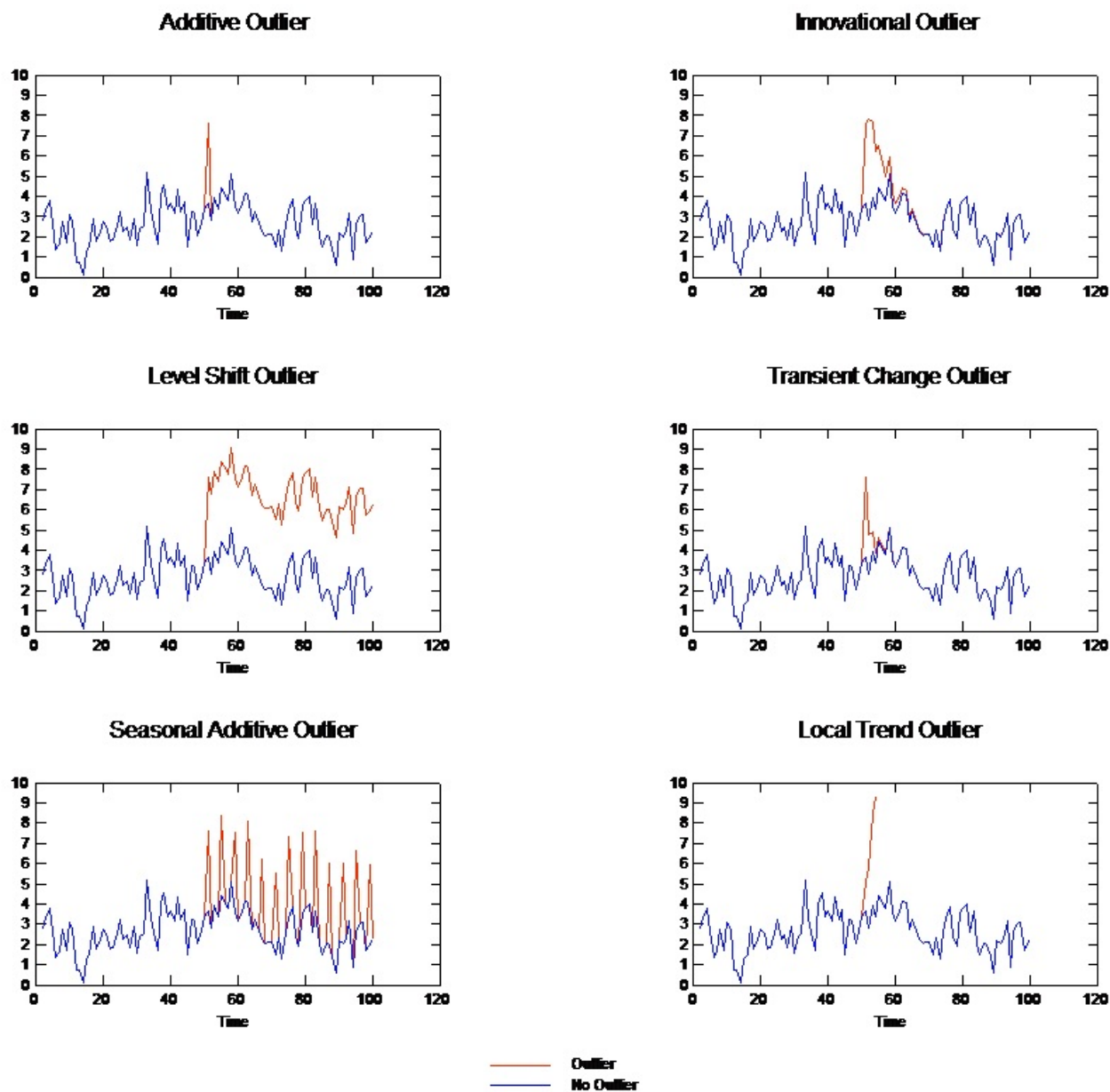
圖 57. 離群值類型
