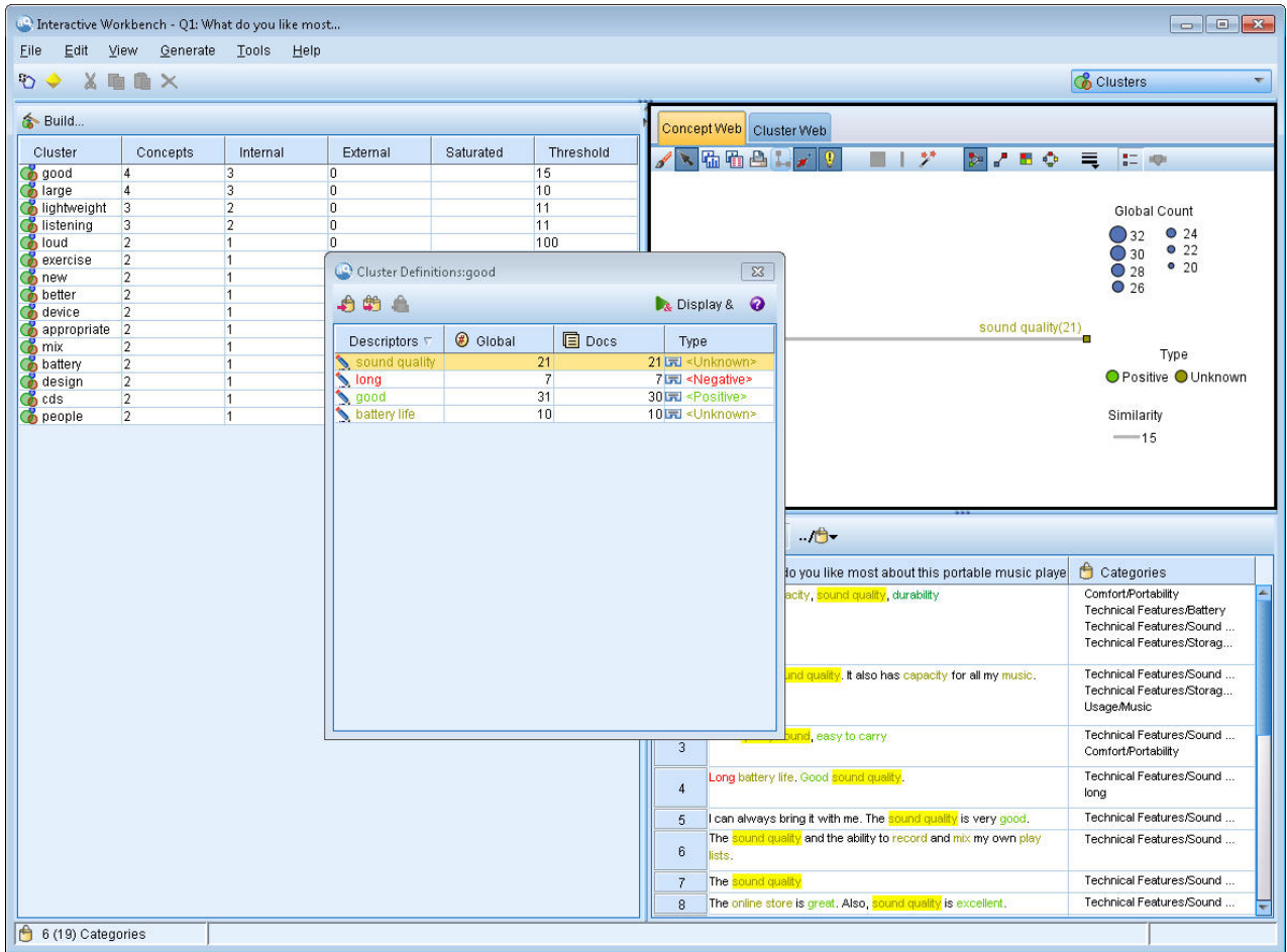
图 24. “聚类”视图
