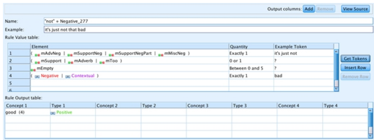
Рисунок 35. TLA rules
