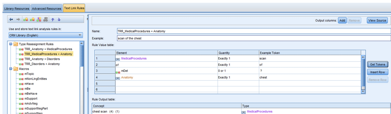
Rysunek 37. Reguła TRR dla: zabiegi medyczne + część ciała
