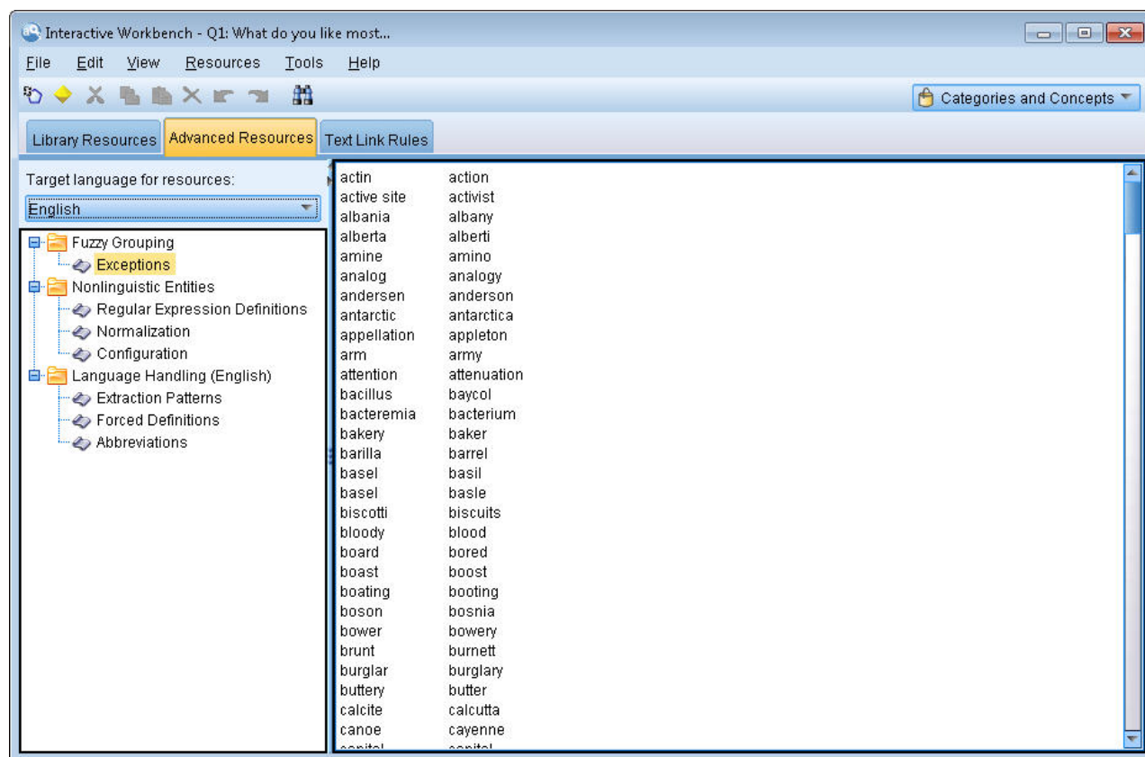
Rysunek 43. Edytor szablonów eksploracji tekstu - karta Advanced Resources
