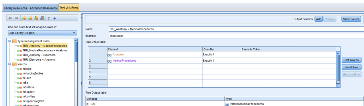
Rysunek 36. Reguła TRR dla: część ciała + zabiegi medyczne
