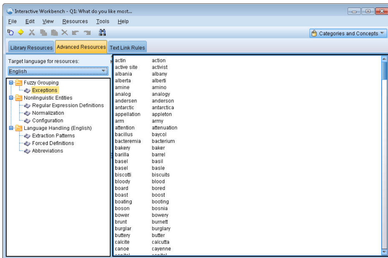
Rysunek 40. Edytor szablonów eksploracji tekstu - karta Advanced Resources
