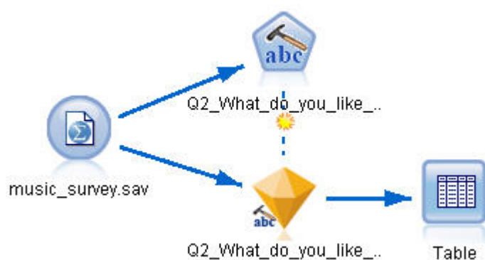
Rysunek 3. Przykładowy strumień: węzeł Plik Statistics z modelem użytkowym Text Mining
