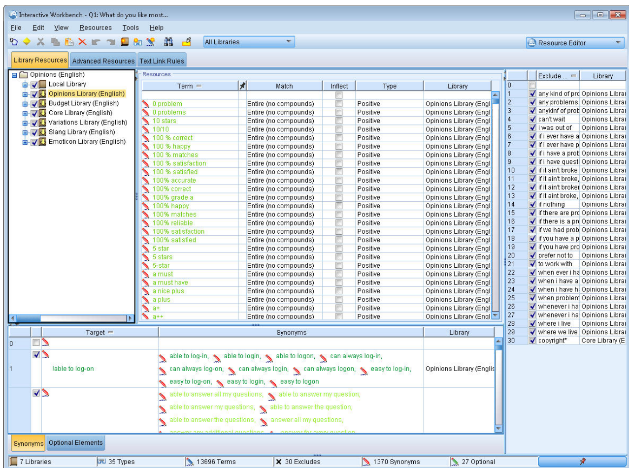
Rysunek 38. Widok Resource Editor
