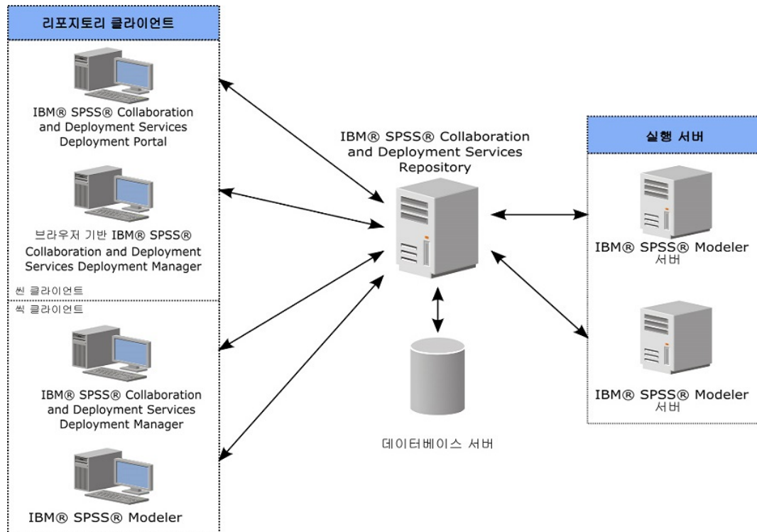
그림 1. IBM SPSS Collaboration and Deployment Services 아키텍처
