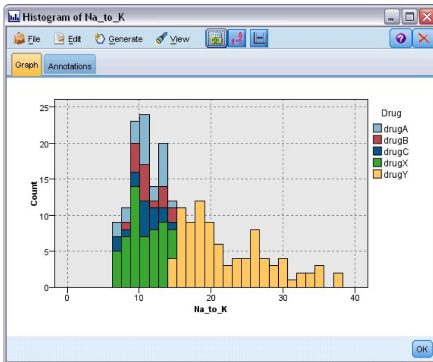
그림 2. 표본 히스토그램
