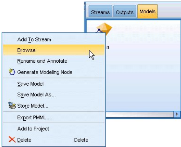
그림 96. 모델 찾아보기
