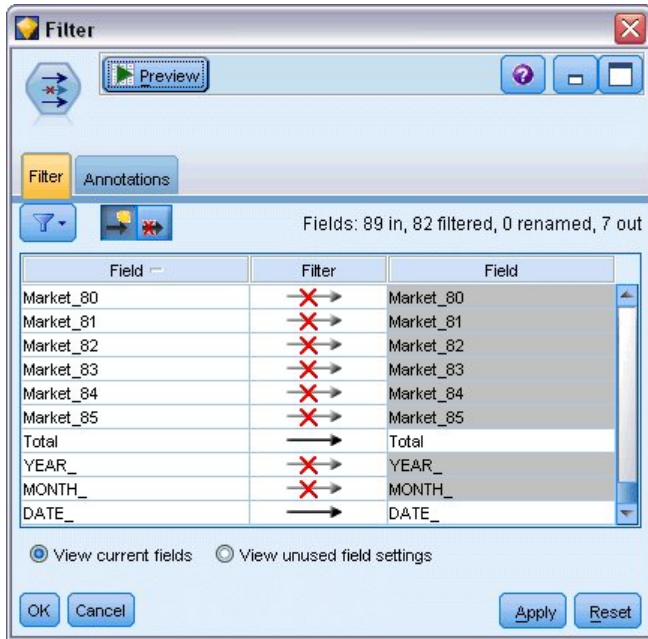
그림 172. 모델 단순화
