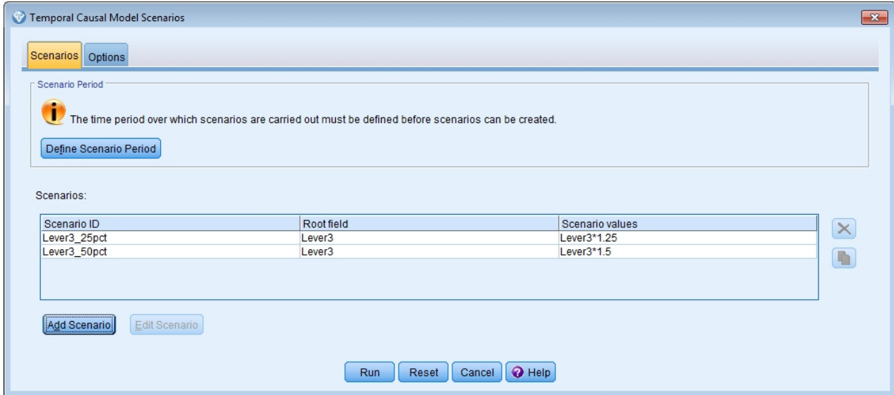
그림 411. 시나리오
