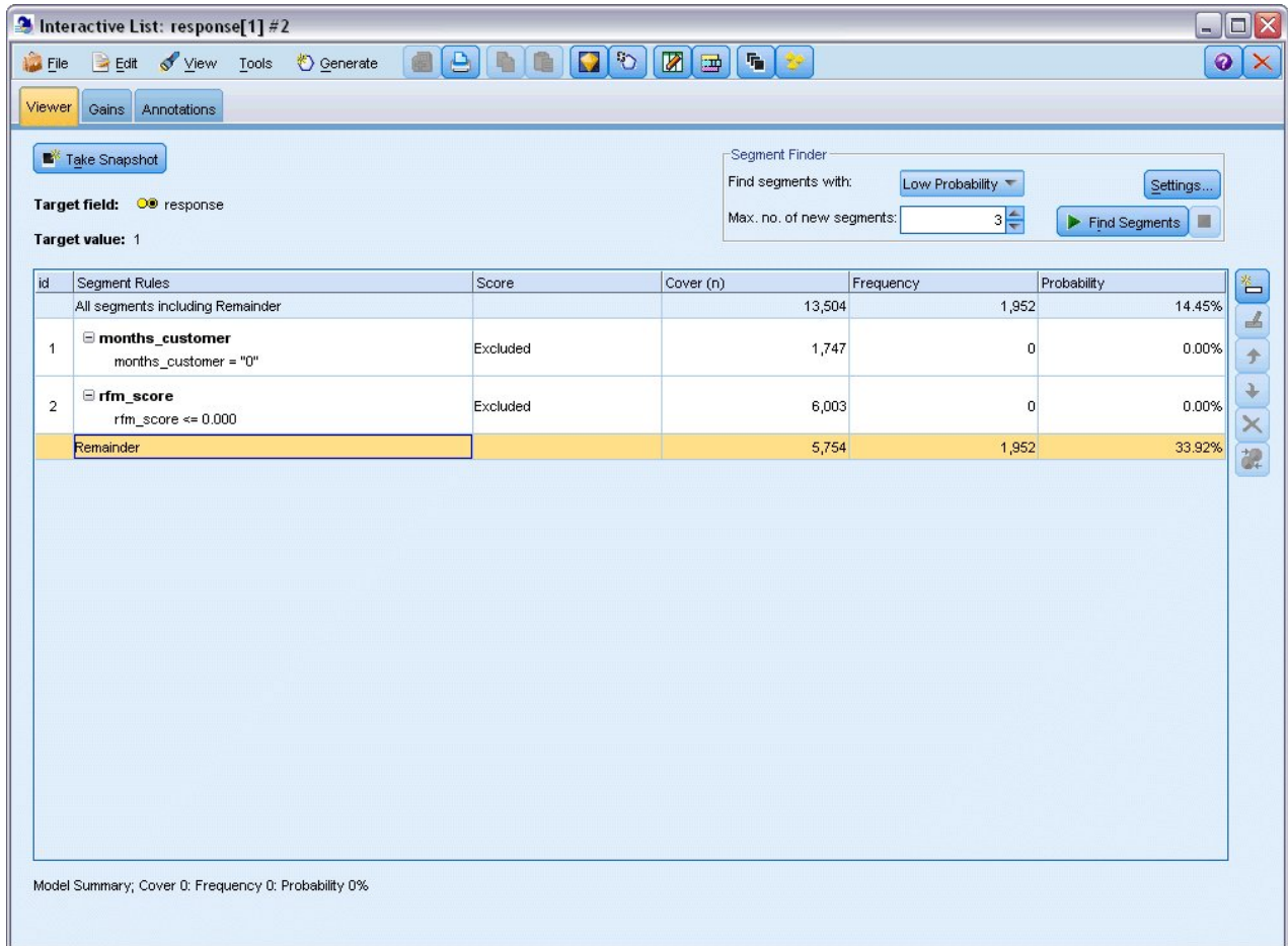
그림 131. 세그먼트 선택
