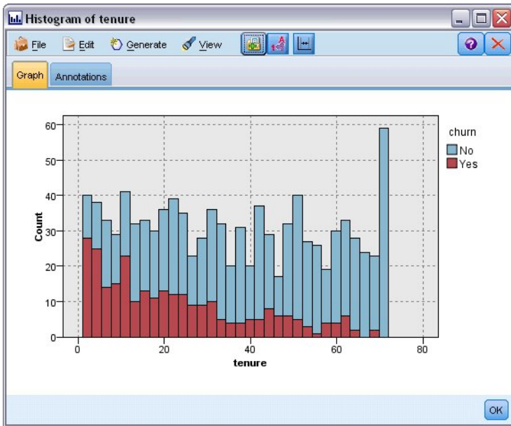
그림 67. 재직 히스토그램
