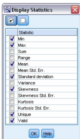
그림 66. 통계 표시
