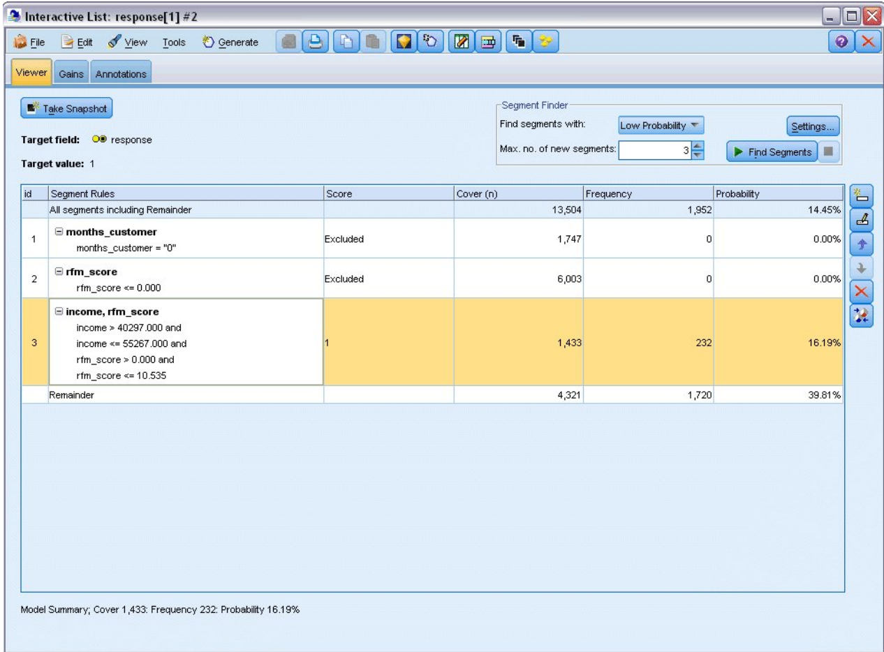
그림 130. 세그먼트 제외
