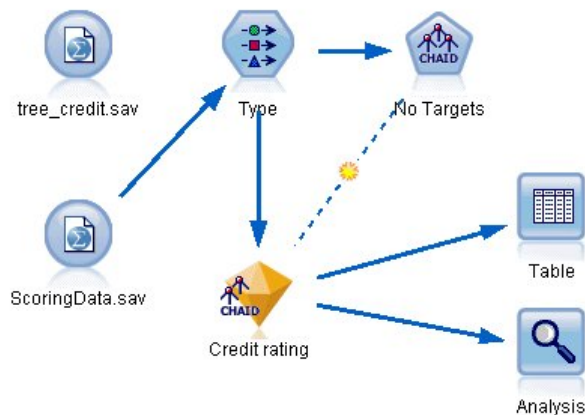
Figure 18. Association de nouvelles données pour le scoring
