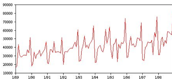
Figure 54. Cycle saisonnier
