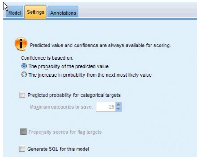
Figure 43. Onglet Paramètres
